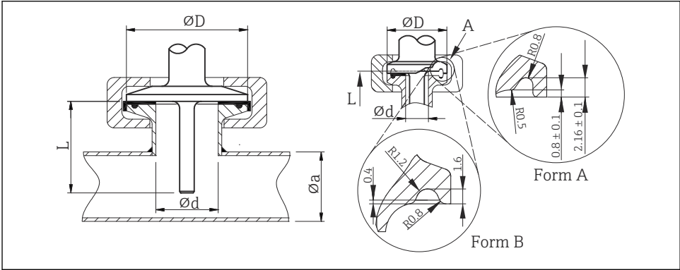
12 Зажим в соответствии с ISO 2852
