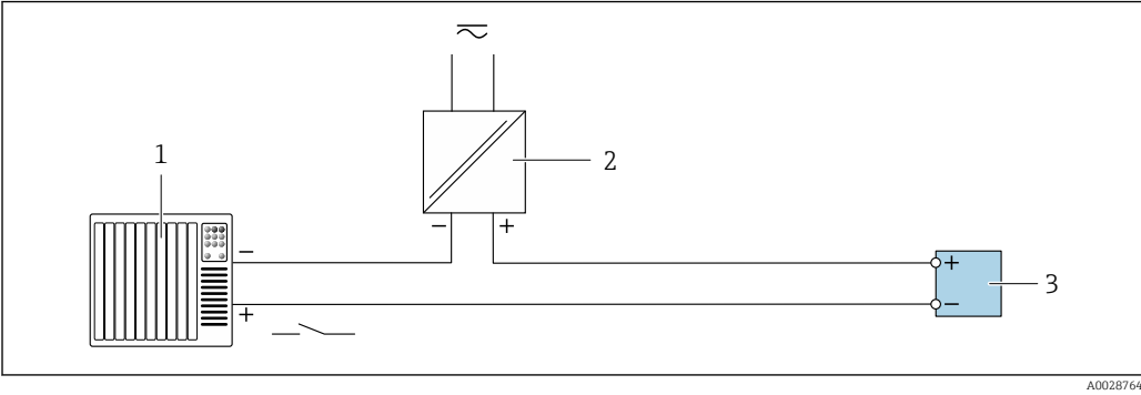
29 Exemple de raccordement pour l'entrée état 1 Système/automate avec sortie état (p. ex. API) 2 Alimentation électrique 3 Transmetteur
