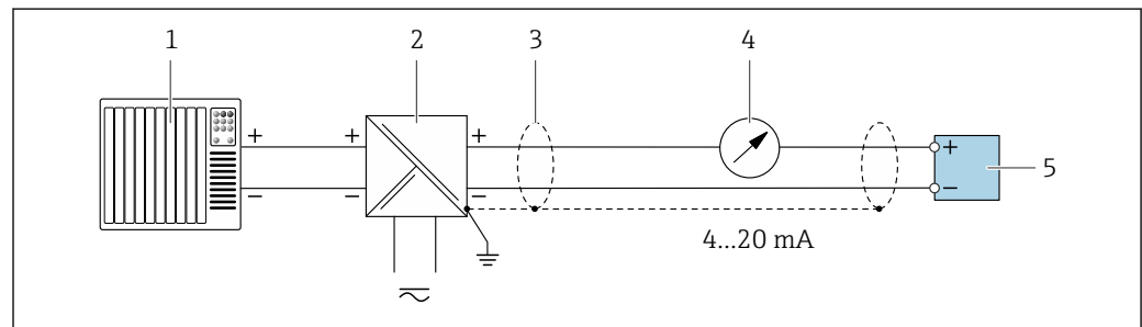
19 Exemple de raccordement pour sortie courant 4 à 20 mA HART (passive)
