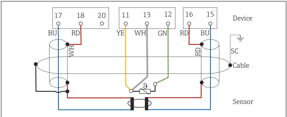
8 CLS50 к CM42B
