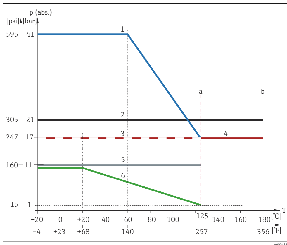
14 Кривые температуры/давления
