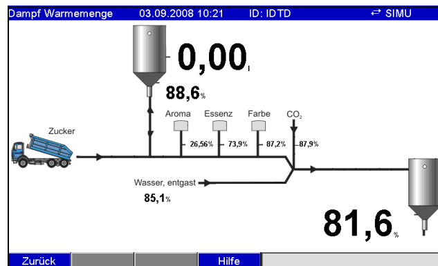
Abb. 97: Prozessbild
