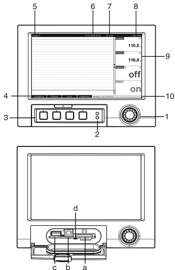
Abb. 12: Geräteanzeige / Bedieneinheiten
