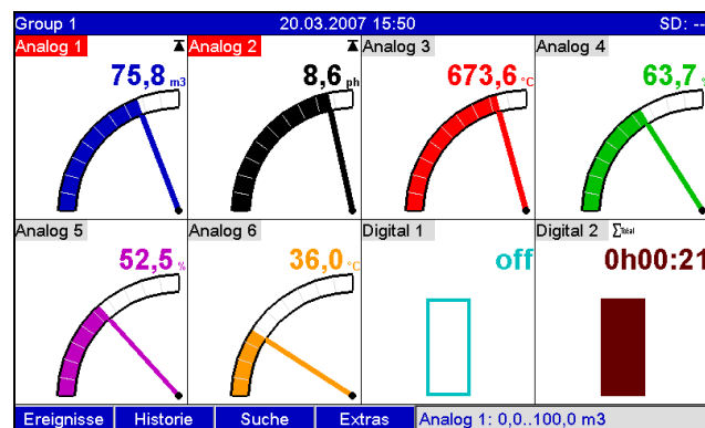
Abb. 95: Instrumentendarstellung
