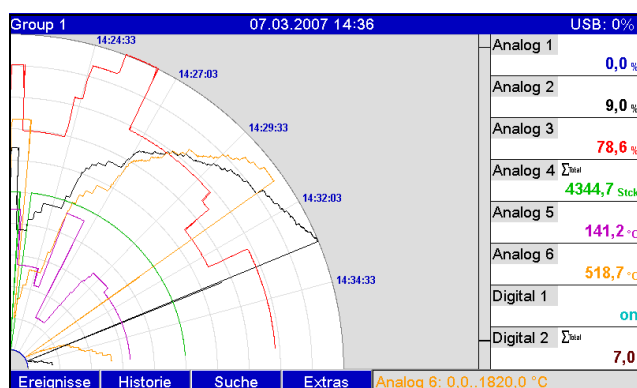
Abb. 92: Kreisblattdarstellung
