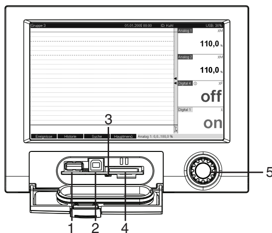
Abb. 85: Gerätefront mit geöffneter Klappe/Tastatur
