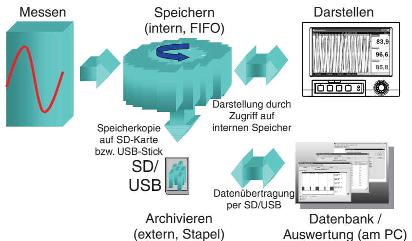
Abb. 80: Schematische Darstellung der Messwertspeicherung
