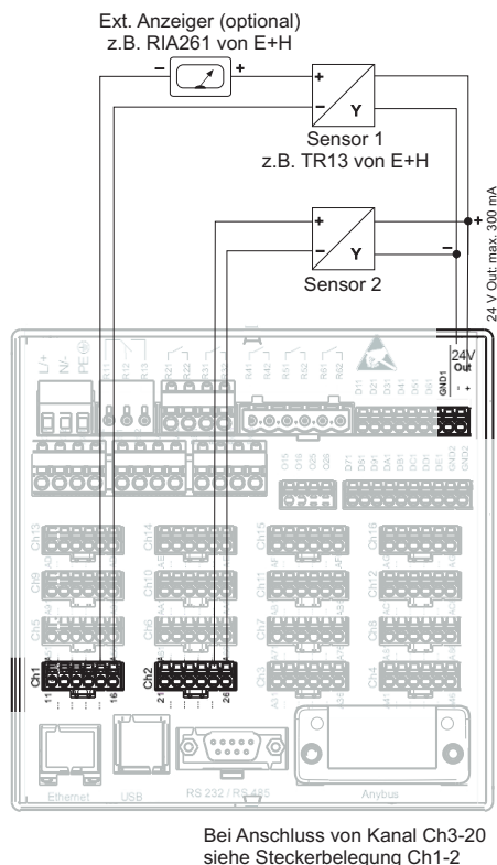
Abb. 6: Anschluss des Hilfsspannungsausgangs bei Verwendung als Messumformerspeisung (MUS) für 4-Leiter-Sensoren im Strommessbereich
