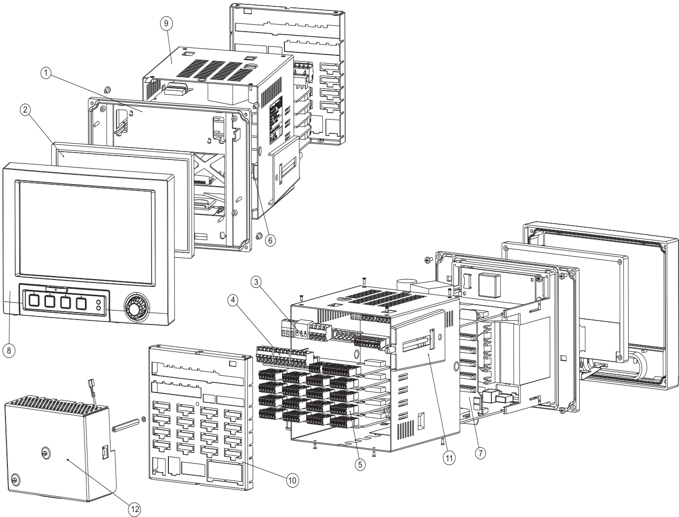
Abb. 84: Ersatzteildetail
