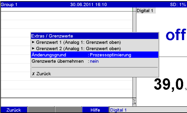
Abb. 73: Extras "Grenzwerte"
