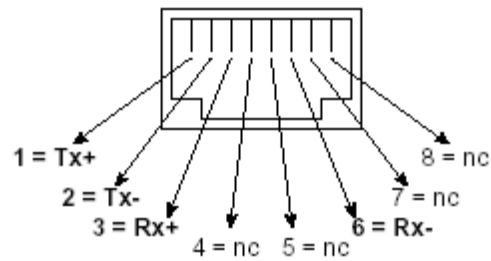
Abb. 10: RJ45-Buchse (Belegung AT&T25b)
