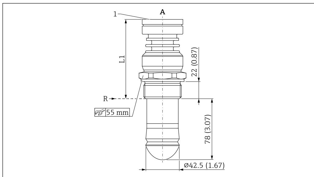
30 Размеры антенны с защитой от конденсата 50 мм (2 дюйм), резьбовое присоединение к процессу
