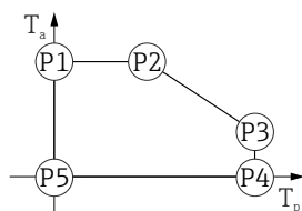
■ 12 Пластмассовый корпус; рабочая температура 0 до +130 °C ( +32 до +266 °F) для приборов с сертификатом CSA C/US
