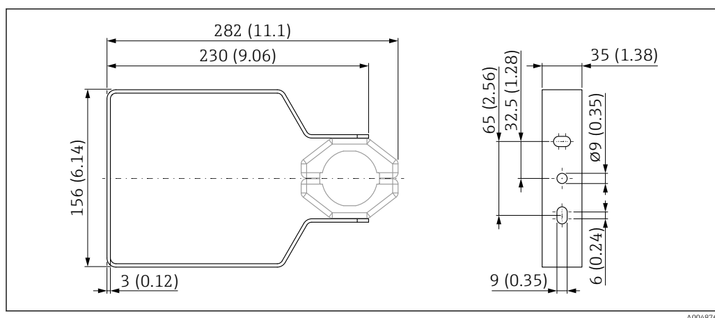
42 Размеры; регулируемый монтажный кронштейн FMR6xB. Единица измерения мм (дюйм)
