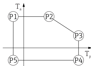
■ 18 Корпус 316L, гигиенический; рабочая температура -40 до +130 °C ( -40 до +266 °F)
