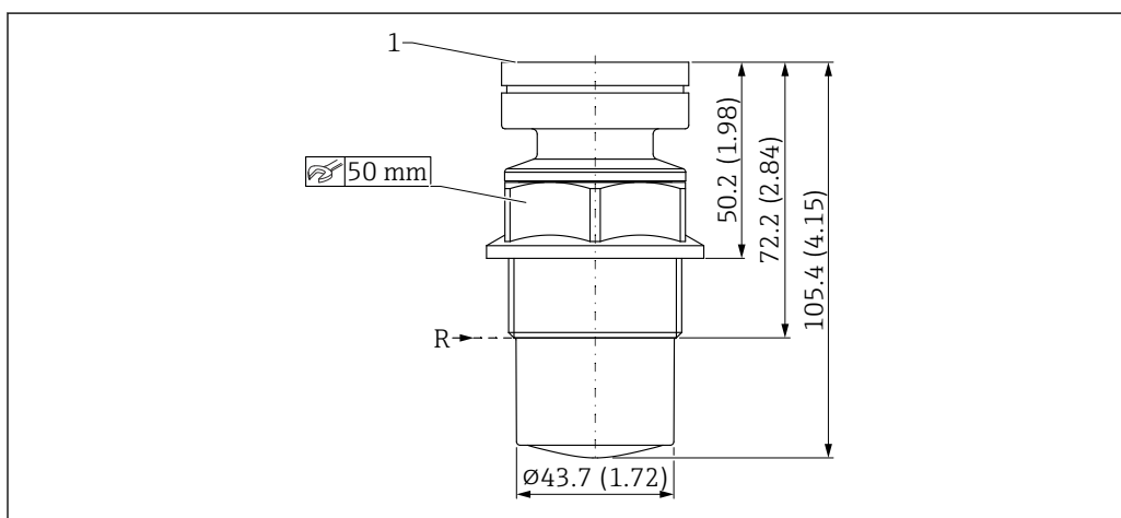
25 Размеры герметичной антенны, PVDF, 40 мм (1,5 дюйм). Единица измерения мм (дюйм)
