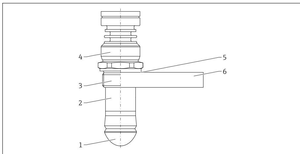
Антенна с защитой от конденсата 50 мм (2 дюйм)
