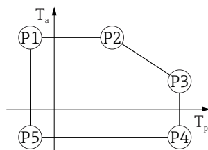
■ 17 Корпус 316L, гигиенический; рабочая температура -40 до +80 °C ( -40 до +176 °F)
