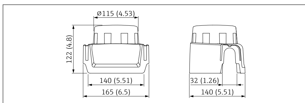
40 Размеры защитного козырька от погодных явлений, пластмасса, XW111. Единица измерения мм (дюйм)
