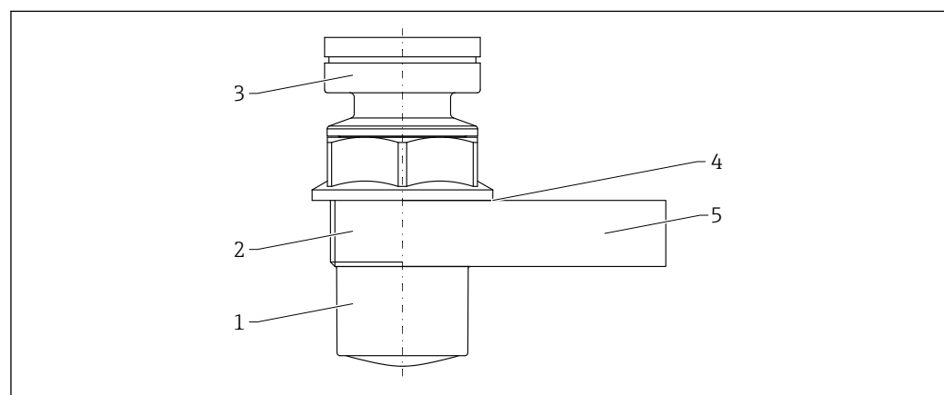
35 Материал; герметичная антенна из ПВХФ, 40 мм (1,5 дюйм)
