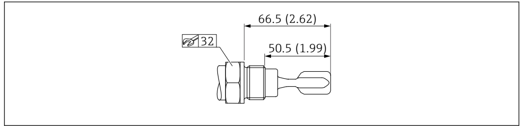
32 ISO228 G 3/4 螺纹。测量单位 mm (in)
