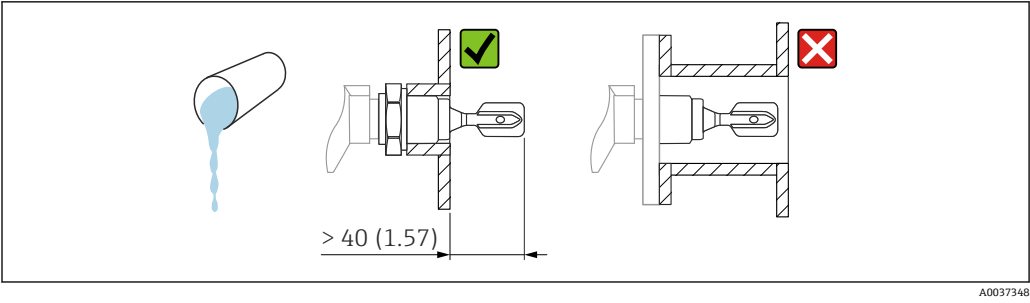
图 9 安装实例：测量高粘度液体。测量单位 mm (in)
