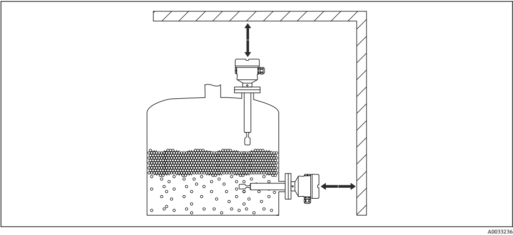
图 11 预留安装间隙
