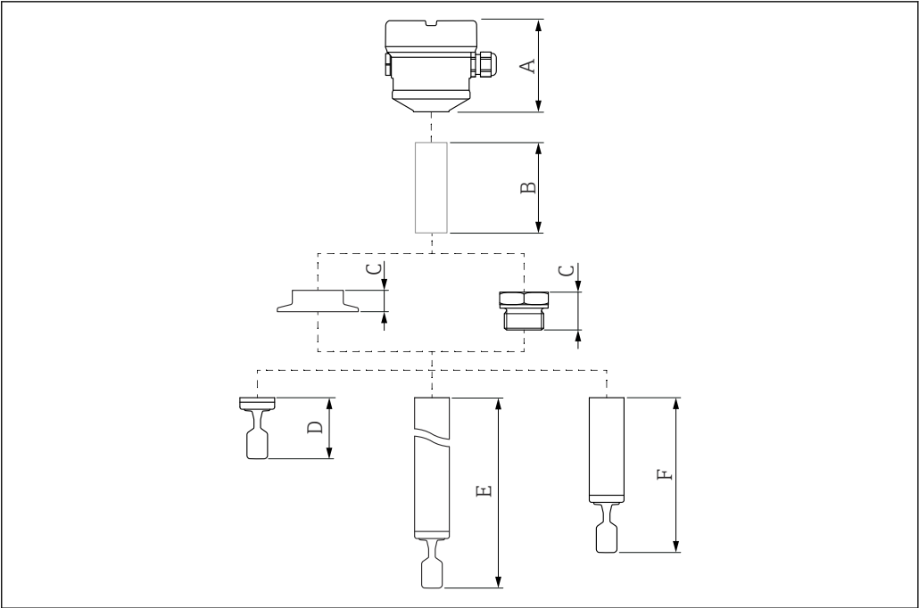
图 22 计算设备高度所需考虑的部件
