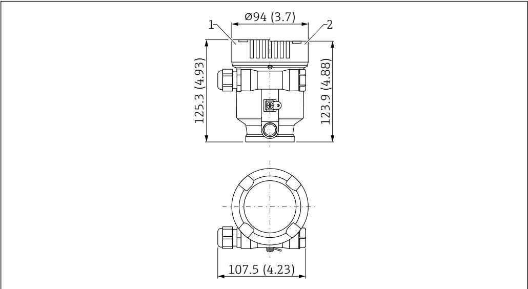
图 23 单腔室塑料外壳的外形尺寸示意图；包括 M20 接头和塑料插头。测量单位 mm (in)
