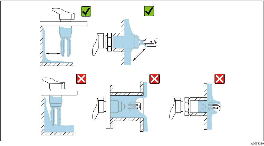
图 10 安装实例：测量高粘度过程介质
