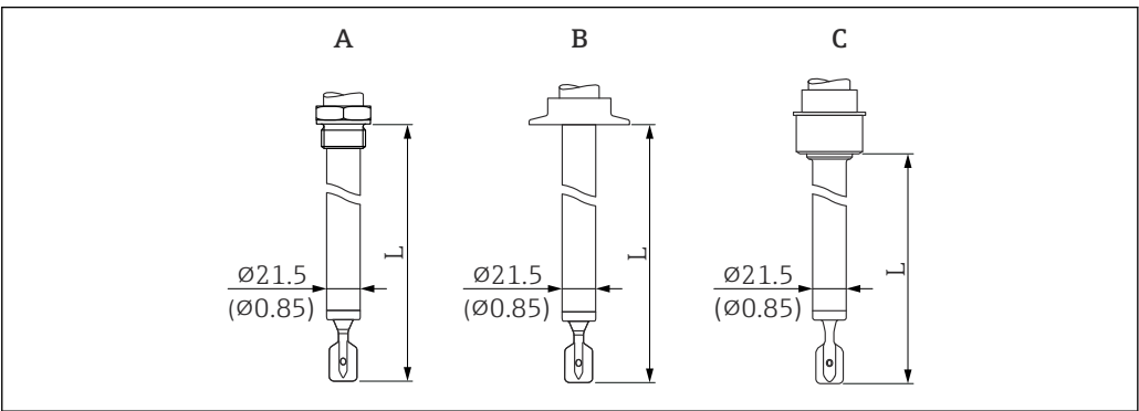
29 探头类型：延长管型、短管型；（传感器长度 L）。测量单位 mm (in)
