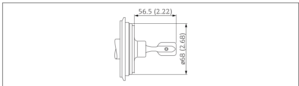
37 Varivent N 型接头, DN65-162 PN25 配合管道。测量单位 mm (in)
