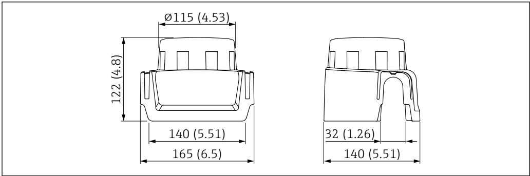
图 43 防护罩，适用单腔体铝外壳。测量单位 mm (in)
