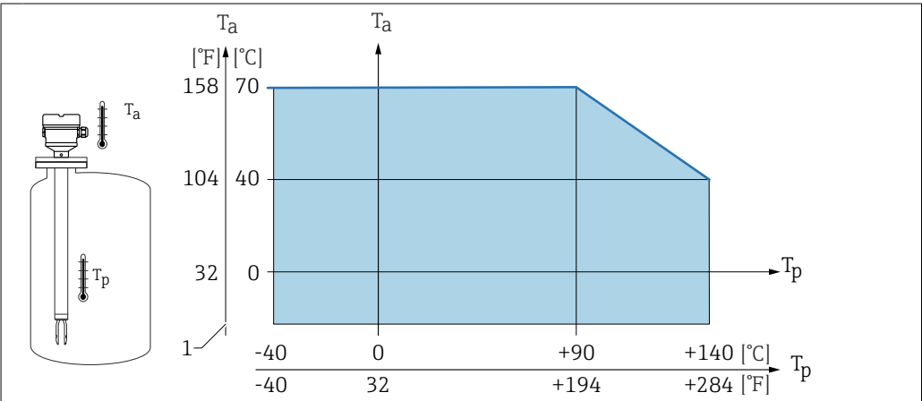
19 外壳允许环境温度 T_a 与罐体内部过程温度 T_p 的关系
