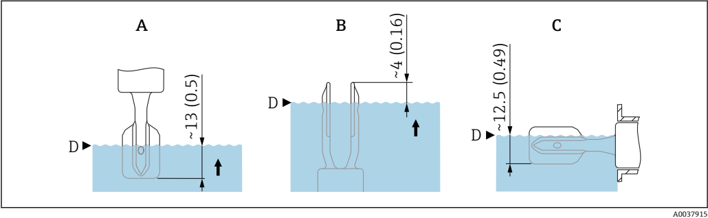
图 5 常见开关点。测量单位 mm (in)
