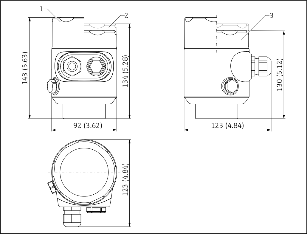
图 25 单腔体 316L 外壳（卫生型）的外形尺寸示意图。测量单位 mm (in)
