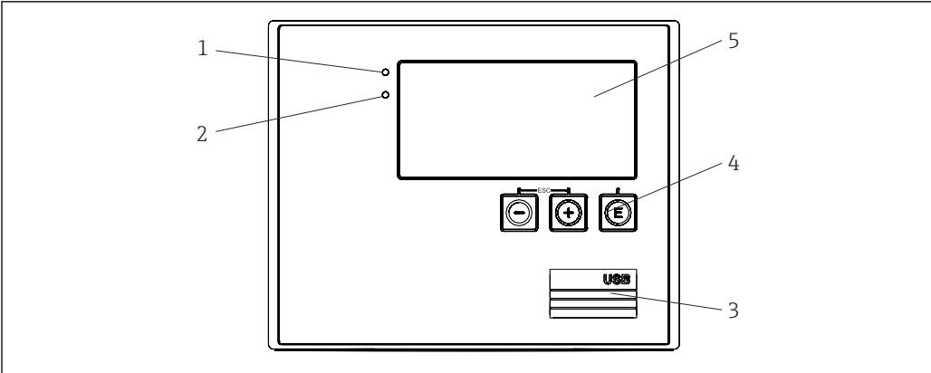
42 Display ed elementi operativi 1 LED verde, "Funzionamento" 2 LED rosso, "Messaggio di guasto" 3 Connessione USB per la configurazione 4 Tasti operativi: -, +, E 5 Display a matrice di punti 160x80
