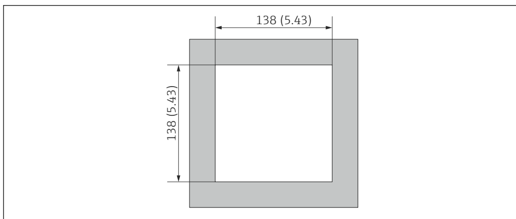
3 Dimensioni dell'apertura nel quadro in mm (in)
