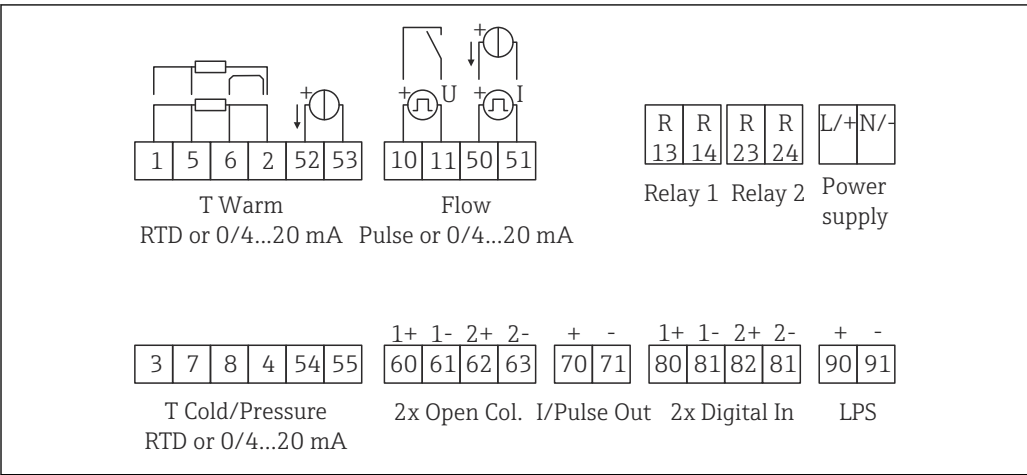
37 Assegnazione dei morsetti di EngyCal
