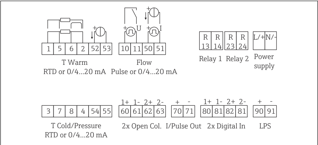
15 Schema di connessione del dispositivo
