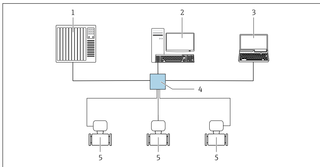
29 Opções para operação remota através da rede EtherNet/IP: topologia estrela
