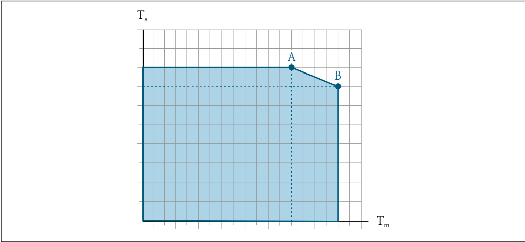
40 Representação exemplar, valores na tabela abaixo. T a Temperatura ambiente T m Temperatura do meio A Temperatura máxima permitida do meio T m a T a máx. = 60 °C (140 °F); temperaturas do meio mais altas T m requerem uma redução na temperatura ambiente T a B Temperatura ambiente T a máxima permitida para a temperatura média T m máxima especificada do sensor
