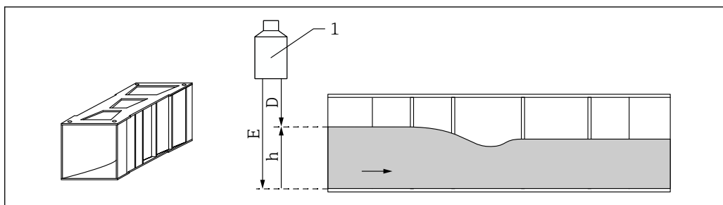
図 46 フリュームの空校正
