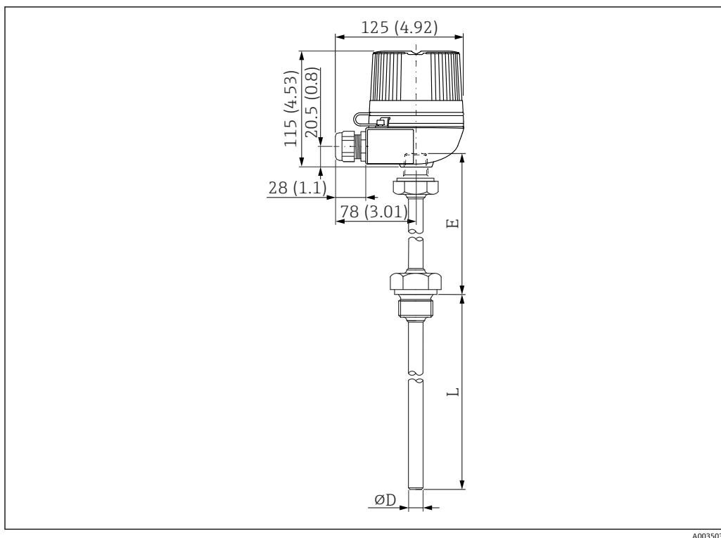
図 70 Omnigrad S TR61 の構成 ; 寸法 : mm (in)
