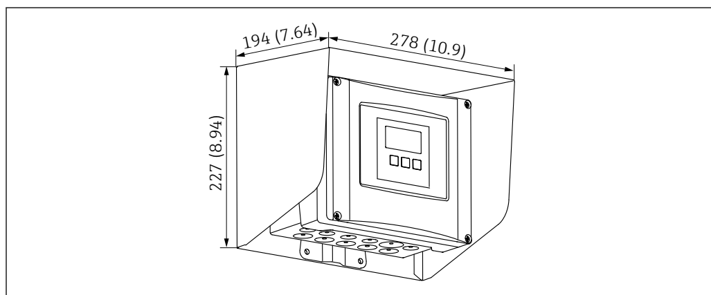
図 65 ポリカーボネート製フィールドハウジング用の日除けカバー。測定単位 mm (in)
