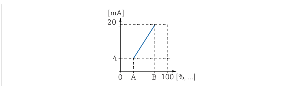
図 62 電流ターンダウンの動作原理
