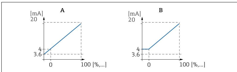
図 61 4mA しきい値（電流出力スパン = 4～20 mA の場合のみ）
