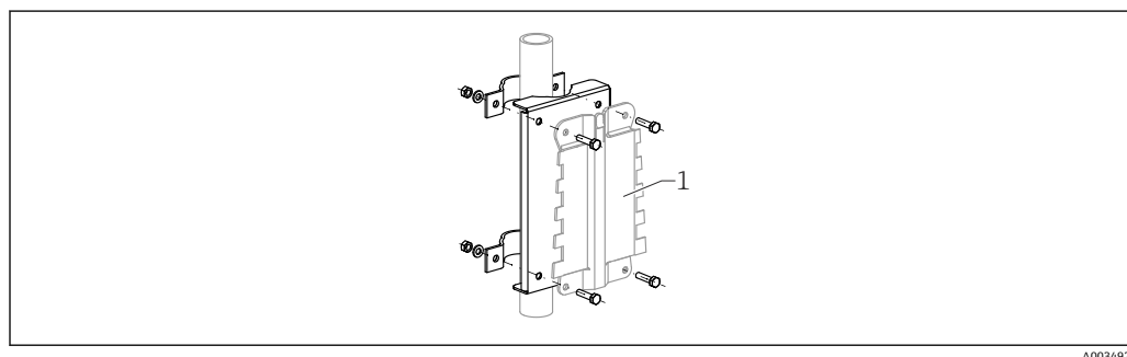
図 66 ポリカーボネート製フィールドハウジング用の取付プレート
