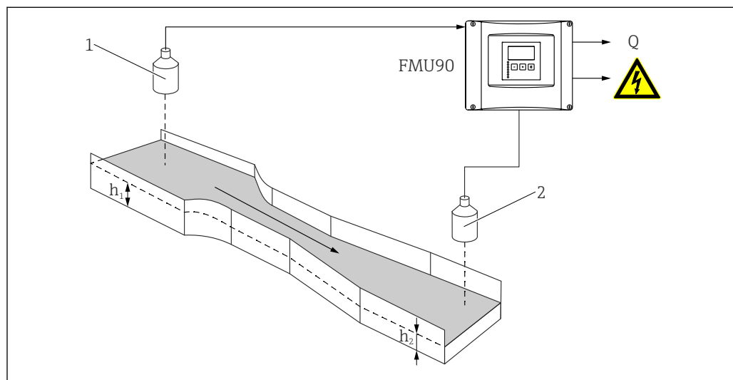
図 49 2つの超音波センサを使用したバックウォーターディテクション
