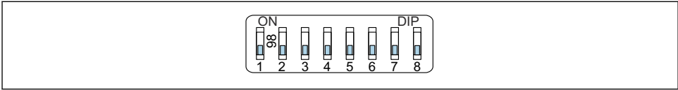
11 소프트웨어 주소 지정의 예: 스위치 8을 "OFF" 위치로 설정하고, 작업 메뉴에서 주소를 지정합니다.
