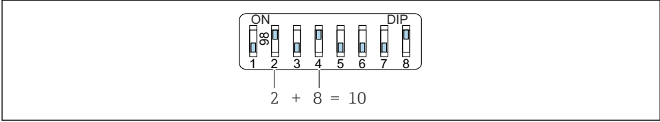
10 하드웨어 주소 지정의 예: 스위치 8을 "ON" 위치로 설정하고, 스위치 1 ~ 7을 사용해 주소를 지정합니다.
