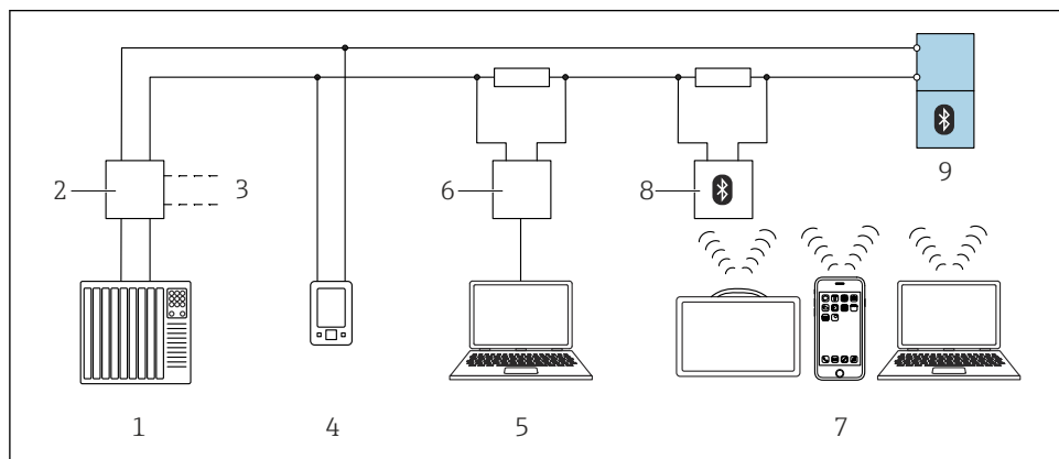
21 Варианты дистанционного управления по протоколу HART
