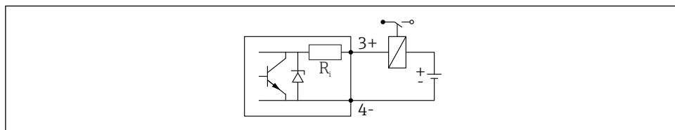
8 Пример подключения реле
