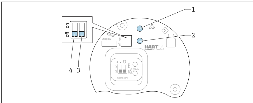
18 Кнопки управления и DIP-переключатели на электронной вставке HART
