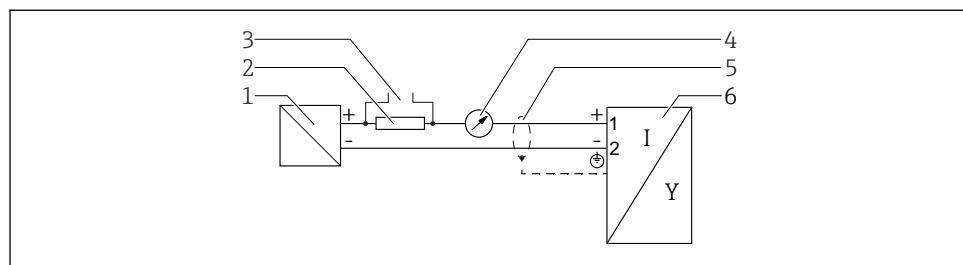
6 Функциональная схема 4 до 20 мА HART
