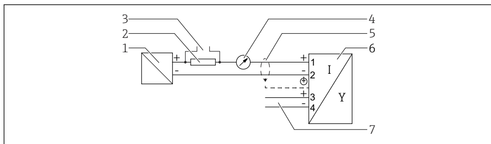
7 Функциональная схема 4 до 20 мА HART, релейный выход
