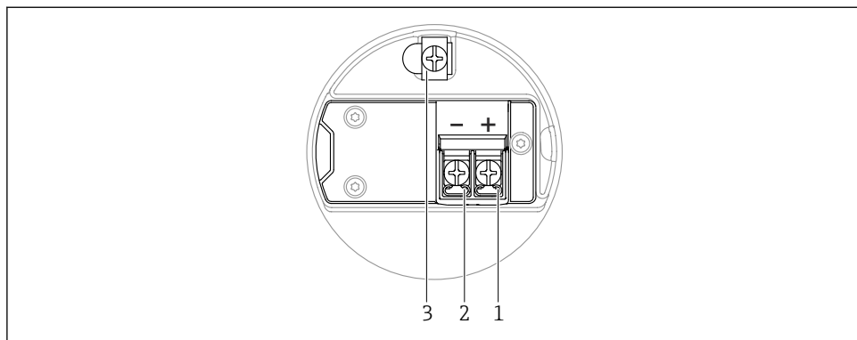
12 Назначение клемм в клеммном отсеке; 4 до 20 мА HART; корпус с двумя отсеками
