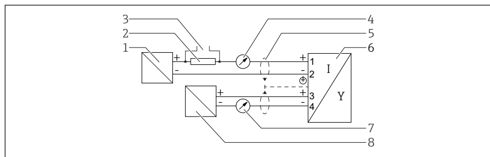
10 Функциональная схема 4 до 20 мА HART + 4 до 20 мА аналогов.
