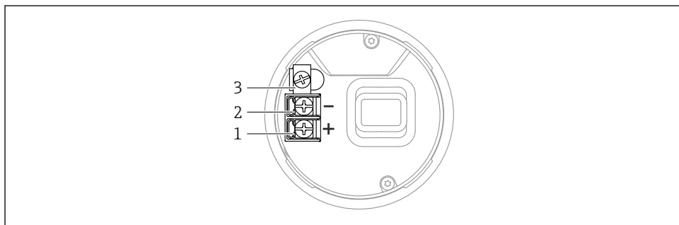
11 Клеммы подключения и клемма заземления в клеммном отсеке, корпус с одним отсеком
