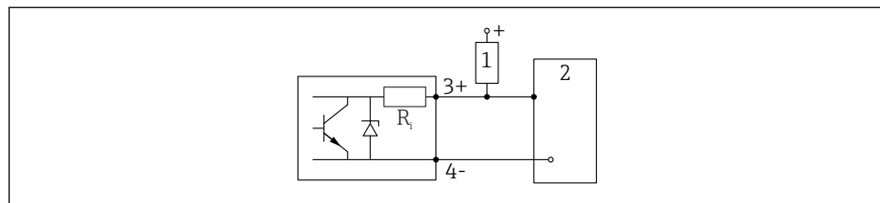
9 Пример подключения через цифровой вход
