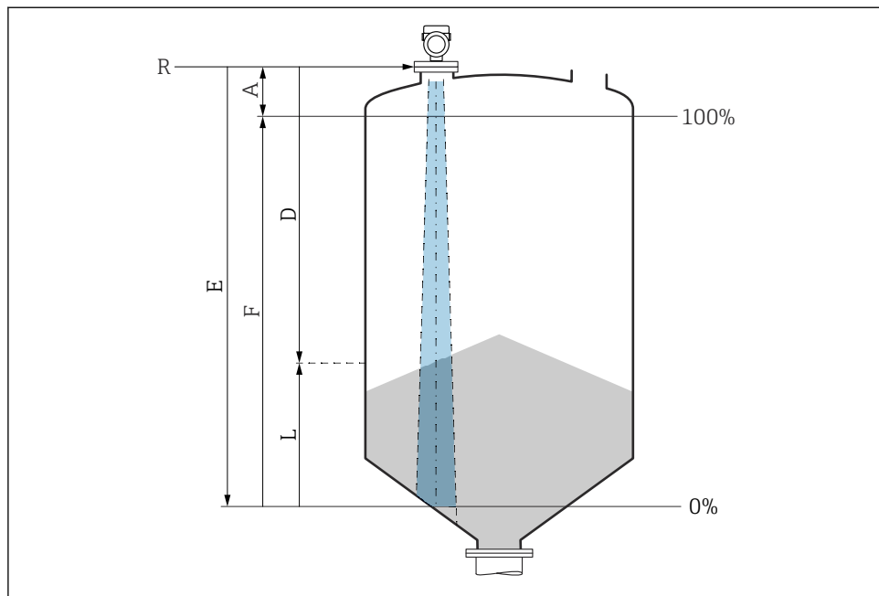
22 Параметры конфигурации для измерения уровня сыпучих сред
