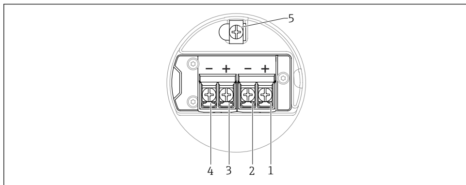
13 Назначение клемм в клеммном отсеке; 4 до 20 мА HART + 4 до 20 мА аналогов.; корпус с двумя отсеками
