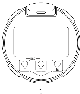
19 Графический дисплей с оптическими кнопками управления (1)
