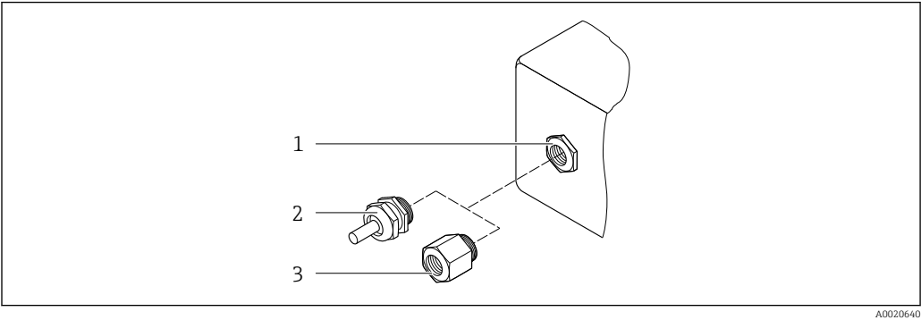
35 Возможные варианты кабельных вводов / кабельных уплотнений 1 Внутренняя резьба M20 × 1,5 2 Кабельное уплотнение M20 × 1,5 3 Переходник для кабельного ввода с внутренней резьбой G ½" или NPT ½"
