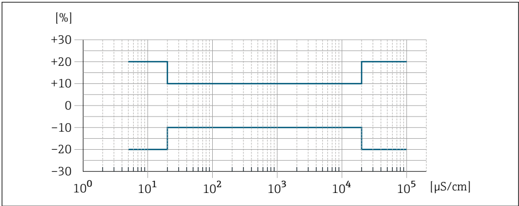
33 Погрешность измерения (стандартный вариант)
