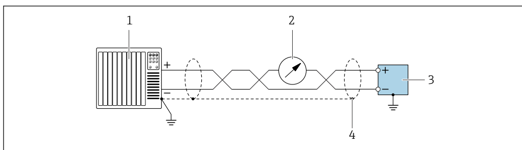
15 Пример подключения для токового выхода 4 до 20 мА (активного) с протоколом HART
