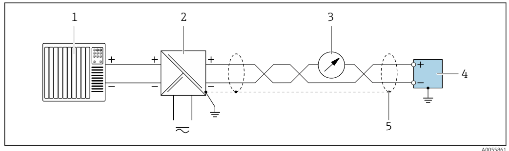
16 Пример подключения для токового выхода 4 до 20 мА (пассивного) с протоколом HART
