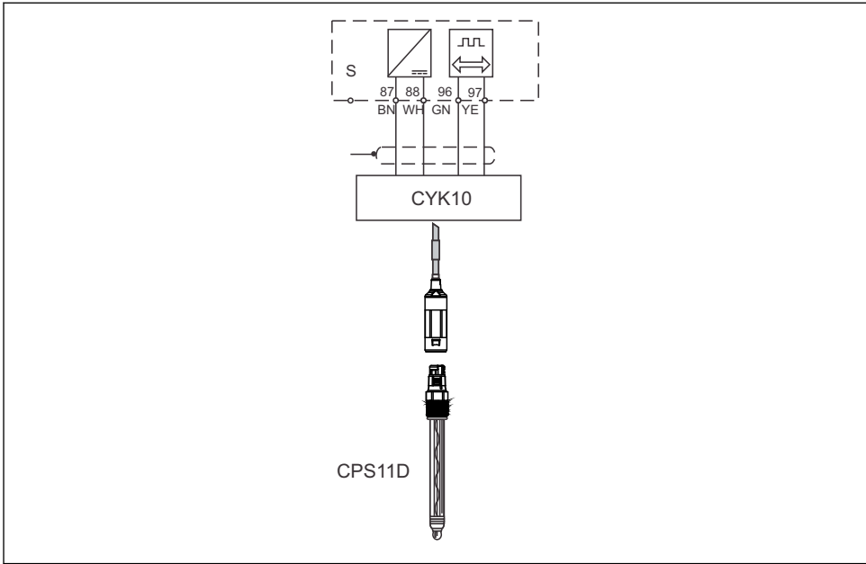
7 Exemplu de conexiune CPS11D cu CYK10
