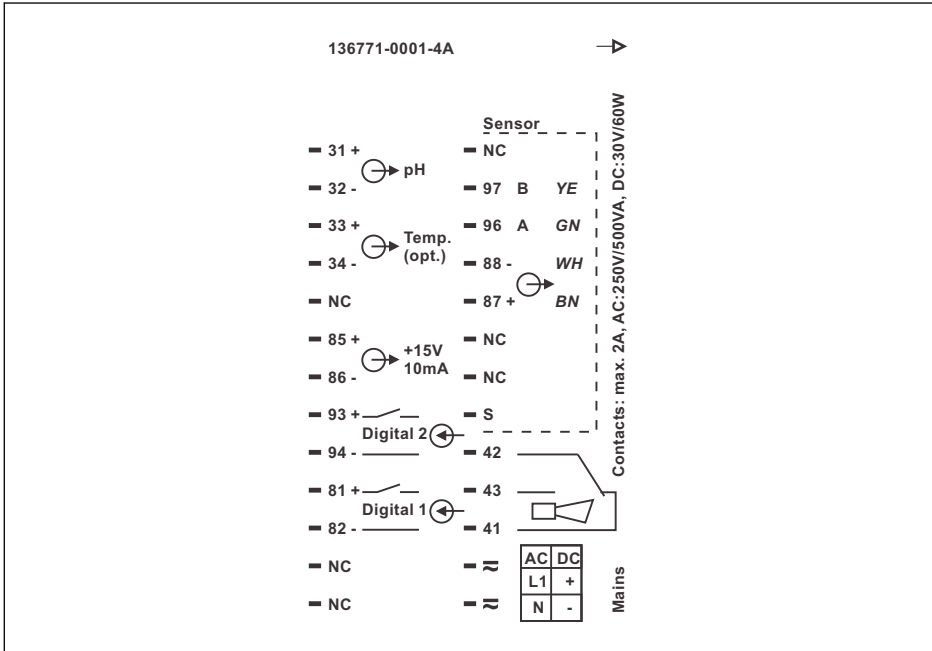
4 Etichetă conexiune/alocarea bornelor
