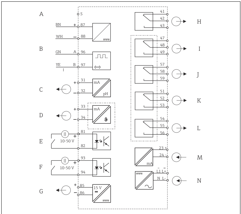
3 Conexiunea electrică a transmițătorului cu tehnologie Memosens
