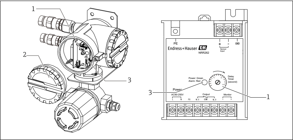
图 16 报警输出继电器 1 延迟微调器 2 盖板 3 LED 指示灯，电源（绿色）/报警（红色）
