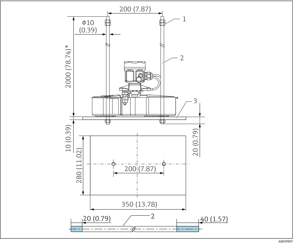
图 22 浮子导杆 1 螺母 (M10) 2 浮子导杆 3 重量
