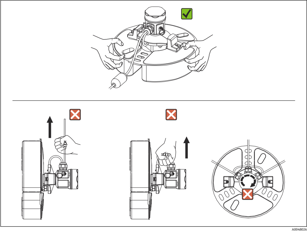
图 12 操作 NAR300
