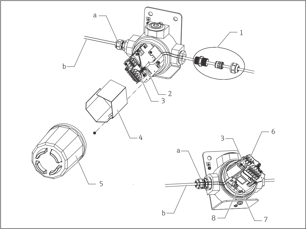
图 14 NAR300-x6xxxx 和防爆型传感器数据转换盒电缆安装
