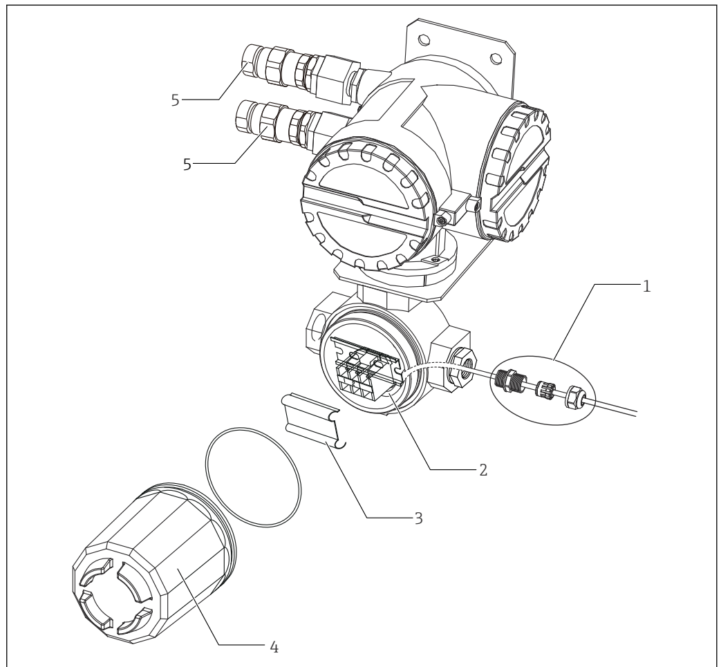
图 15 NRR261-5xx 电缆安装操作
