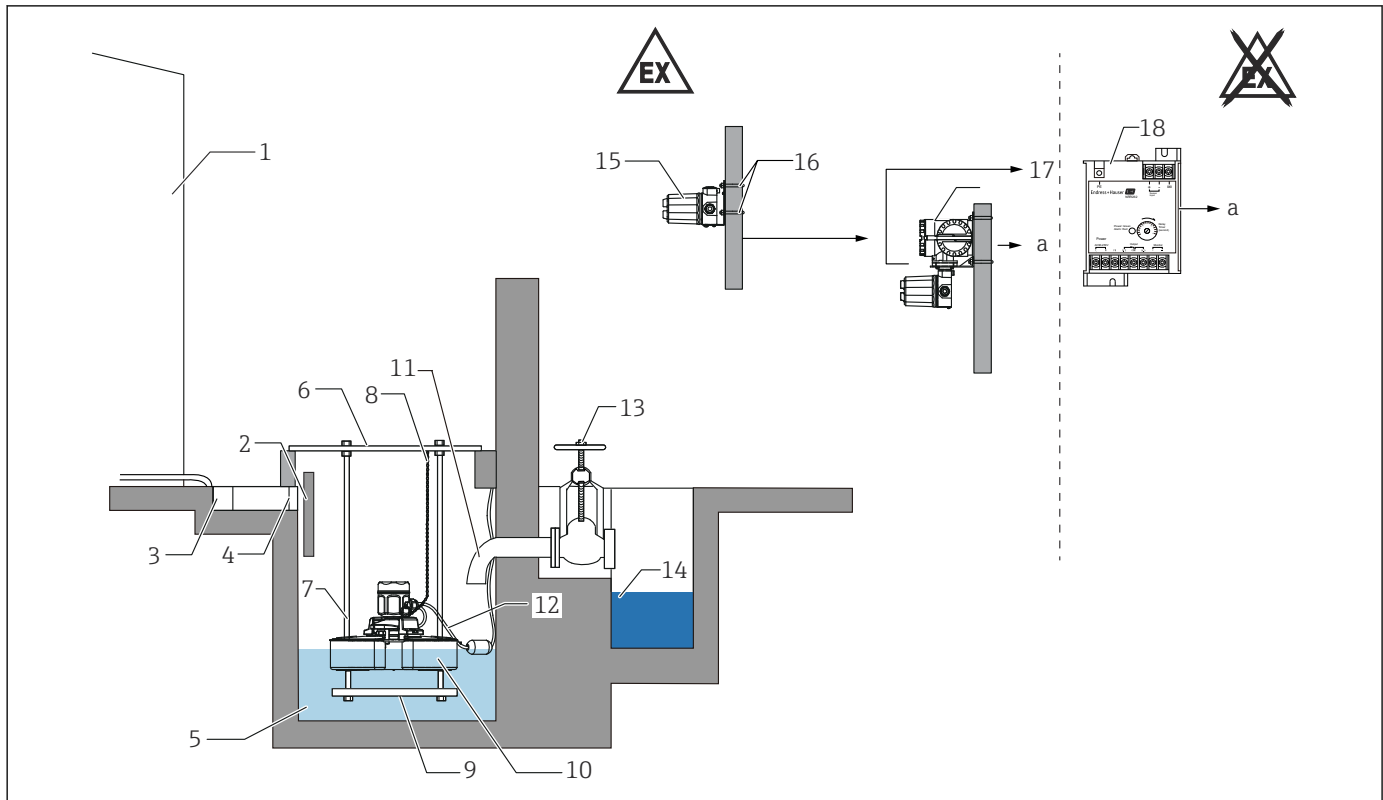
图 11 NAR300 + NRR26x
