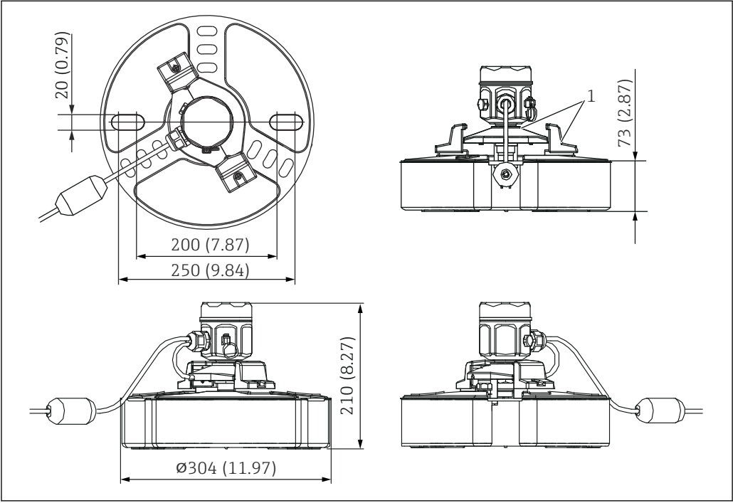
图 7 NAR300 浮子开关的外形尺寸示意图
