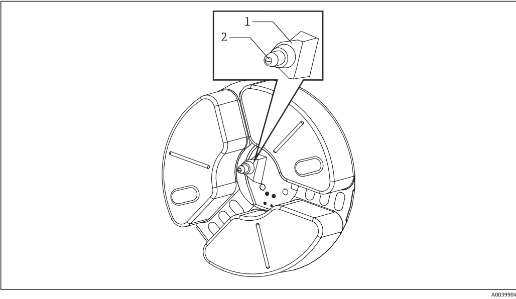
图 21 传感器清洁
