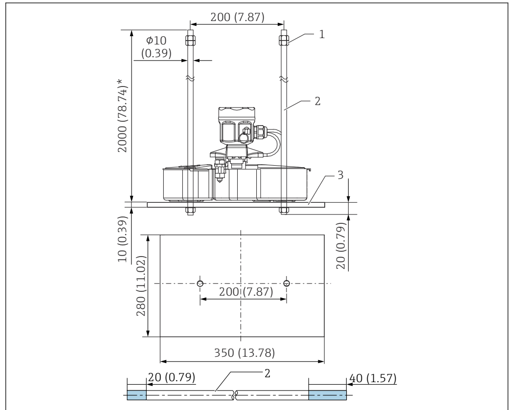
图 13 NAR300, 浮子导杆
