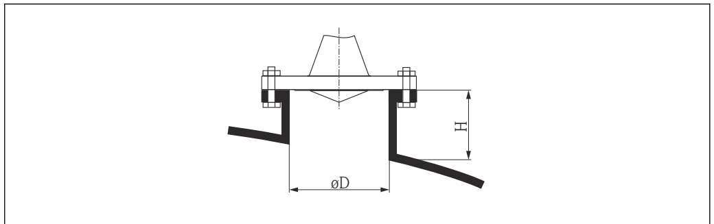
20 Diamètre et hauteur de piquage pour les antennes cornet avec bride tournante
