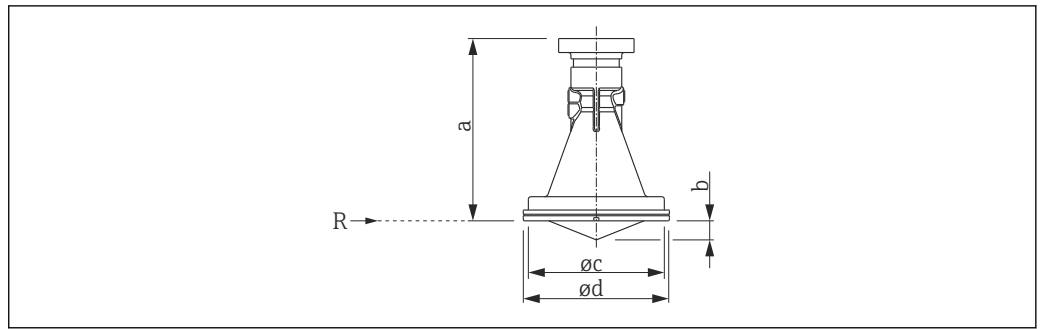
29 Dimensions du FMR56 sans raccord process. Unité de mesure mm (in)
