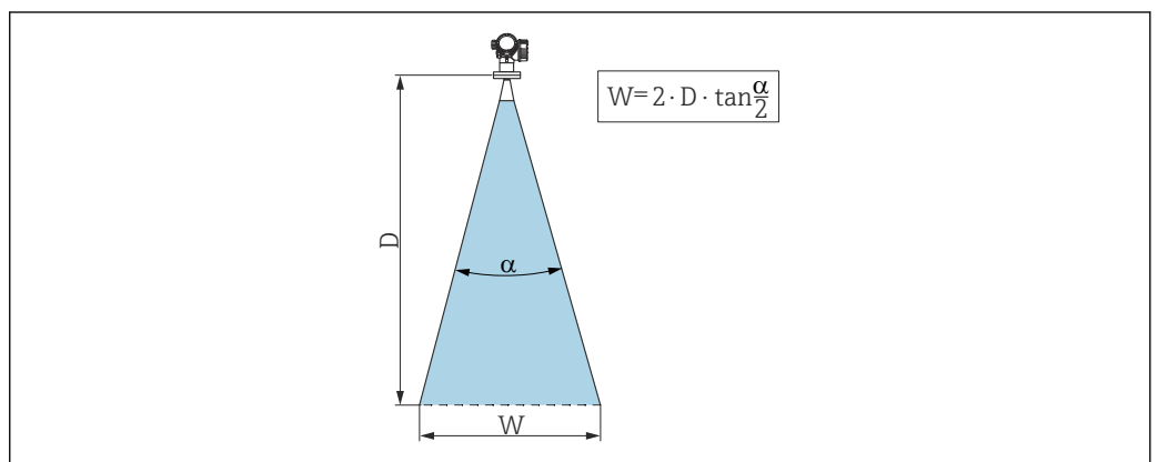
19 Relation entre l'angle de faisceau \alpha , la distance D et la largeur de faisceau W
