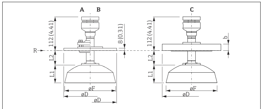
36 Dimensions du FMR57 avec antenne parabolique, unité de mesure : mm (in)
