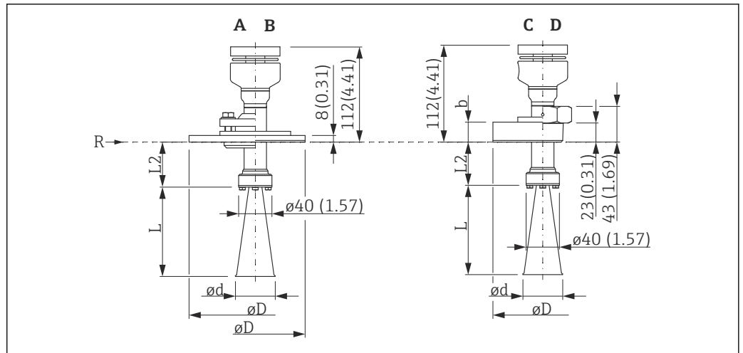
34 Dimensions du FMR57 avec antenne cornet - version standard. Unité de mesure mm (in)
