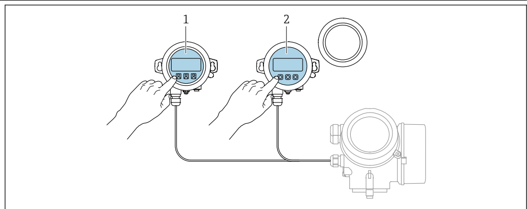
37 Possibilités de configuration via FHX50
