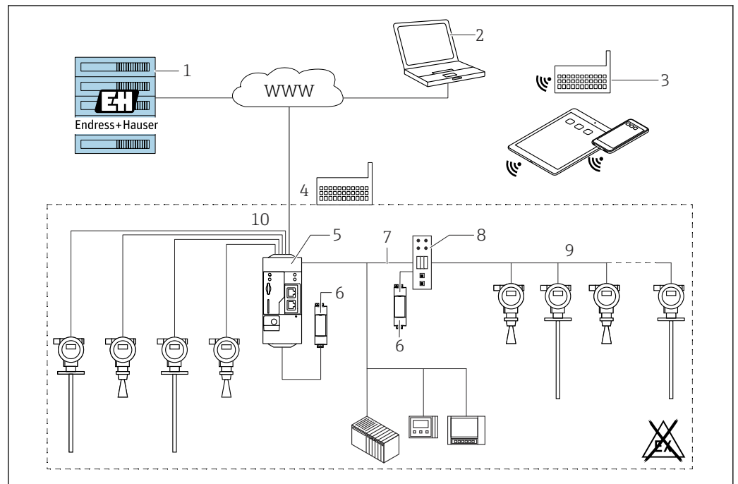
45 Exemple de plateforme de gestion des stocks avec SupplyCare Hosting SCH30
