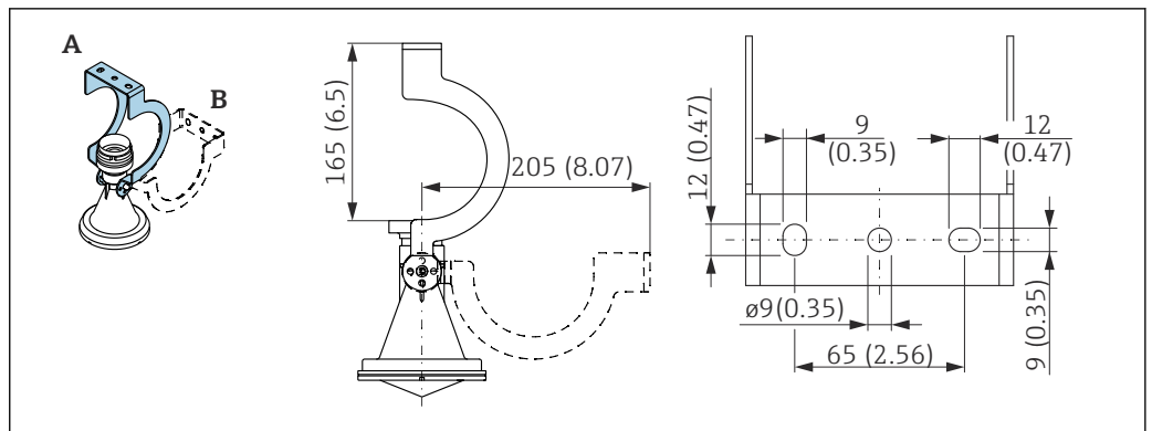
30 Dimensions de l'étrier de montage. Unité de mesure mm (in)
