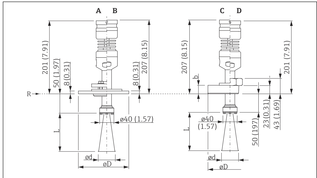
35 Dimensions du FMR57 avec antenne cornet - version haute température ; unité de mesure : mm(in)
