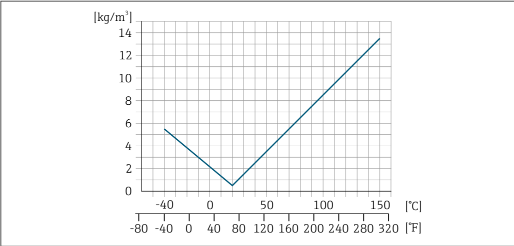
41 Felddichtejustierung, Beispiel bei +20 °C (+68 °F)
