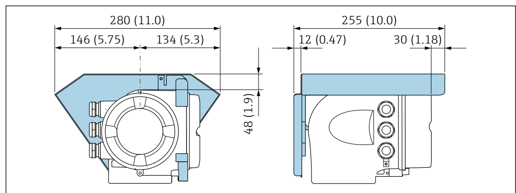
11 Wetterschutzhaube Proline 500; Einheit mm (in)
