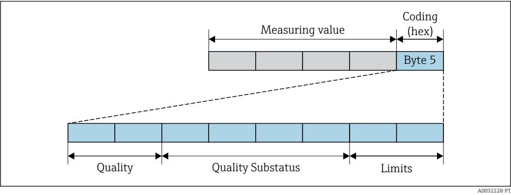
41 Estrutura do byte de codificação
