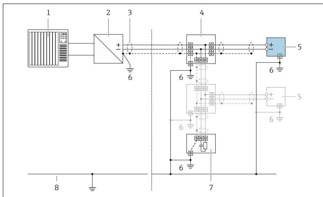
18 Exemplo de conexão para o PROFIBUS PA
