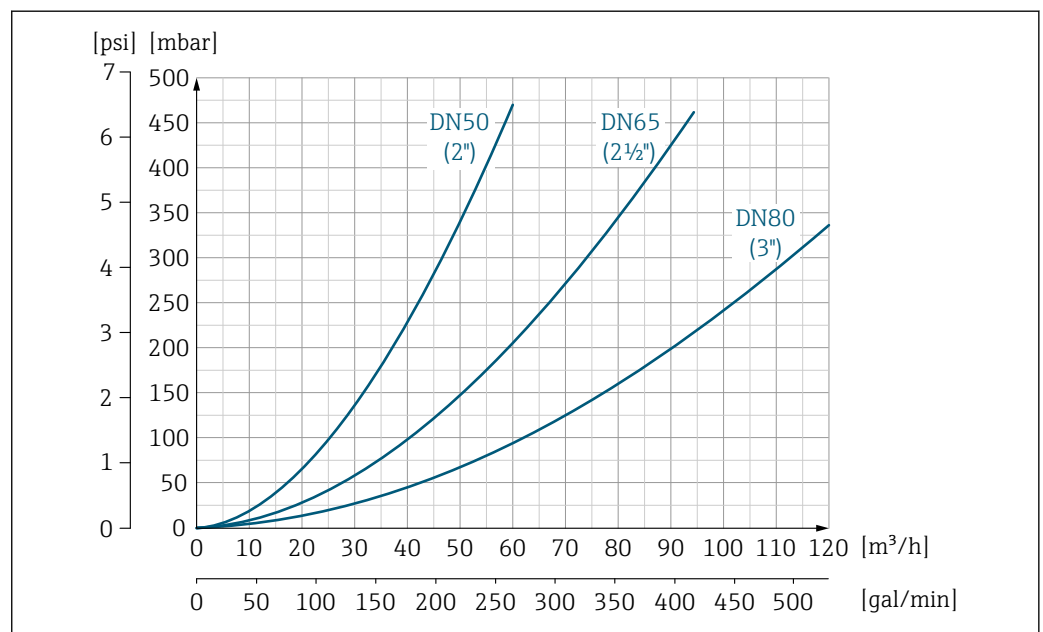
20 Pérdida de presión de DN 50 a 80 (de 2 a 3") para código de pedido para "Diseño", opción C "Brida fija, tubería de medición con contracción", 0 x DN tramos rectos de entrada/salida"
