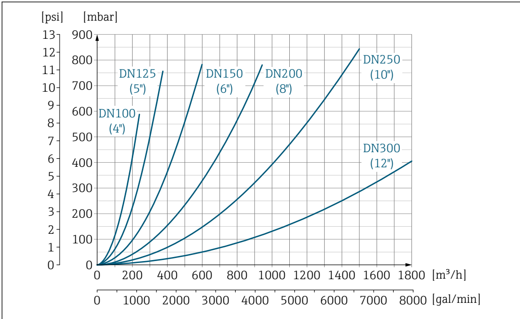
21 Pérdida de presión de DN 100 a 300 (de 4 a 12") para código de pedido para "Diseño", opción C "Brida fija, tubería de medición con contracción", 0 x DN tramos rectos de entrada/salida"
