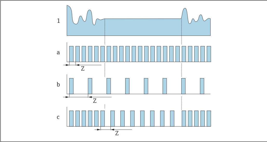
18 Principio de funcionamiento de varios métodos de registro de datos
