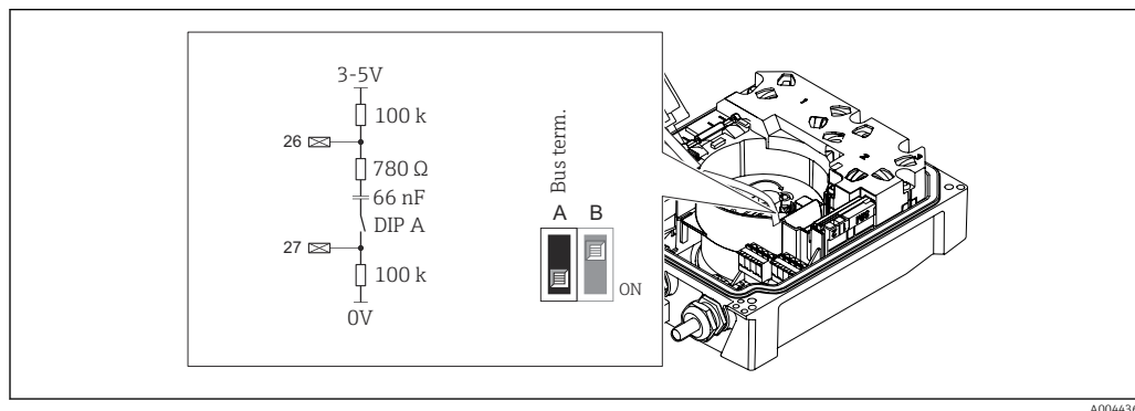
17 La resistencia de terminación se puede habilitar mediante el microinterruptor situado en el módulo del sistema electrónico
