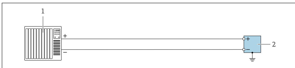
22 Esempio di collegamento per uscita impulsi/uscita frequenza/uscita contatto (attiva)
