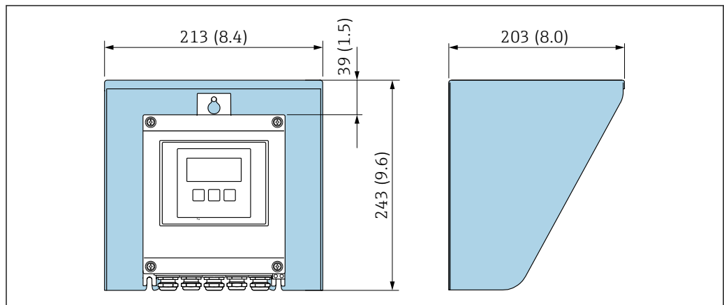
26 Capot de protection pour Proline 500 – numérique ; unité mm (in)
