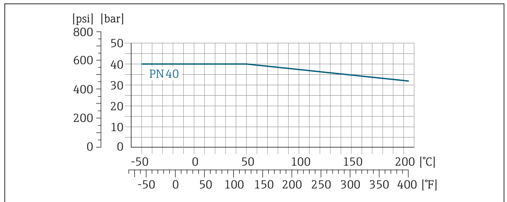
22 Avec matériau de bride 1.4301 (304) ; pièces en contact avec le produit : zirconium 702, tantale
