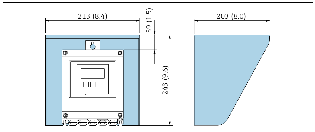
19 Capot de protection pour Proline 500 – numérique ; unité mm (in)
