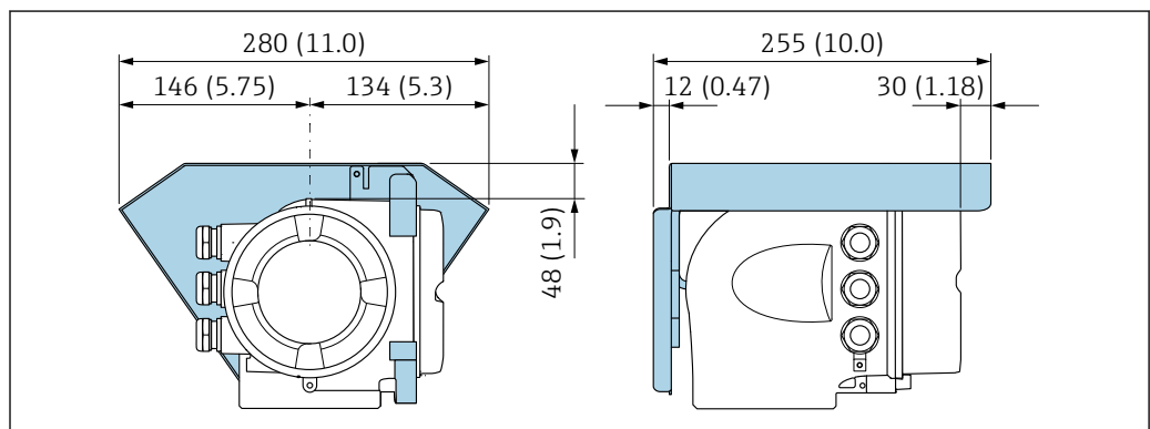
27 Capot de protection pour Proline 500 ; unité mm (in)
