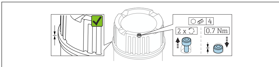
4 Dæksel med låseskrue
