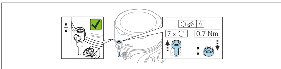
5 Dæksel med låseskrue; hygiejnisk hus (kun til støveksplodingsbeskyttelse)
