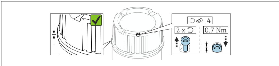
图 1 带锁定螺丝的外壳盖
