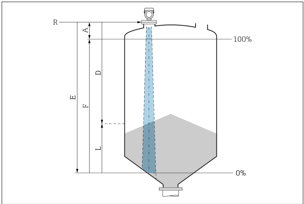
图 11 固体散料料位测量的设置参数
