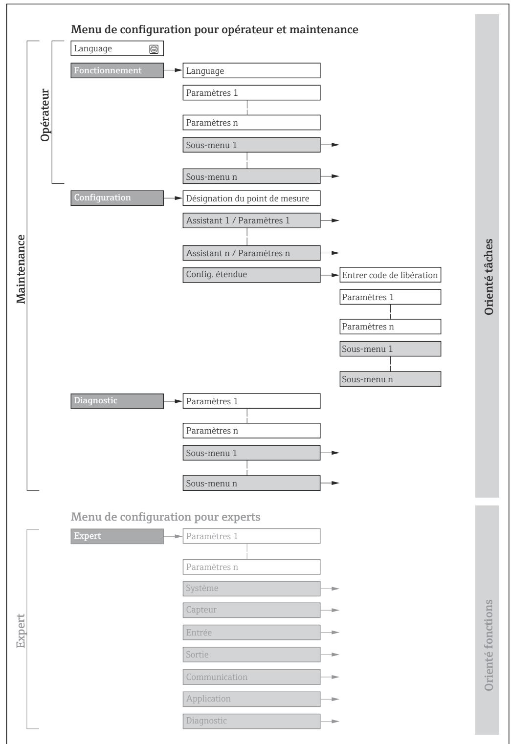
11 Structure schématique du menu de configuration
