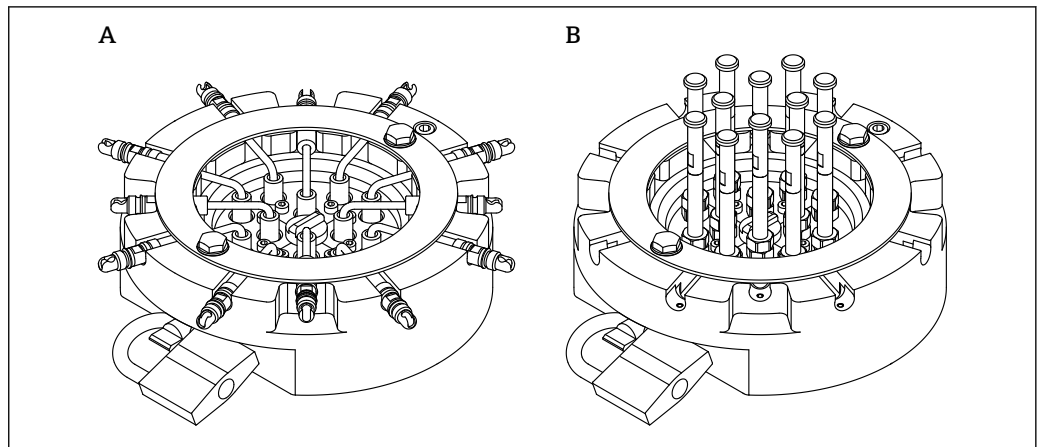
☞ 5 12개의 탈착식 방사선원이 있는 고정 링
