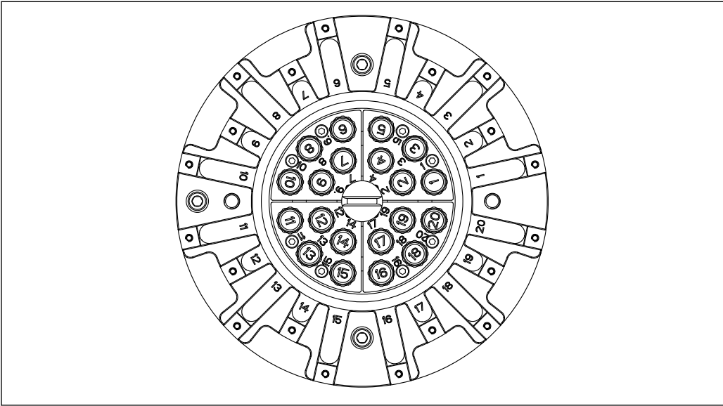
30 장착 개요, 방사선원 매거진(20자리)
