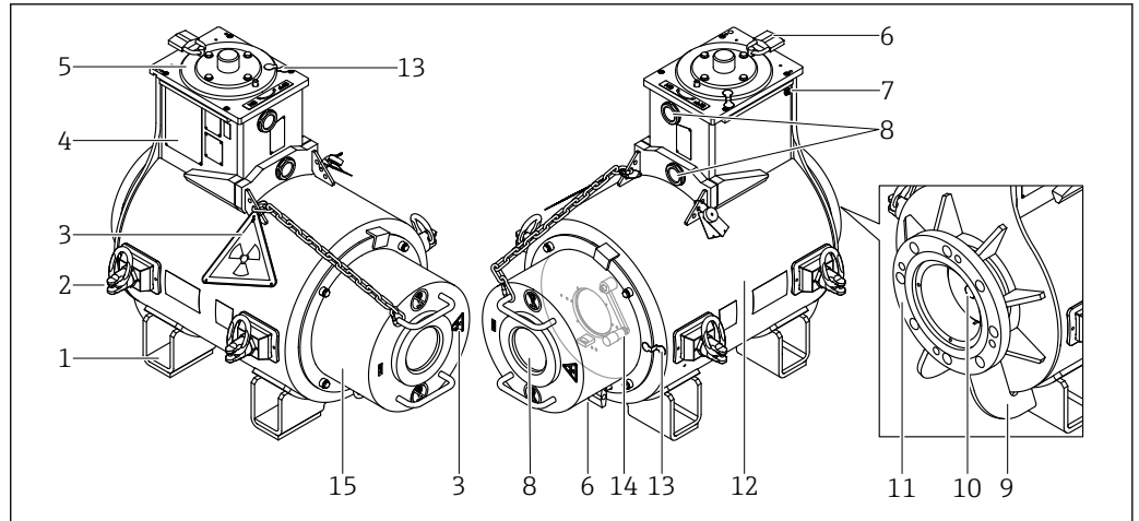
☐ 2 방사선원 컨테이너의 구성품 개요
