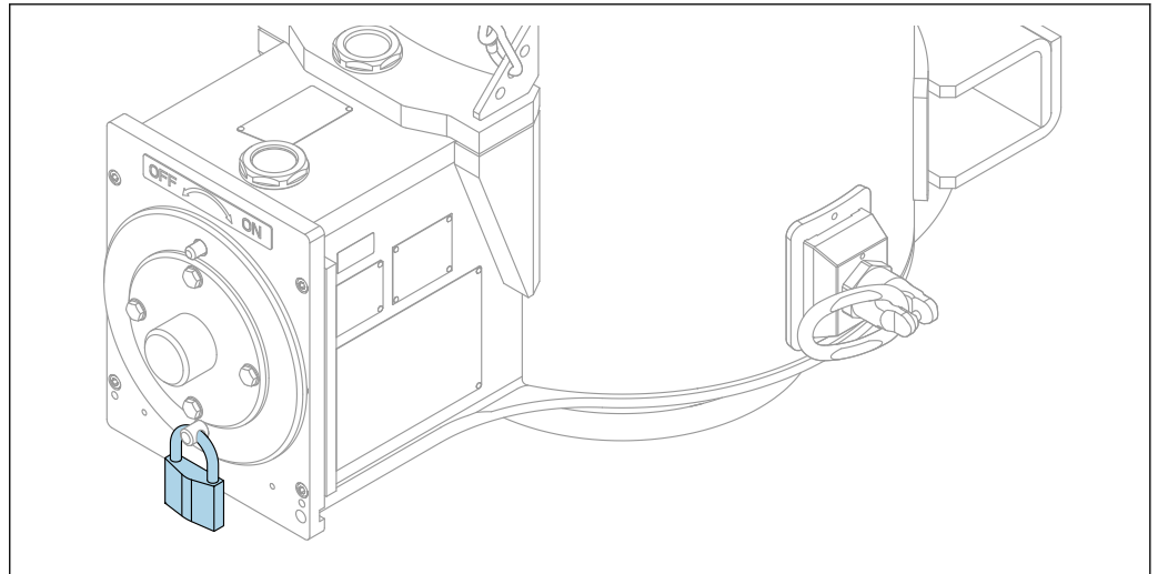
☐ 11 비틀림 방지 잠금 장치
