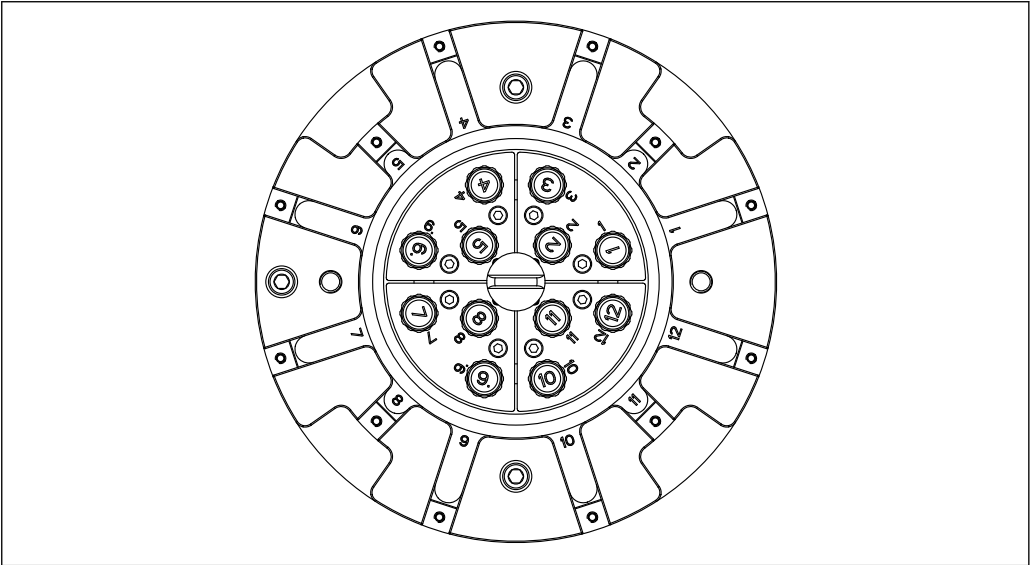
31 장착 개요, 방사선원 매거진(12자리)
