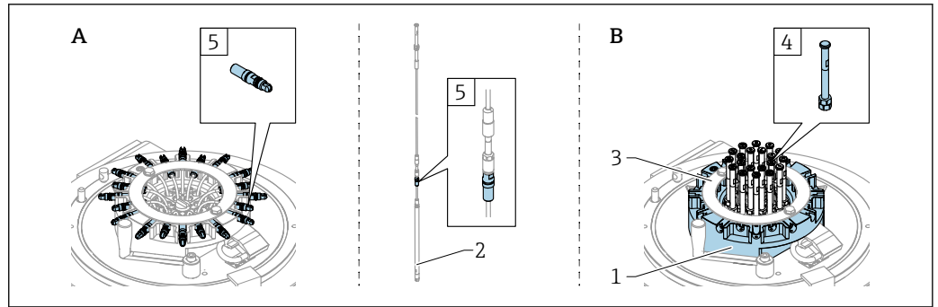
☐ 38 방사선원 매거진 및 방사선원 홀더
