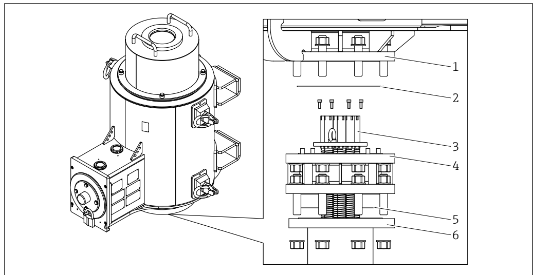
☐ 14 주름진 호스용 설치 어댑터
