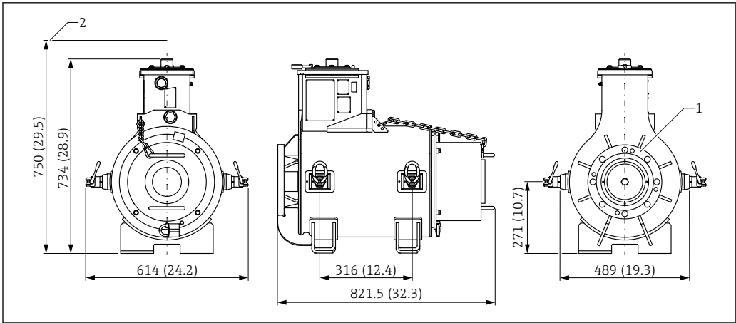
23 치수. 측정 단위 mm (in)
