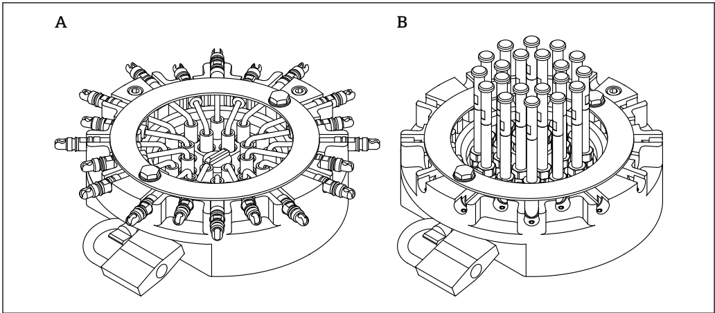
4 20개의 탈착식 방사선원이 있는 고정 링
