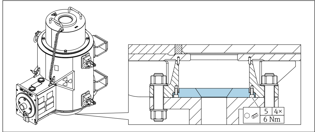
☐ 13 보호 파이프용 설치 어댑터
