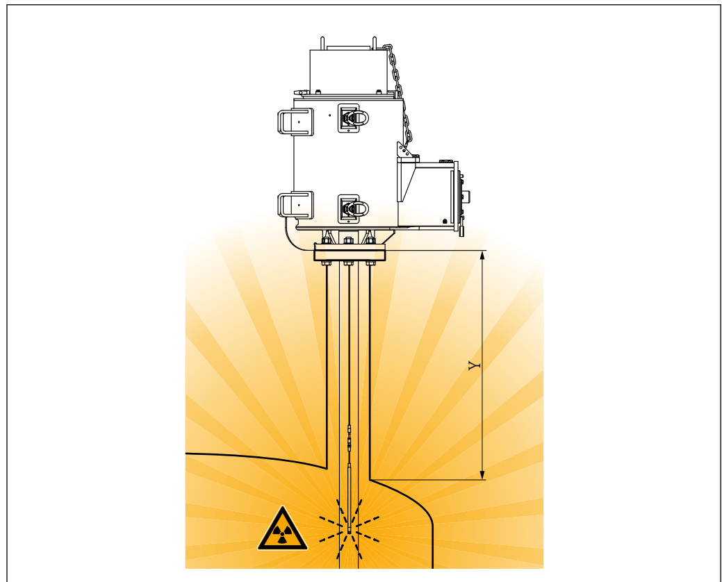
☞ 26 설치 치수
