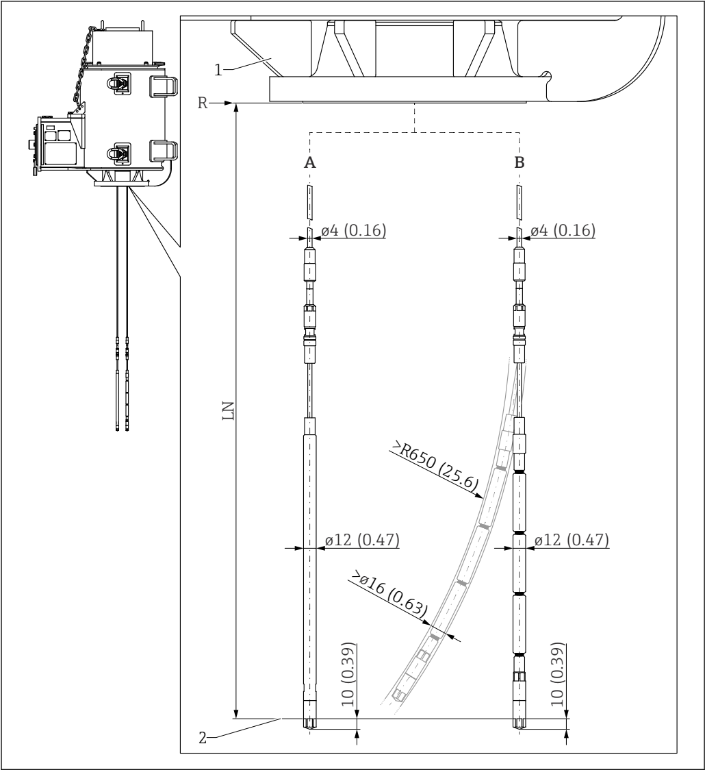
6 방사선원 홀더 버전 1 방사선원 컨테이너 A 로프 연장부 및 강성 방사선원 홀더(항목 025, 옵션 "A1", "B1") B 로프 연장부 및 연성 방사선원 홀더(항목 025, 옵션 "B3") R 기준점 LN 가변 공칭 길이(주문에 따라 다름)
