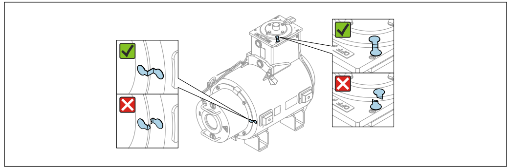
☞ 32 방사선원 컨테이너의 보안 씬
