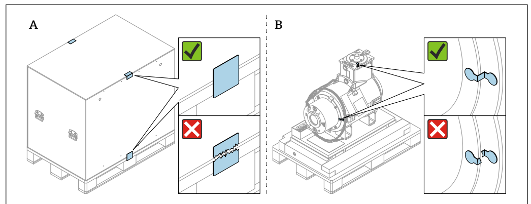
15 보호 씰 위치
