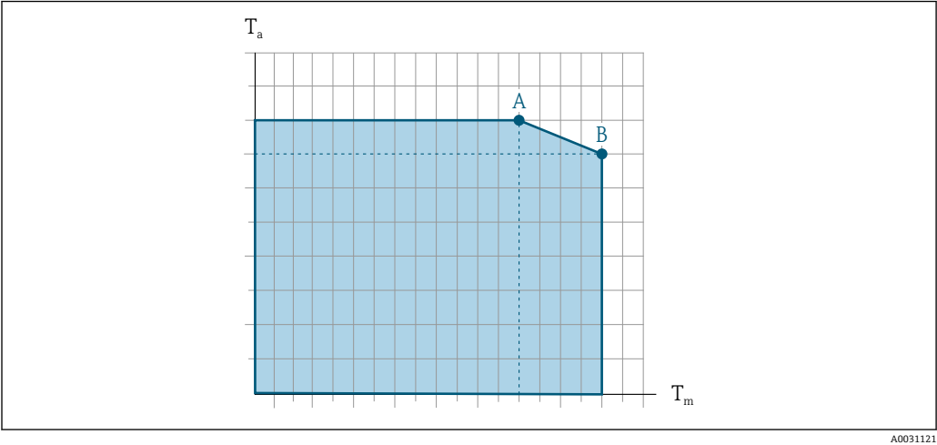
図 37 例示、値は下表を参照 Ta 周囲温度 Tm 測定物温度 A 許容最高測定物温度 Tm、Ta max = 60 °C (140 °F) 時；測定物温度 Tm が高い場合は、周囲温度 Ta を下げる必要があります。 B 規定されたセンサの最高測定物温度 Tm における許容最高周囲温度 Ta
