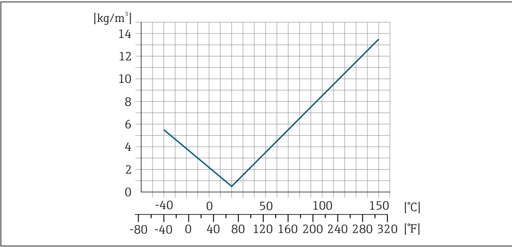
36 現場密度調整、例：+20 °C (+68 °F) 時
