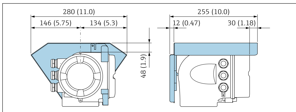
図 8 単位 mm (in)
