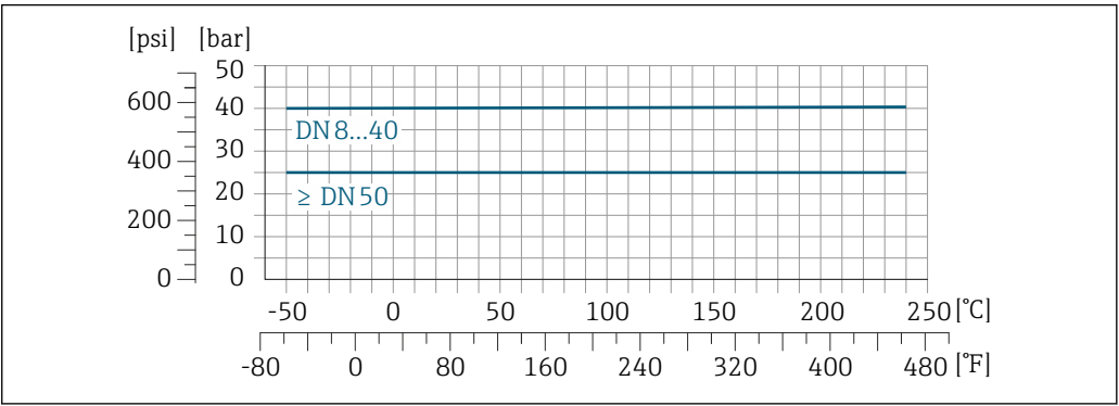
28 Avec matériau de raccord 1.4404 (316/316L)
