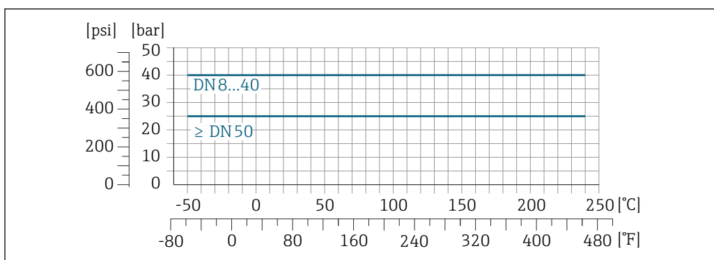
29 Avec matériau de raccord 1.4404 (316/316L)
