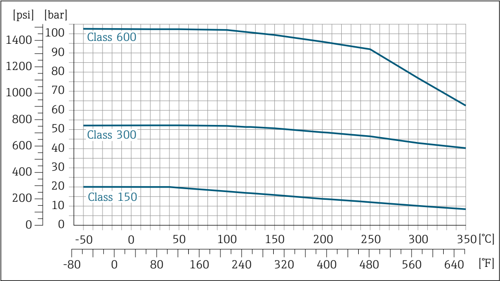
22 Avec matériau de bride Alloy C22
