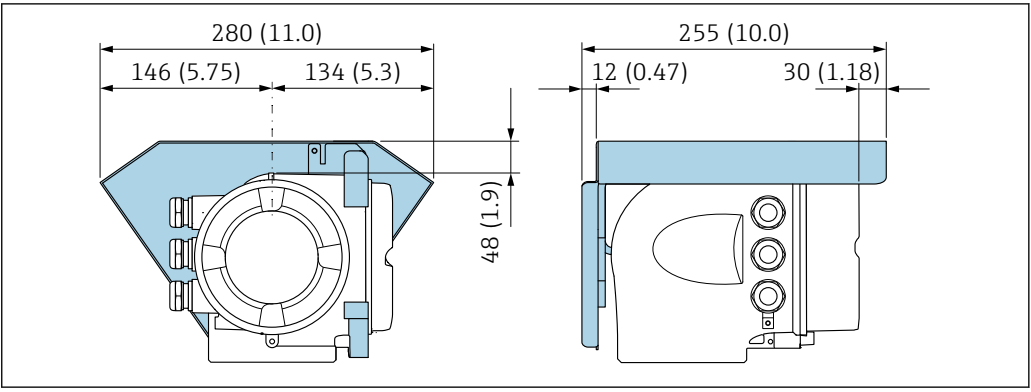
37 Capot de protection climatique pour Proline 500 – unité mm (in)
