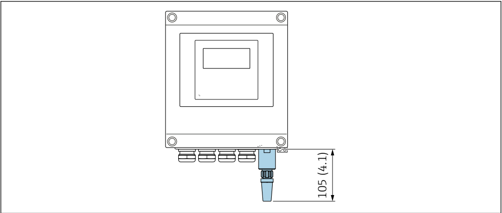
38 Unité mm (in)
