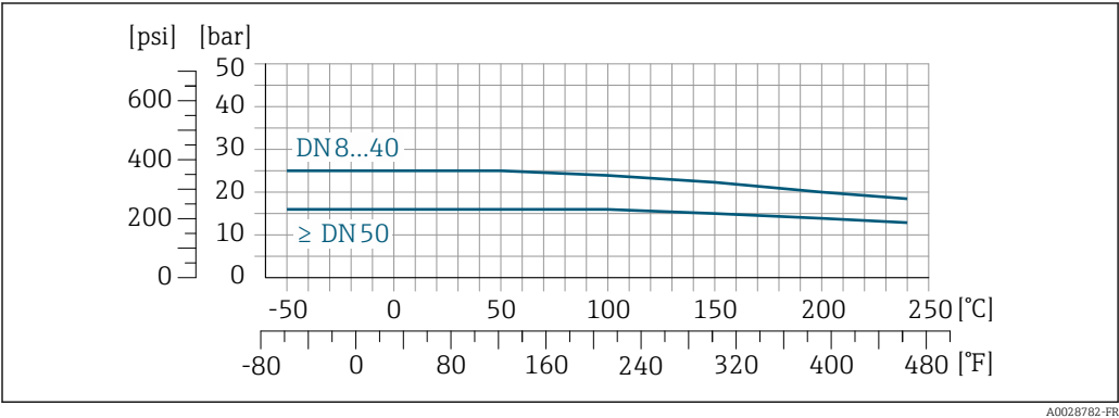
24 Avec matériau de raccord 1.4404 (316/316L)
