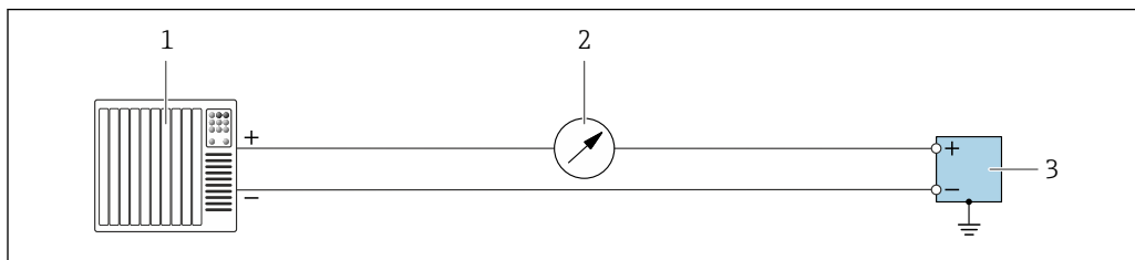
2 Exemple de raccordement pour sortie courant 4 ... 20 mA (active)
