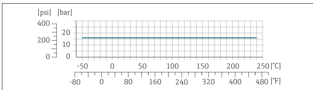
30 Avec matériau de raccord 1.4404 (316/316L)
