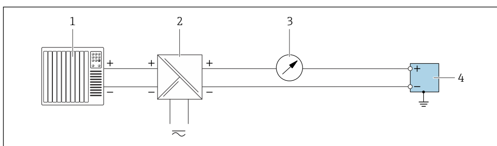
3 Exemple de raccordement pour sortie courant 4 ... 20 mA (passive)
