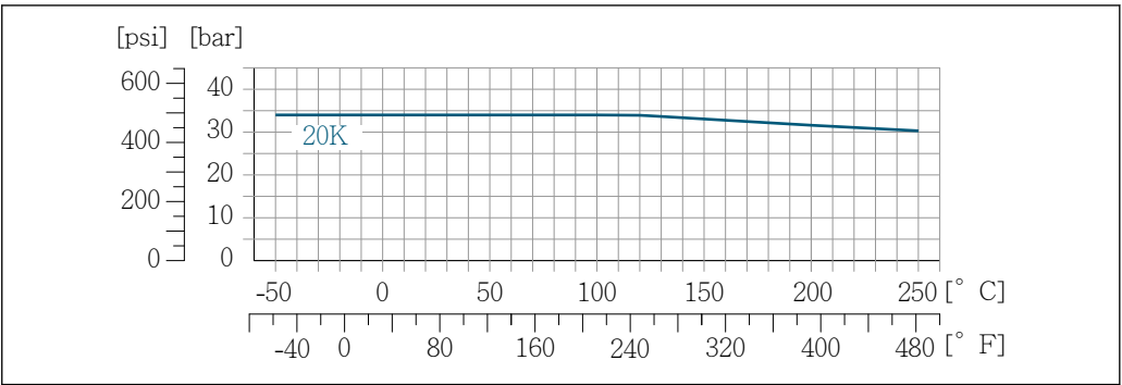
27 Avec matériau de bride 1.4301 (F304) ; pièces en contact avec le produit Alloy C22
