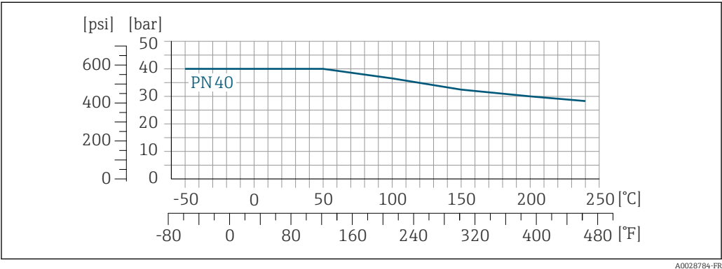
25 Avec matériau de bride 1.4301 (F304) ; pièces en contact avec le produit Alloy C22
