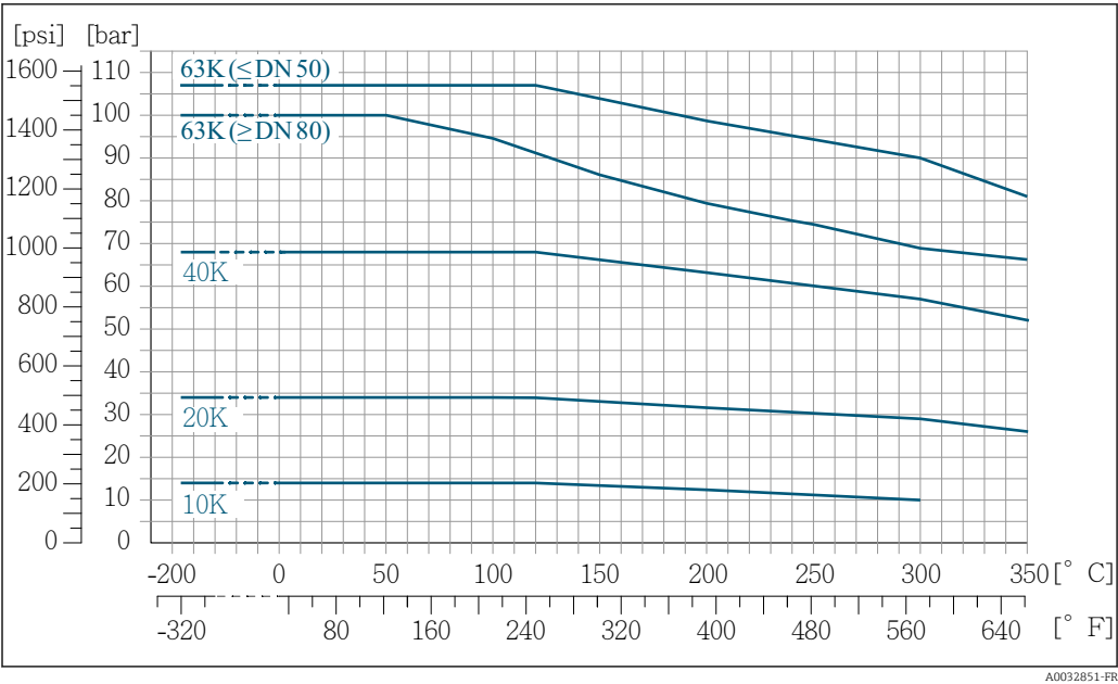
23 Avec matériau de bride 1.4404 (F316/F316L), Alloy C22
