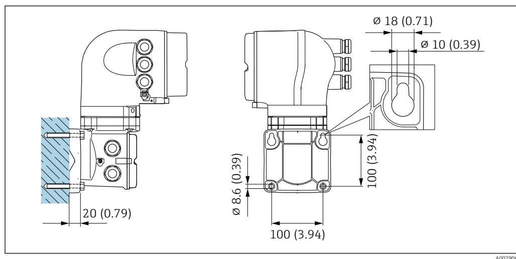
15 Unità mm (in)
