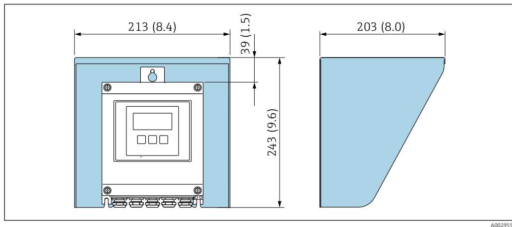
■ 11 Tettuccio di protezione dalle intemperie per Proline 500 – digital; unità ingegneristica mm (in)
