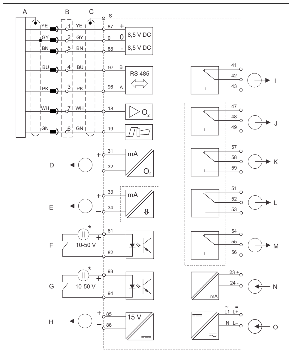
10 Elektrisk tilslutning af Liquisys M COM223/253 i WX- eller WS-version
