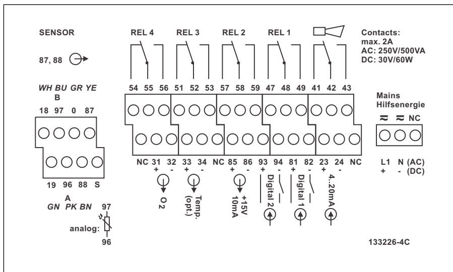
11 Liquisys M mærkat til tilslutningsrum, version WX/WS
