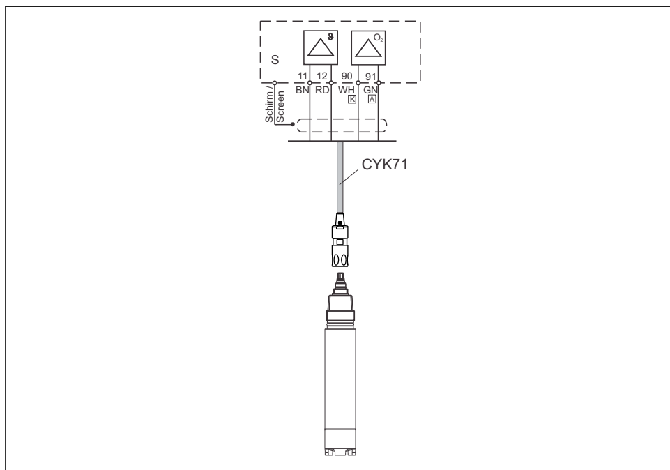
9 Tilslutningseksempel: COS41 med CYK71-kabel
