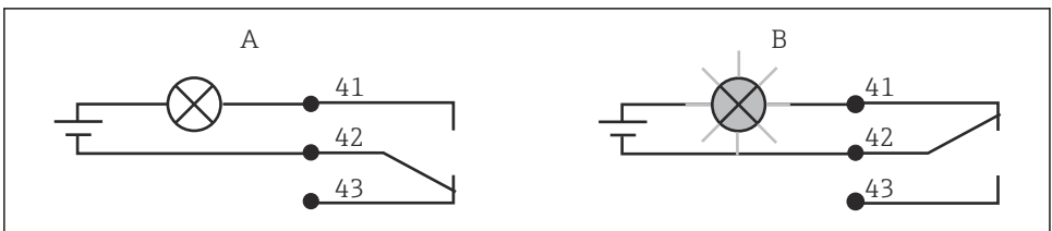
14 Anbefalet fejlsikker afbryder for alarmkontakten
