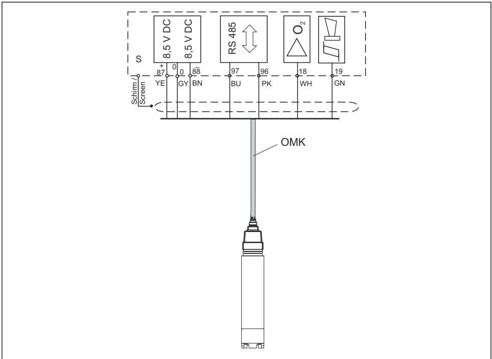
13 Tilslutningseksempel: COS31/71 med OMK-kabel
