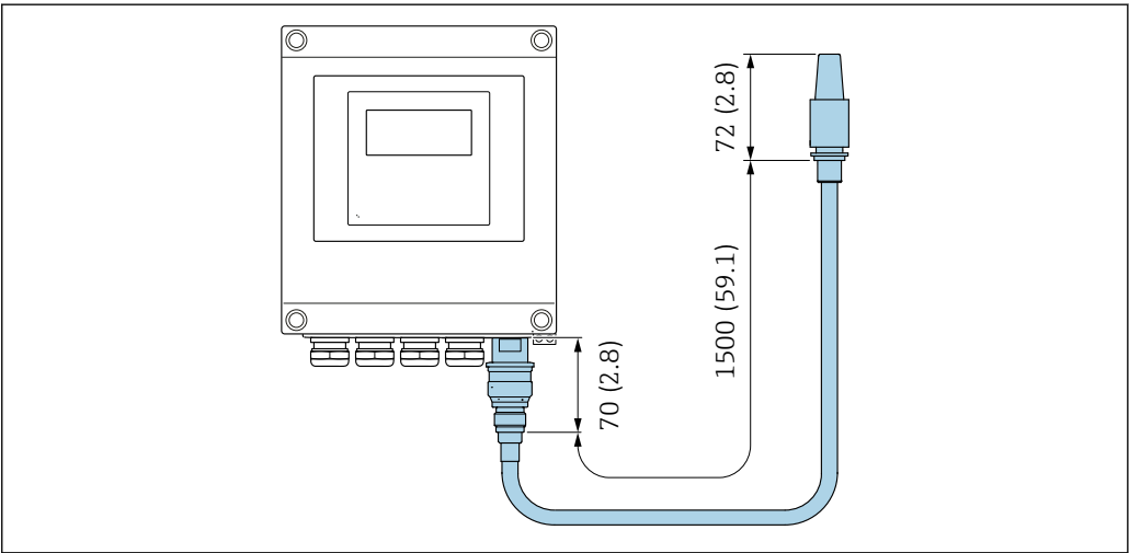
34 Unidad mm (in)
