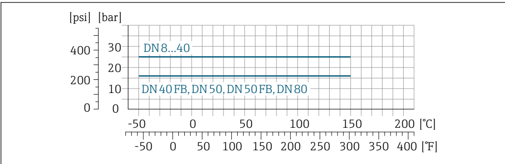
24 Con material de la brida titanio de grado 2
