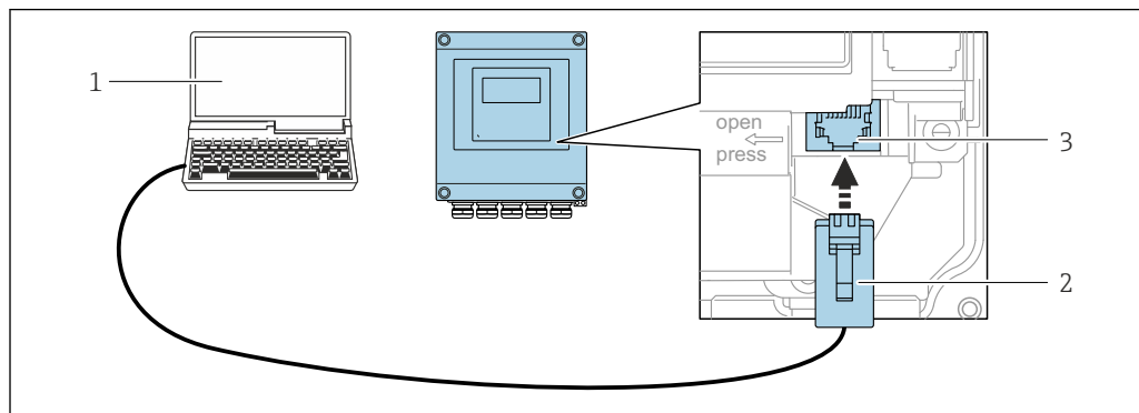
57 Conexión mediante la interfaz de servicio (CDI-RJ45)
