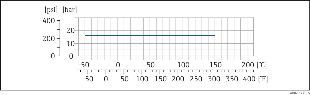
28 Con material de conexión titanio de grado 2
