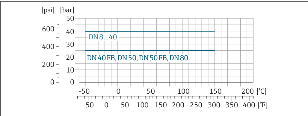
25 Con material de conexión titanio de grado 2
