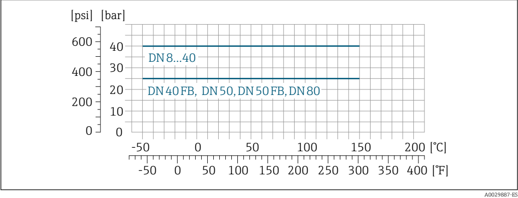
26 Con material de conexión titanio de grado 2
