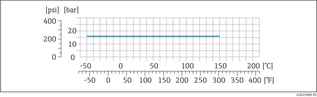
27 Con material de conexión titanio de grado 2
