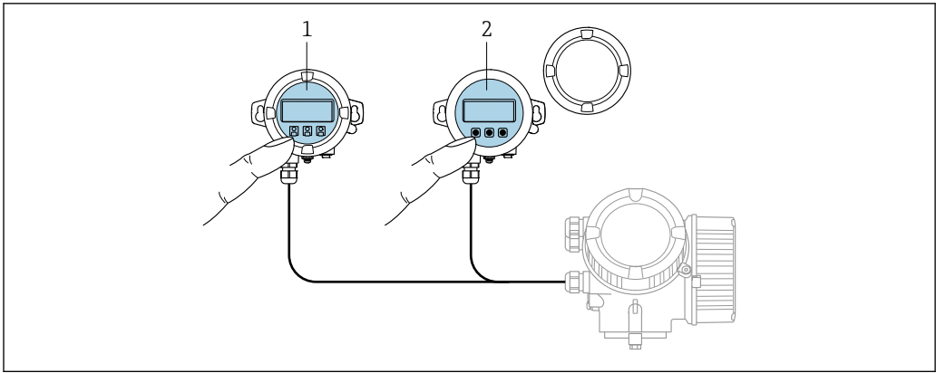
图 32 FHX50 的操作方式 1 SD02 显示与操作单元，按键；操作时必须打开盖板 2 SD03 显示与操作模块，光敏键：可以在玻璃盖外部操作
