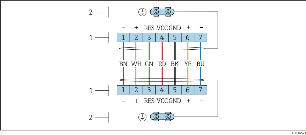
图 13 变送器墙装架中的接线腔和传感器接线盒内的接线端子
