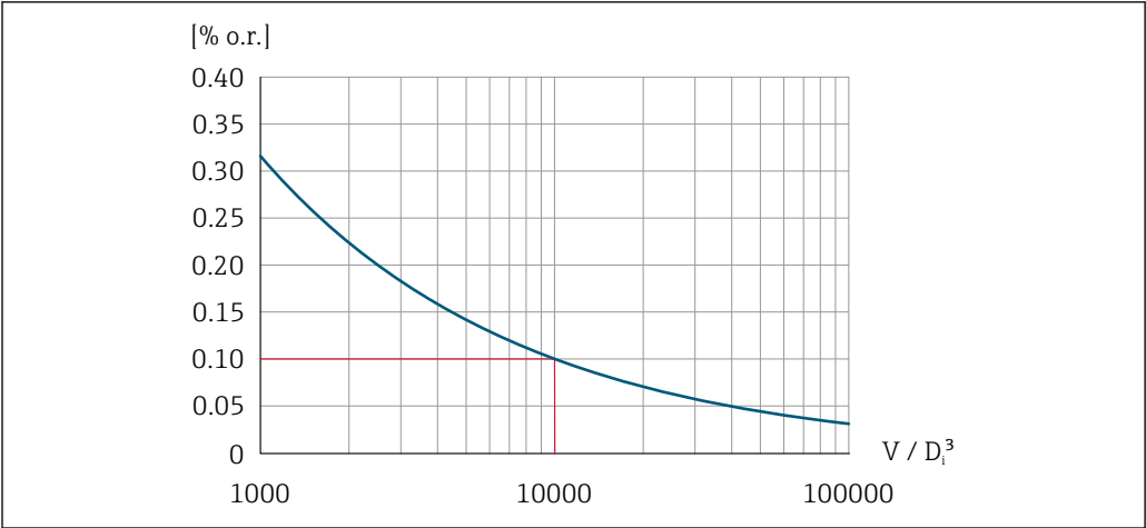
30 重复性 = 0.1 % o.r., 体积流量测量值[m³] of V = 10\,000 \cdot D_i^3
