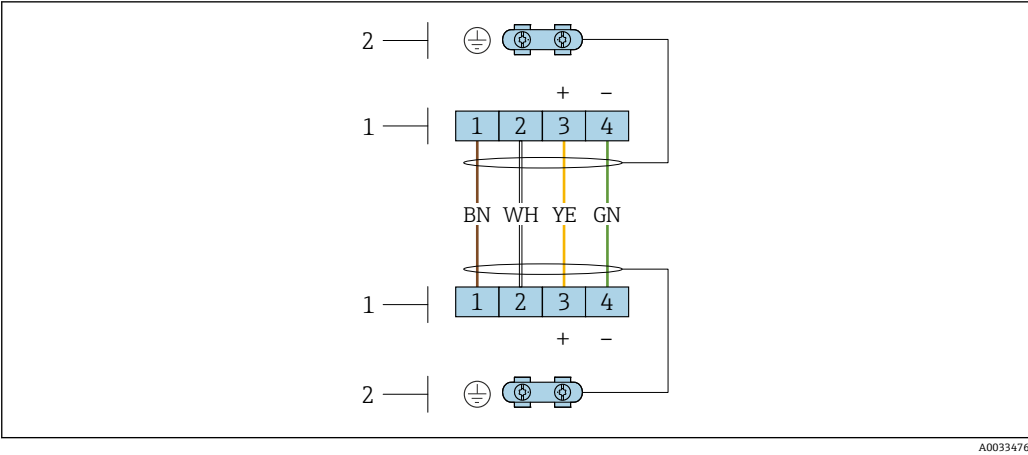
图 12 变送器墙装架中的接线腔和传感器接线盒内的接线端子
