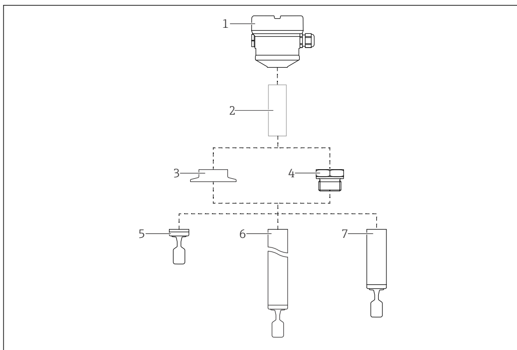
2 Конструкция изделия Liquiphant FTL63
