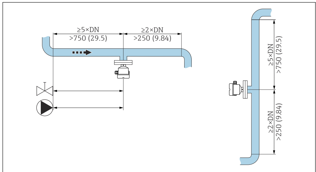
8 Монтаж прямого участка до прибора. Единица измерения мм (дюйм)
