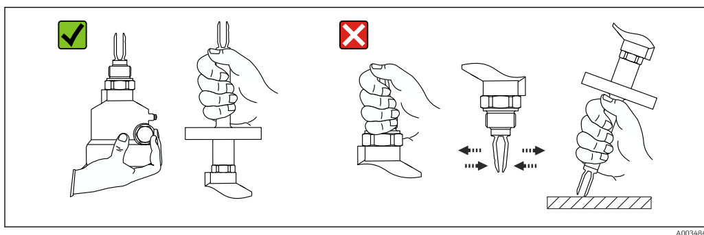
3 Удерживание прибора во время транспортировки
