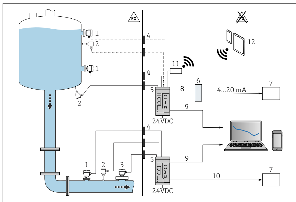
1 Измерение плотности с помощью вычислителя плотности QML51
