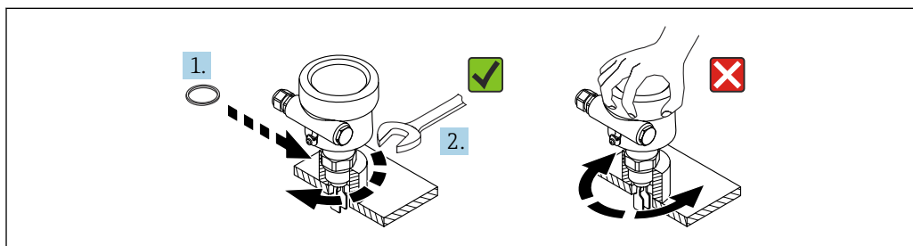
15 Прикручивание прибора
