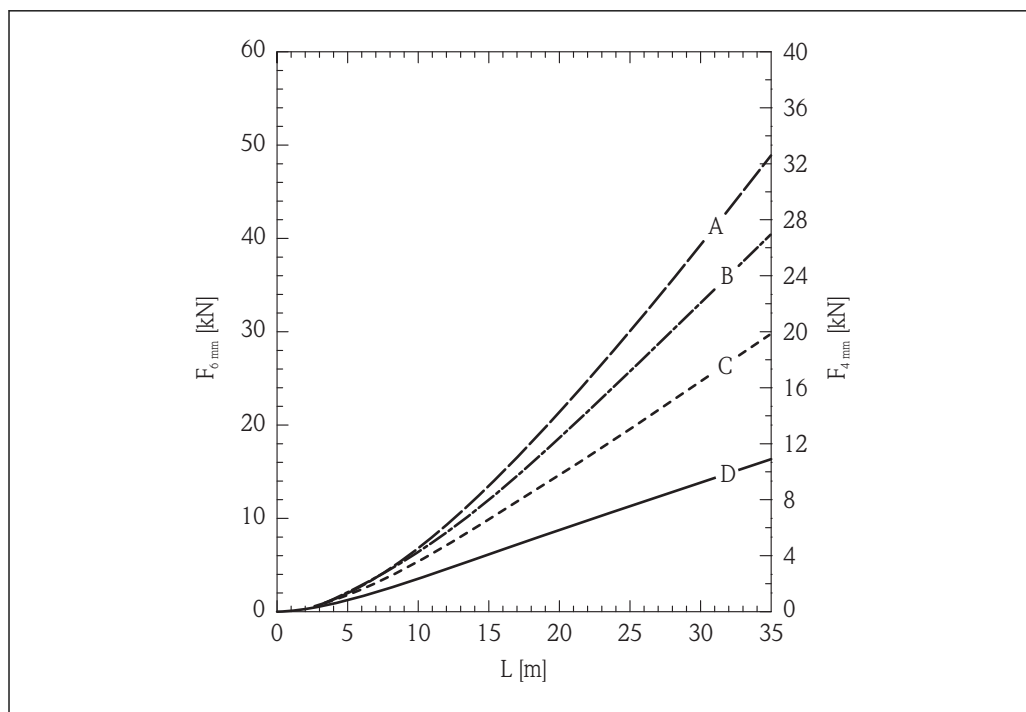
8 Ciment dans un silo métallique avec parois lisses ; charge de traction en fonction du niveau L pour des diamètres de câble de 6 mm (0,24 in) et 4 mm (0,16 in)
