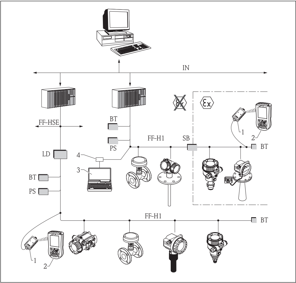
18 Architecture du système FOUNDATION Fieldbus avec composants associés
