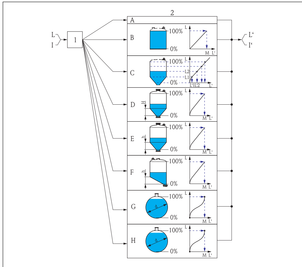
39 Linéarisation : conversion du niveau et, le cas échéant, de l'interface en un volume ou une masse ; la conversion dépend de la forme de la cuve
