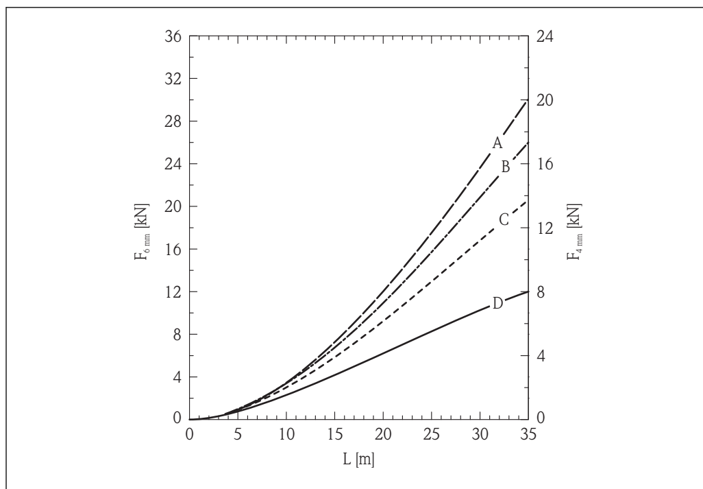
7 Blé dans un silo métallique avec parois lisses ; charge de traction en fonction du niveau L pour des diamètres de câble de 6 mm (0,24 in) et 4 mm (0,16 in)
