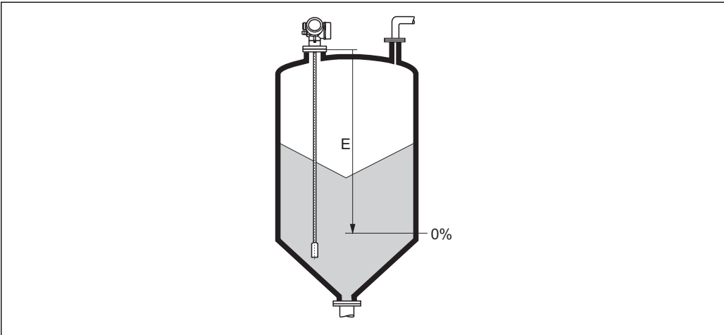
34 Distance du point zéro (E) pour la mesure sur solides
