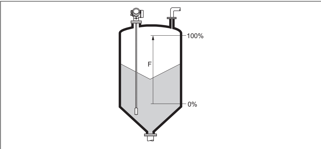
35 Plage de mesure (F) pour la mesure sur solides
