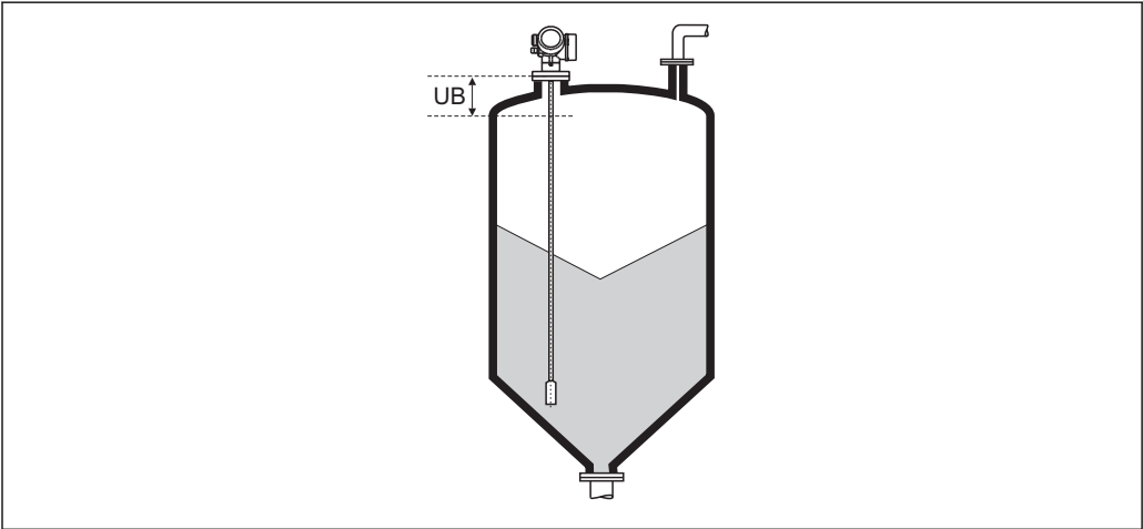
38 Distance de blocage (UB) pour la mesure dans les solides
