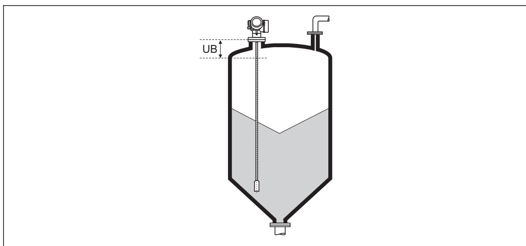
41 Distance de blocage (UB) pour la mesure dans les solides
