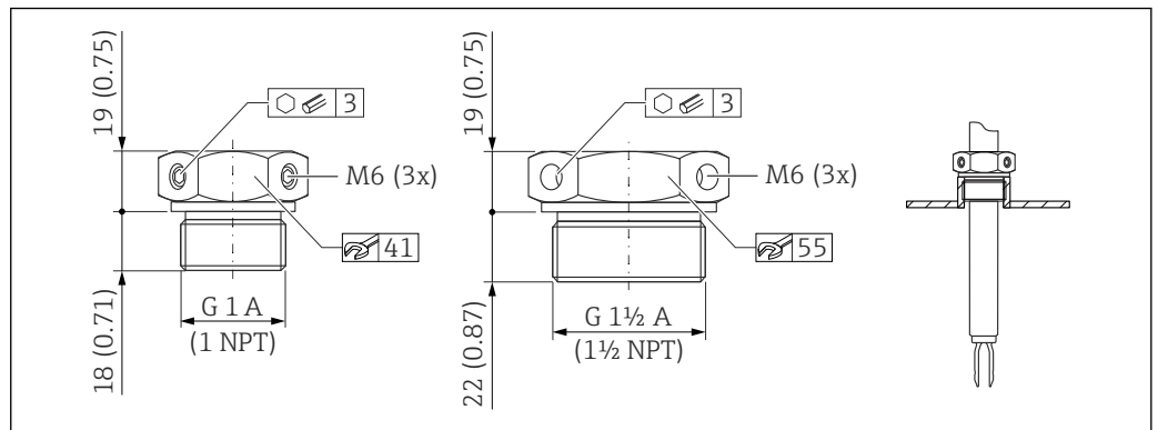
49 常压滑动套管 p_e = 0 \text{ bar (0 psi)} 。测量单位 mm (in)
