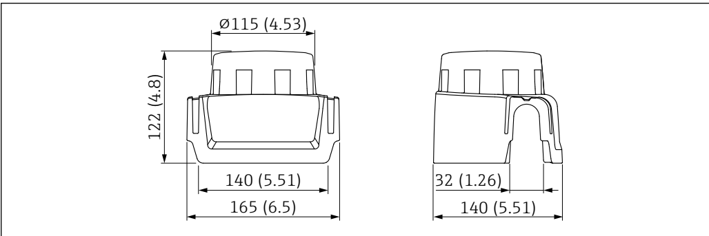
46 塑料防护罩 XW111 的外形尺寸示意图。测量单位 mm (in)
