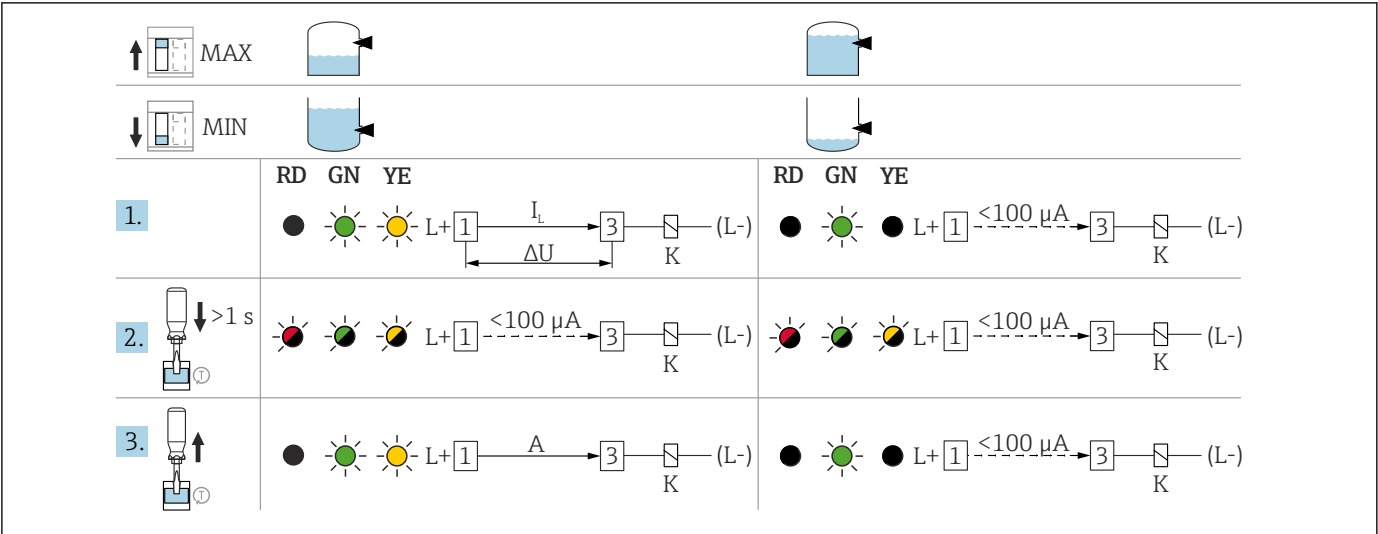
37 FEL62 的继电器响应和故障报警信号
