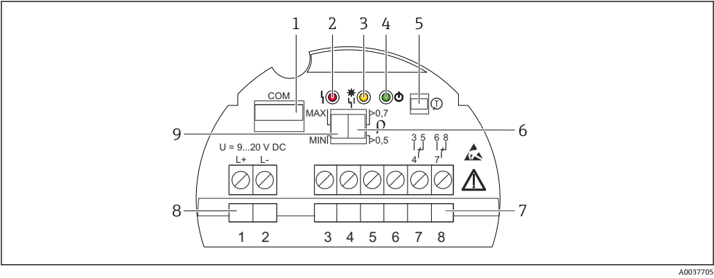
图 33 实例：电子插件 FEL64DC 1 通信接口，用于连接附加模块（LED 指示灯、Bluetooth®蓝牙模块） 2 红色 LED 指示灯：警告或报警 3 黄色 LED 指示灯：音叉开关状态 4 绿色 LED 指示灯：设备工作状态（设备开启） 5 测试按钮，用于执行功能测试 6 DIP 开关，密度设定值为 0.7 或 0.5 7 继电器触点接线端子（3...8） 8 电源接线端子（1...2） 9 DIP 开关，高限（MAX）/低限（MIN）检测设置
