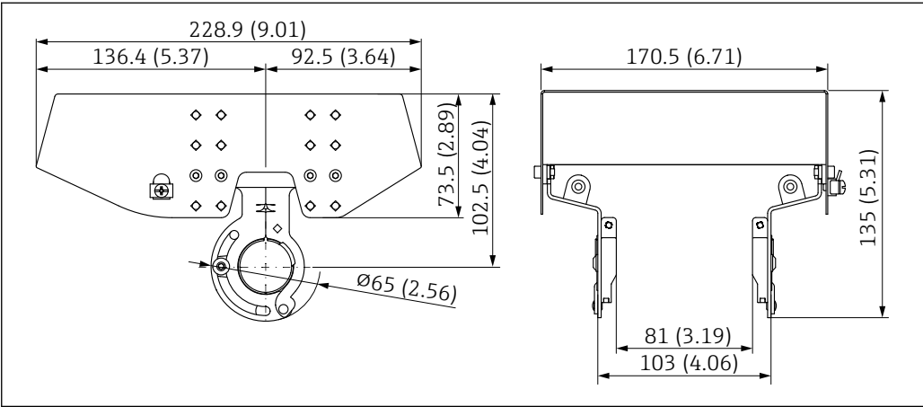
45 316L 防护罩 XW112 的外形尺寸示意图。测量单位 mm (in)
