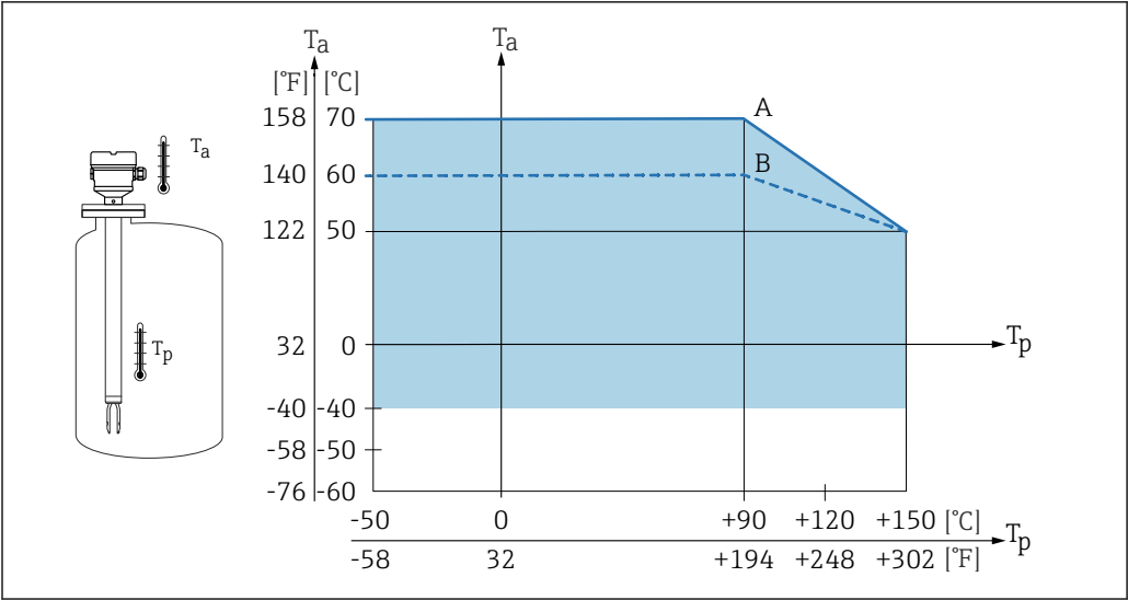
图 52 外壳允许环境温度 T_a 与容器内部过程温度 T_p 的关系：
