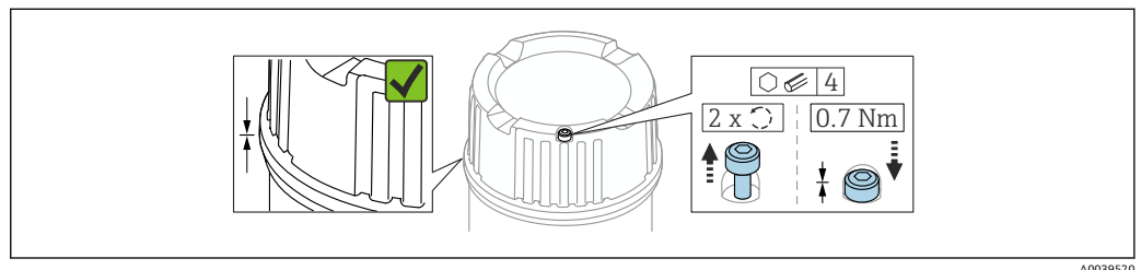
图 16 带锁定螺丝的外壳盖
