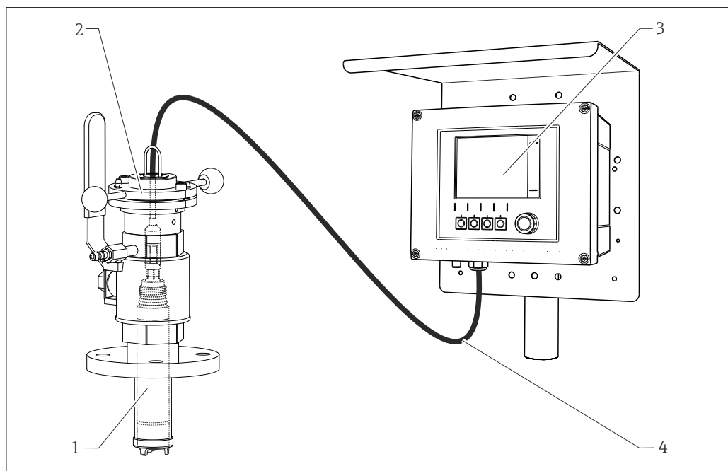
6 Пример измерительной системы с датчиком кислорода Memosens COS51E цифровым датчиком кислорода
