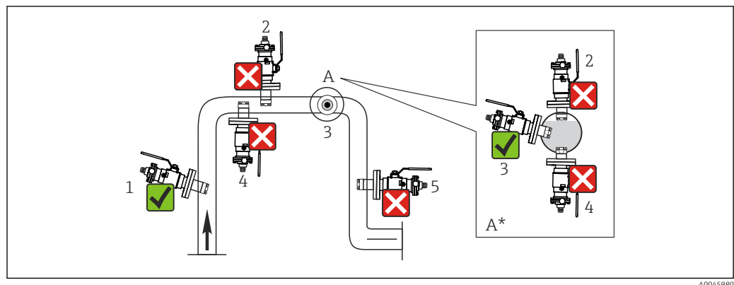
7 Допустимые и недопустимые положения монтажа датчика с выдвижной арматурой
