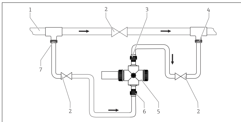
16 Схема подключения
