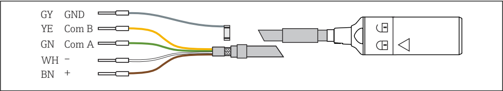
18 Измерительный кабель СУК10
