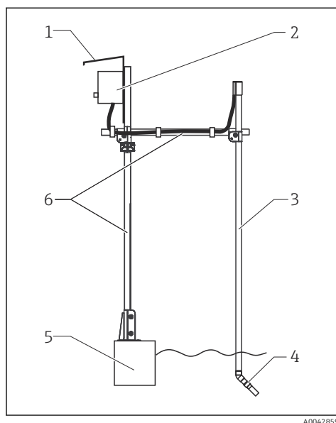
10 Блок держателя с погружной трубой
