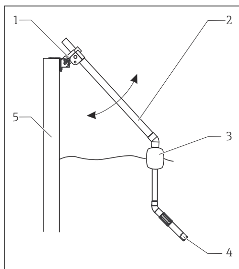
11 Установка на борт резервуара
