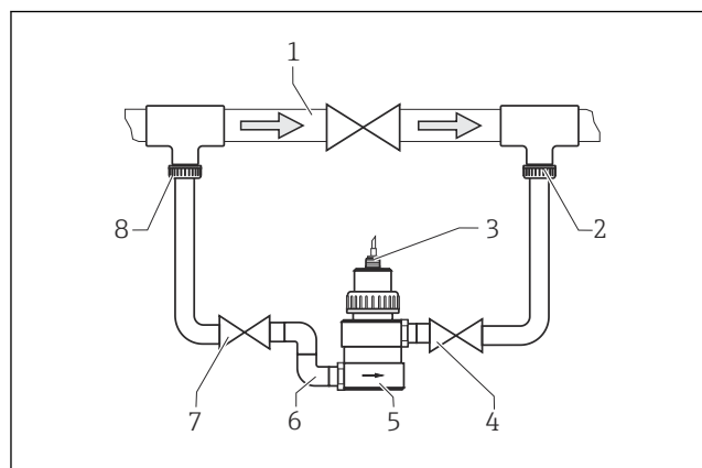
14 Монтаж на байпасной трубе с клапанами с ручным управлением или электромагнитными клапанами
