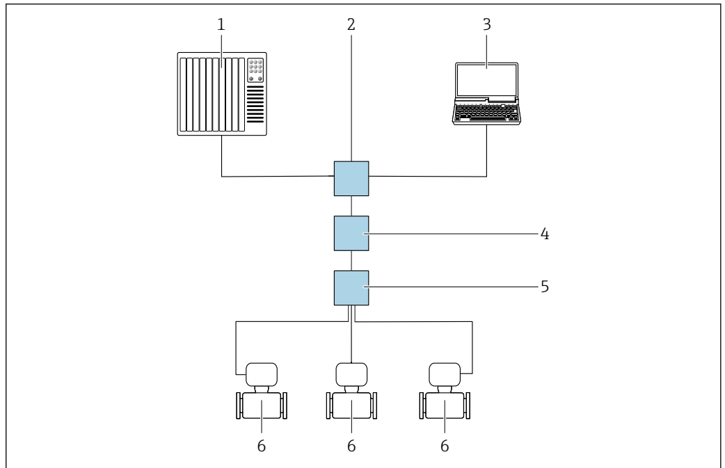
41 Opções para operação remota através do protocolo Modbus TCP por Ethernet-APL (ativa)
