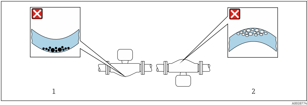
14 Direção do sensor com tubo de medição curvado
