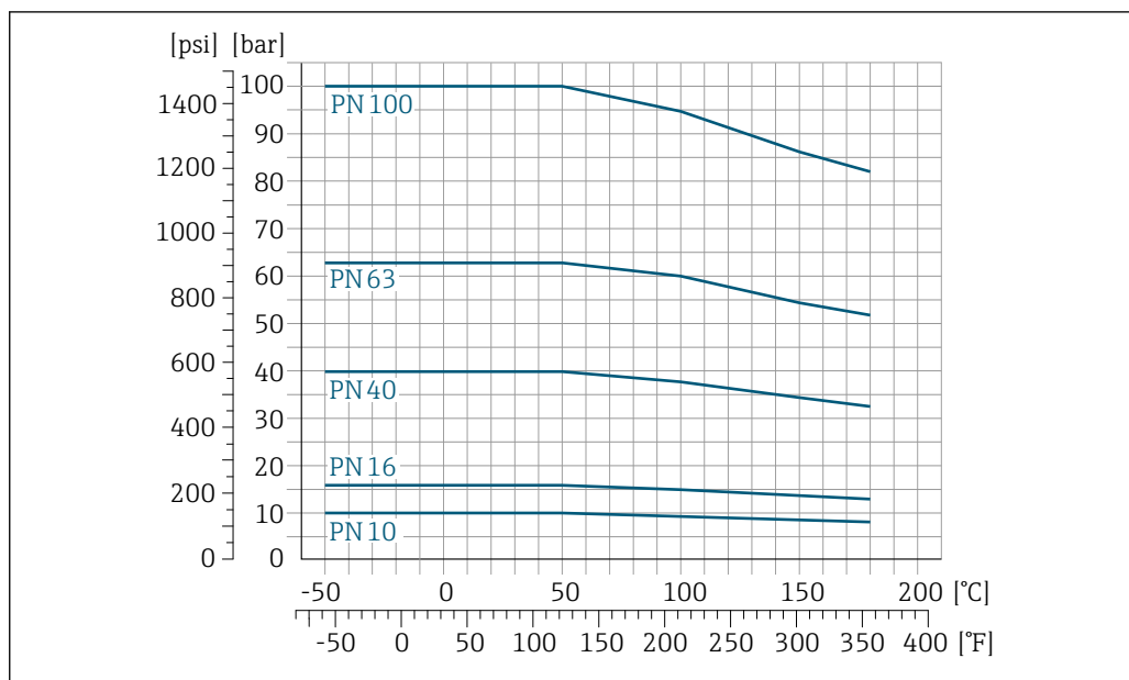
17 Com material de flange 1.4404 (316/316L)
