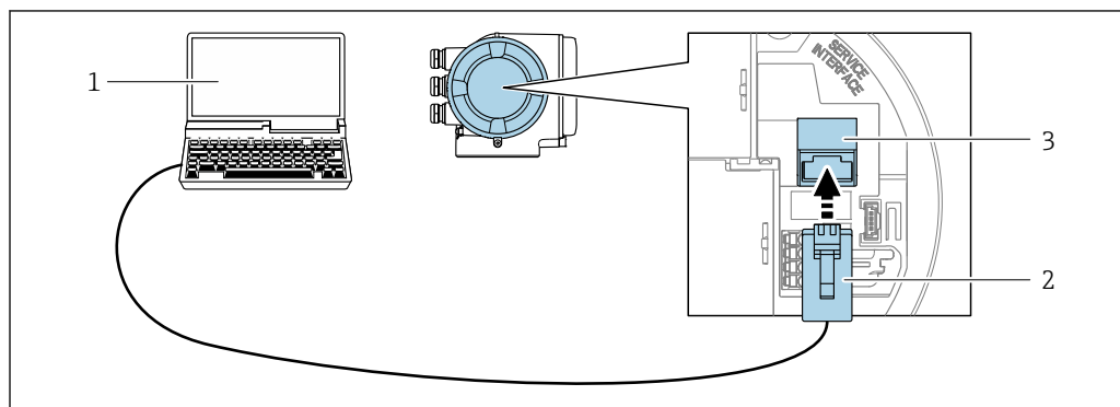
47 Conexão através de Interface de operação (CDI-RJ45)
