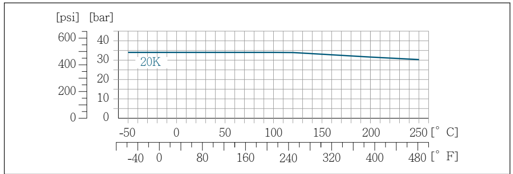
23 Com material do flange 1.4301 (F304), partes úmidas Liga C22
