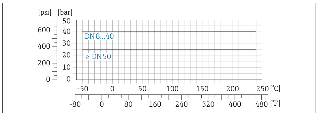
25 Com material da conexão: 1.4404 (316/316L)
