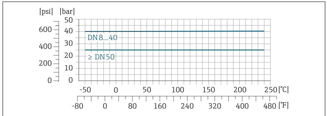
24 Com material da conexão: 1.4404 (316/316L)
