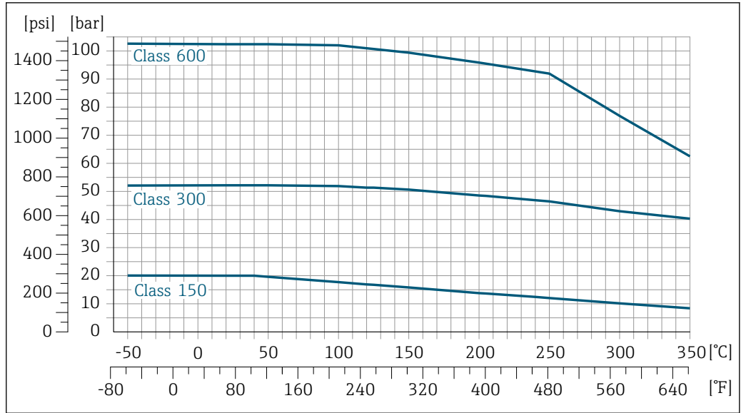
18 Com material do flange Liga C22
