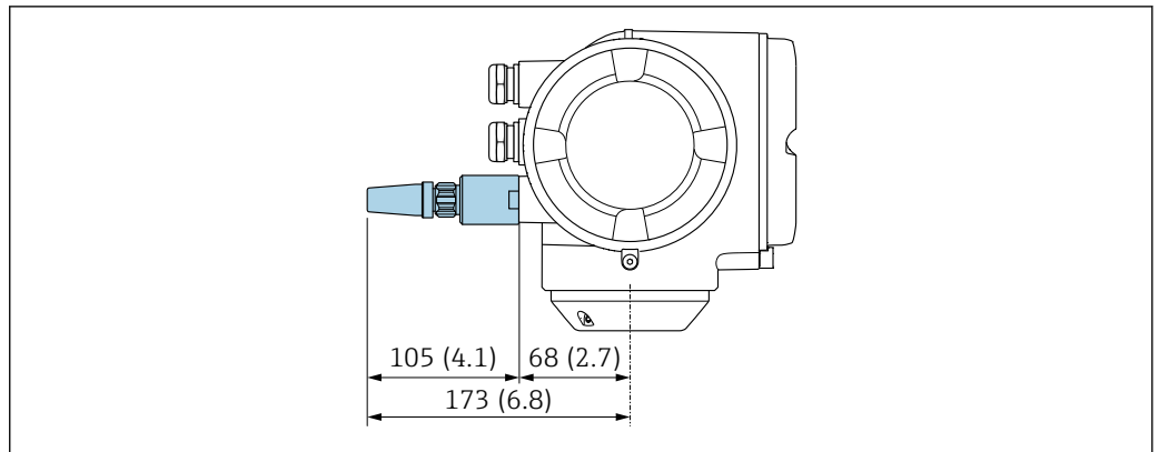
38 Unidade em mm (pol.)
