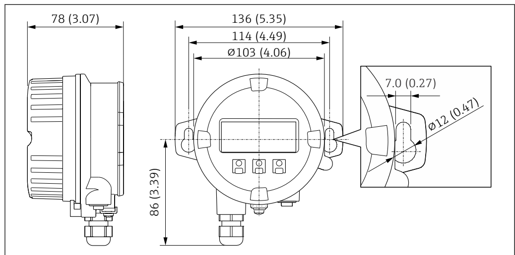
33 Unidade em mm (pol.)
