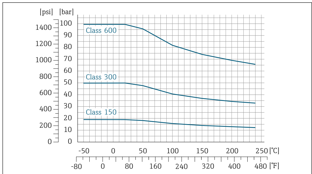
22 Com material do flange 1.4301 (F304), partes úmidas Liga C22
