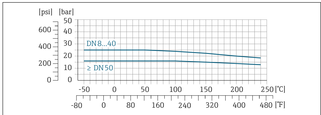
20 Com material da conexão: 1.4404 (316/316L)
