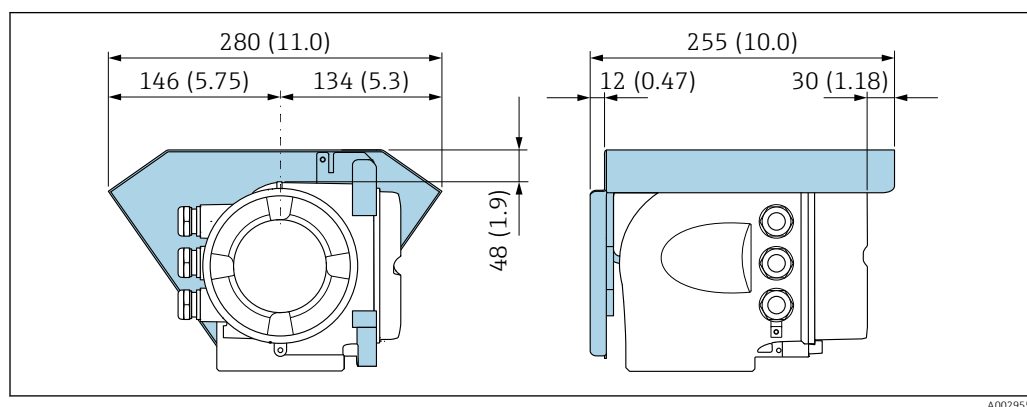
36 Unidade em mm (pol.)
