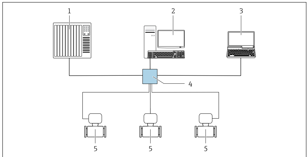
50 Opções para operação remota através do Modbus TCP por Ethernet - 100 Mbit/s: Topologia estrela
