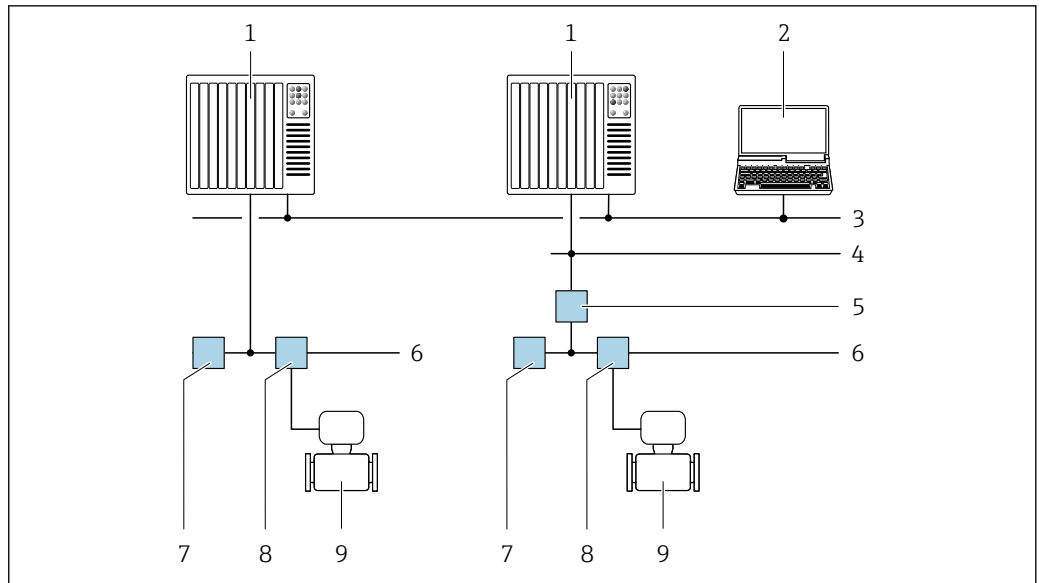
45 Opções para operação remota através da rede FOUNDATION Fieldbus
