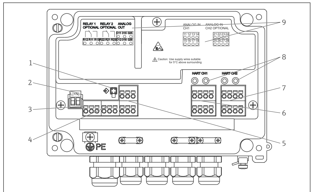
图 4 设备的接线端子分配（通道 2 和继电器，可选）
