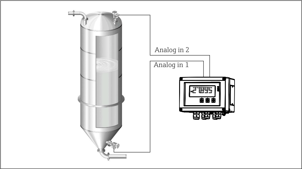
图 8 差压应用
