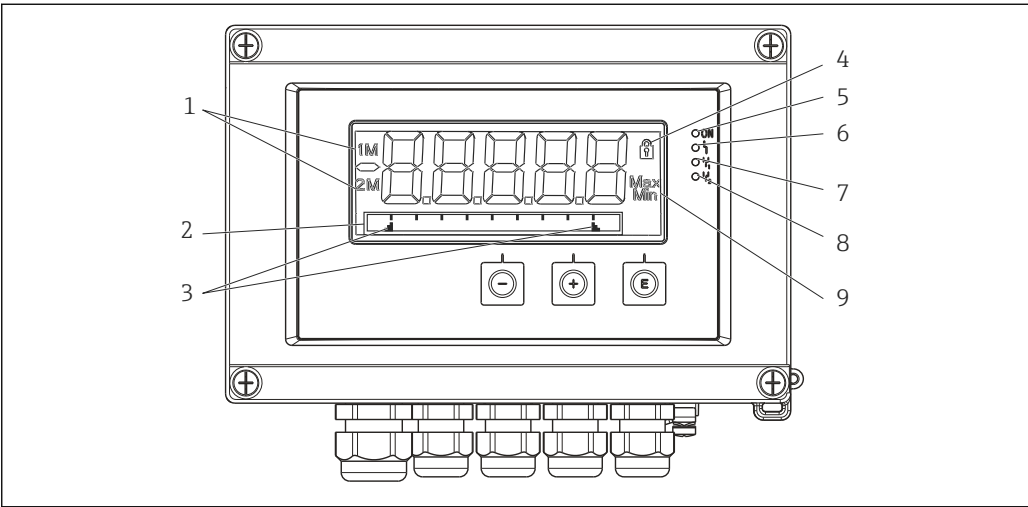
图 19 过程显示单元的显示屏
