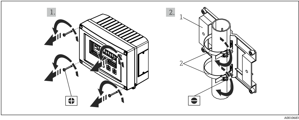
图 2 在管道上安装现场型测控仪
