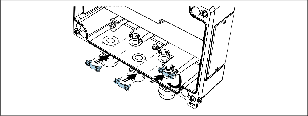
图 6 屏蔽层接地连接
