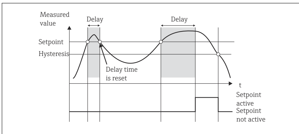
图 14 回差和延迟时间启用
