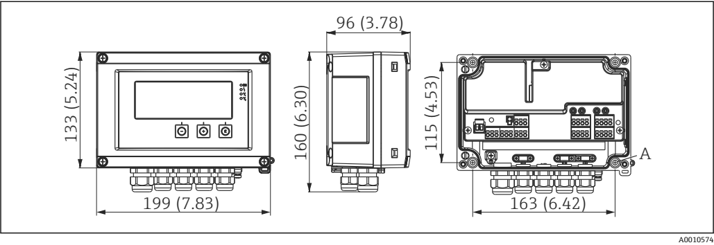
图 18 过程显示单元的外形尺寸示意图；单位：mm (in) A 通过钻孔直接安装在墙壁上，或通过 4 个螺丝 (ø5 mm (2 in)) 安装在选配安装板上
