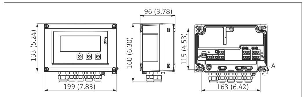
图 1 现场型测控仪的外形尺寸示意图；单位：mm (in)
