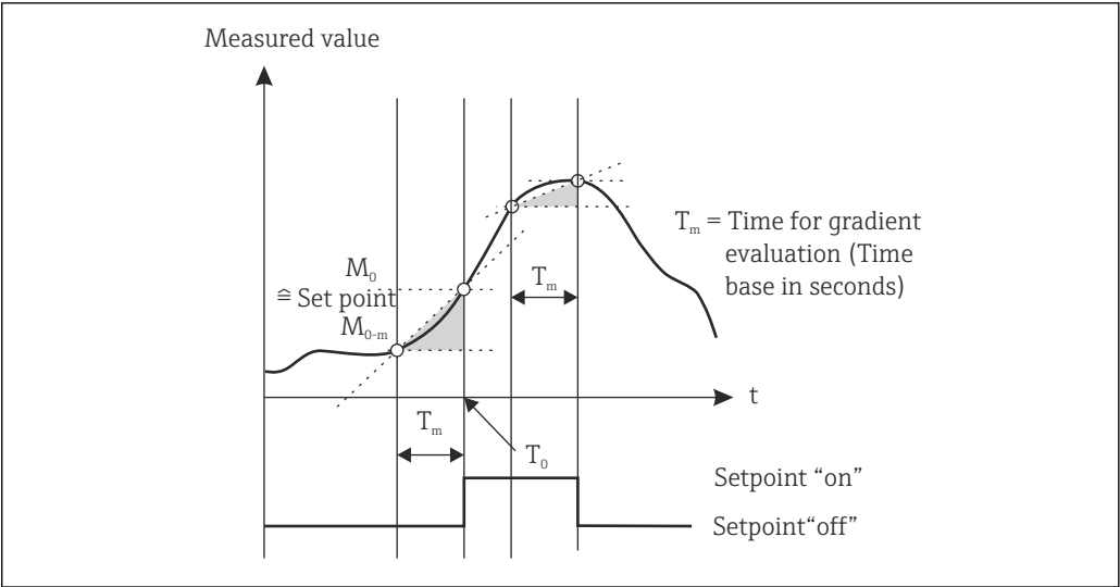
图 11 Gradient 工作模式
