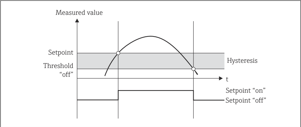
图 10 Max 工作模式
