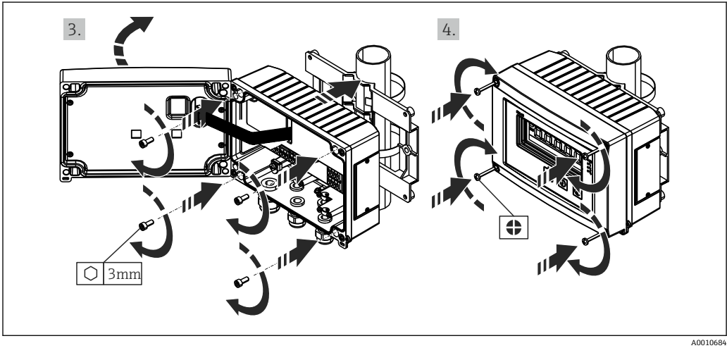
图 3 在管道上安装现场型测控仪
