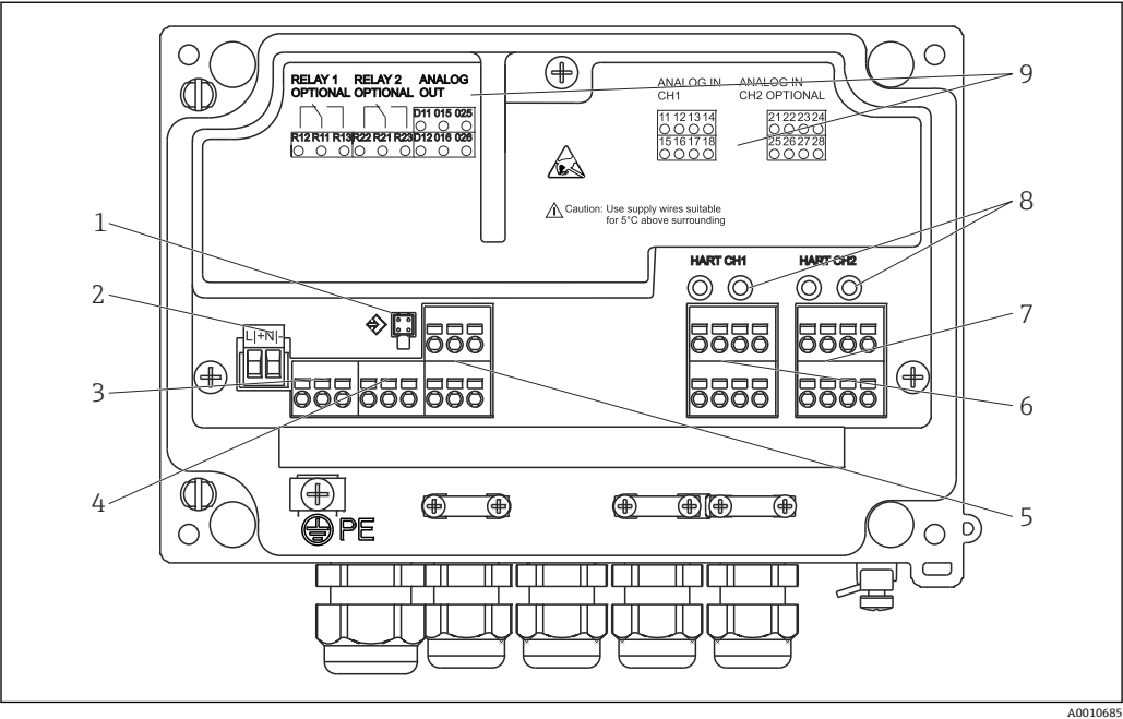
图 17 过程显示单元的内部视图和接线端子分配
