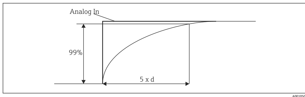
图 15 信号阻尼
