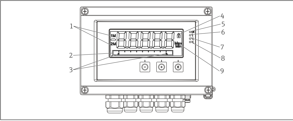
图 7 现场型测控仪的显示屏
