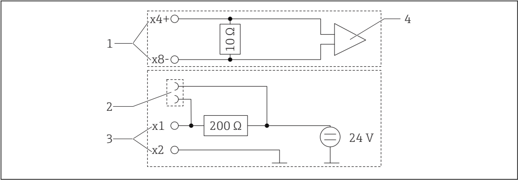
图 5 HART®连接插座的内部电路
