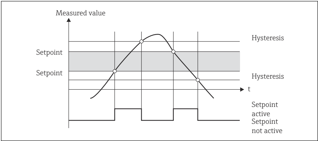
图 12 OutBand 工作模式
