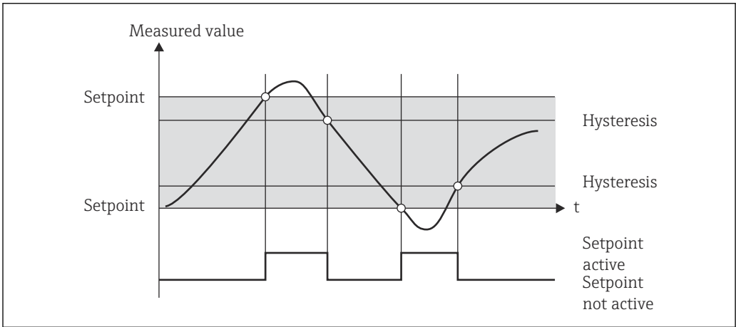
图 13 InBand 工作模式
