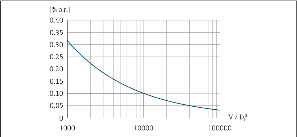
图 30 重复性 = 0.1 % o.r., 体积流量测量值[m³] of V = 10 000 · D i 3
