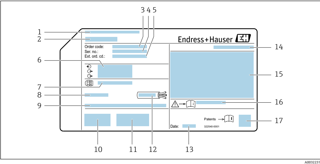
图 2 变送器的铭牌示意图 1 制造商地址/取证地 2 变送器名称 3 订货号 4 序列号 5 扩展订货号 6 电气连接参数（例如可选输入和输出、供电电压） 7 缆塞类型 8 允许环境温度 ( T_a ) 9 出厂固件版本号和设备修订版本号 10 CE 认证、RCM-Tick 认证 11 附加信息（与实际型号相关）：证书、认证 12 电缆允许温度范围 13 生产日期：年-月 14 防护等级 15 防爆认证信息 16 《安全指南》文档资料代号 17 二维码
