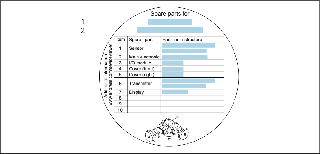
图 29 接线腔盖中的“备件标签”示例
