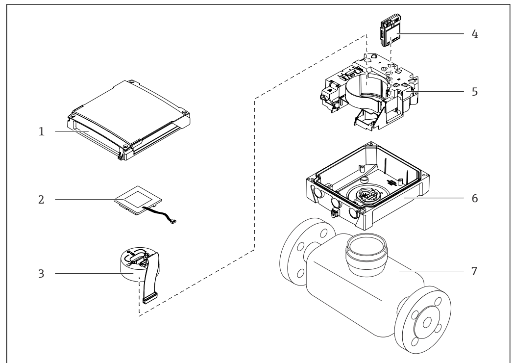
図 2 一体型の主要コンポーネント
