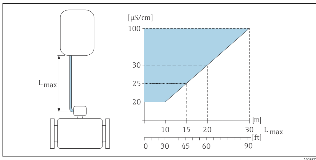
図 3 許容される接続ケーブル長
