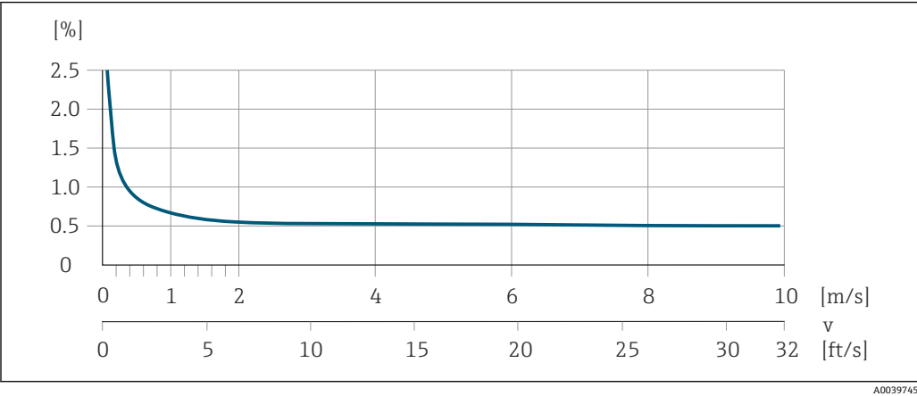
図 17 最大測定誤差 (%) o.r.
