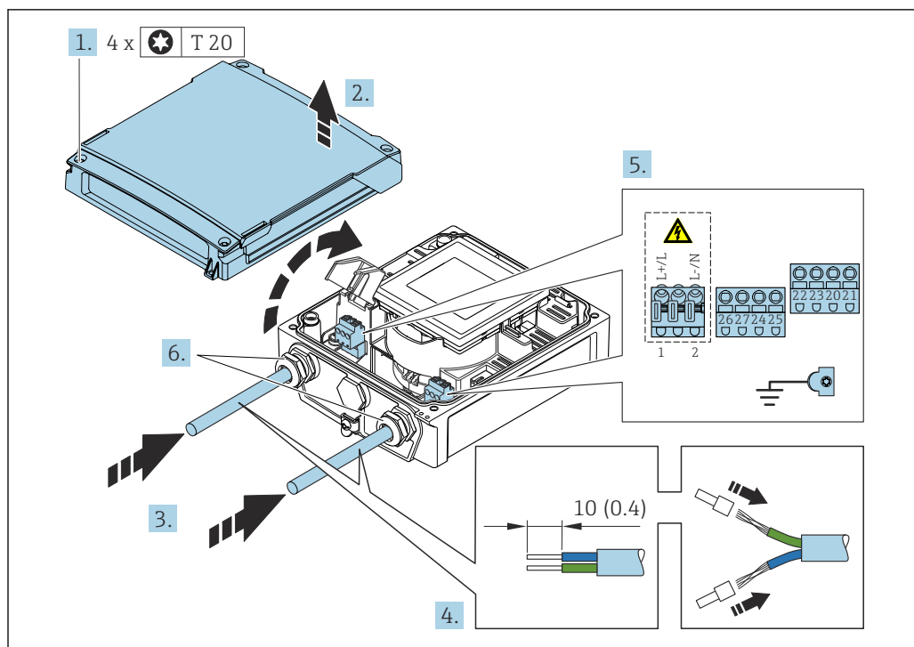
図 14 電源の接続
