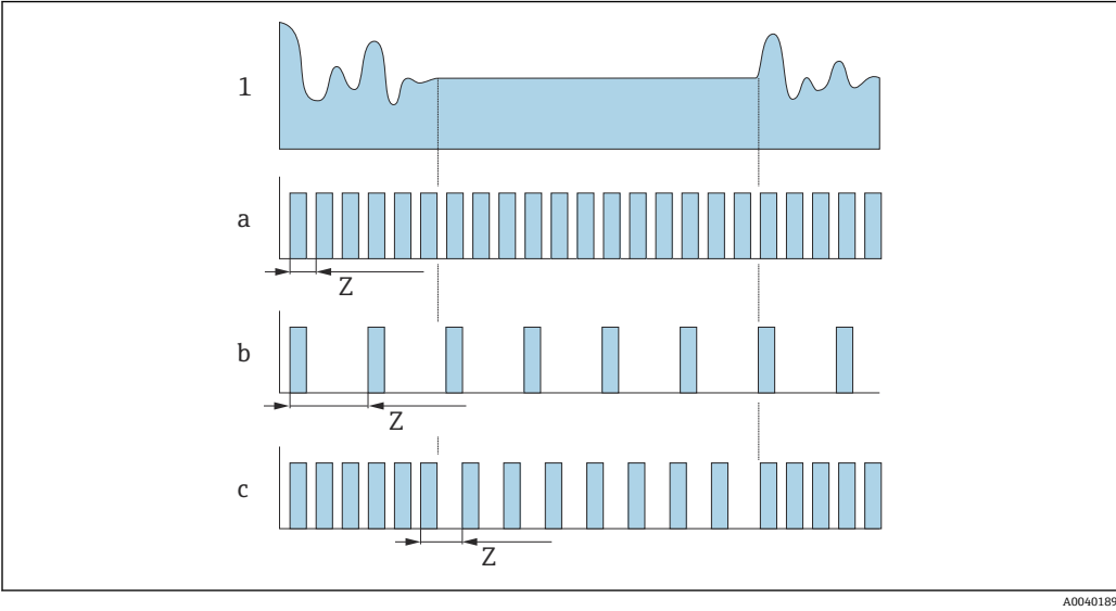
図 16 各種のデータのログ方法の動作原理
