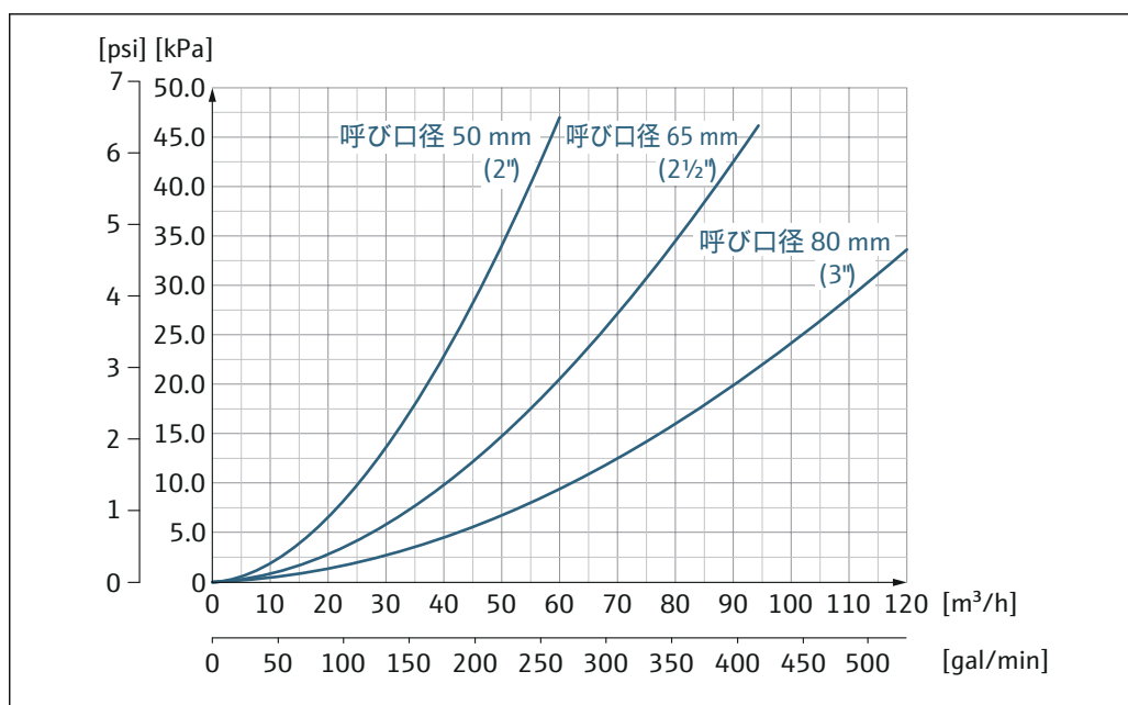
図 18 呼び口径 50～80 mm (2～3") の圧力損失：「設計」のオーダーコード、オプション C「固定フランジ、縮小計測チューブ、0 x 呼び口径 上流側/下流側直管長」の場合
