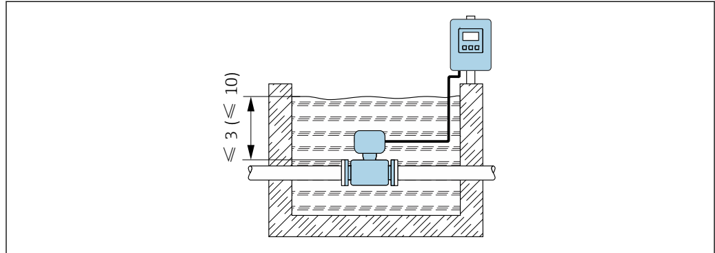
図 5 水中に常時浸漬する場合の設置
