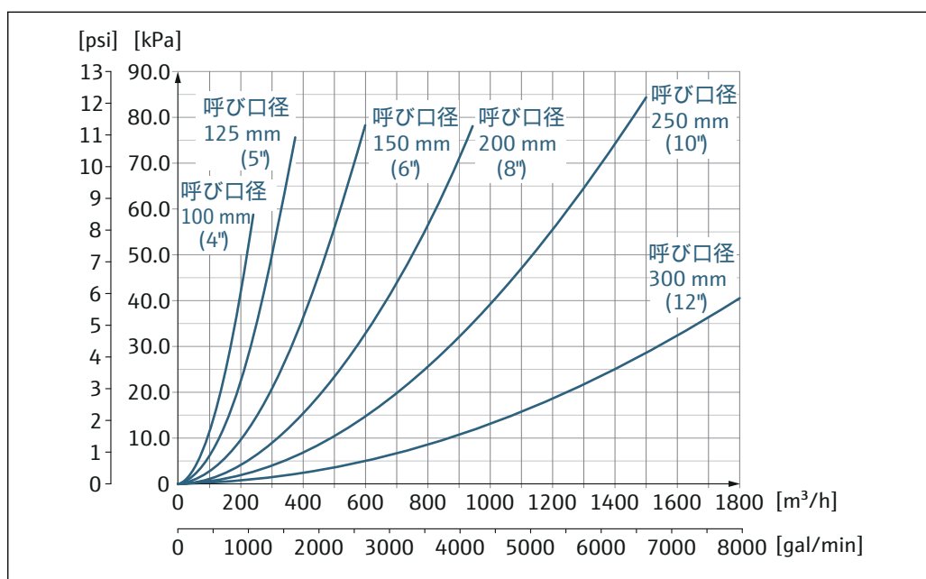
図 19 呼び口径 100～300 mm (4～12") の圧力損失：「設計」のオーダーコード、オプション C「固定フランジ、縮小計測チューブ、0 x 呼び口径 上流側/下流側直管長」の場合
