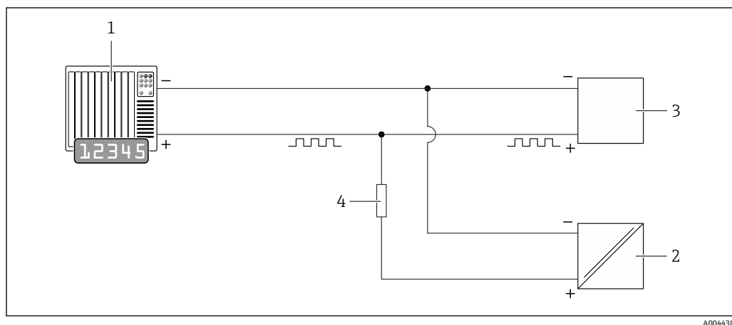
図 15 パルス出力（パッシブ）の接続例
