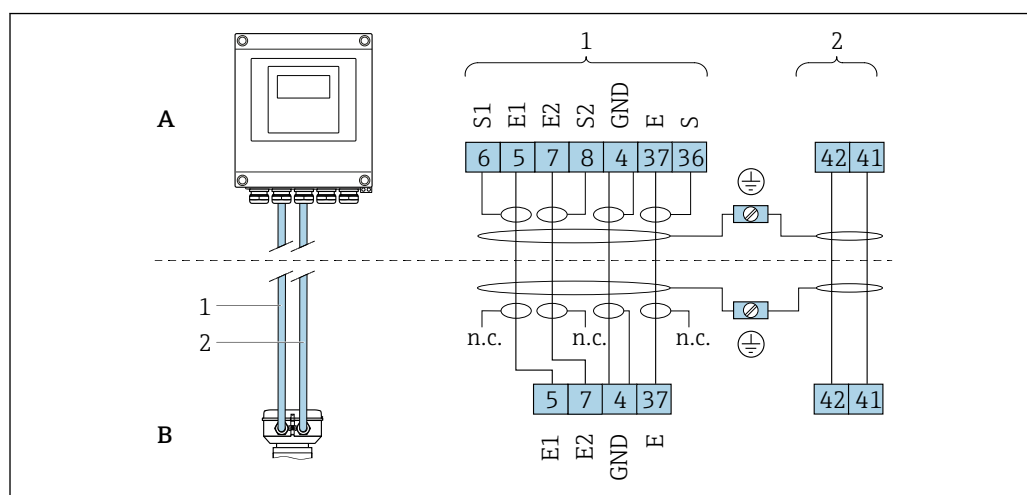
図 9 分離型の端子の割当て
