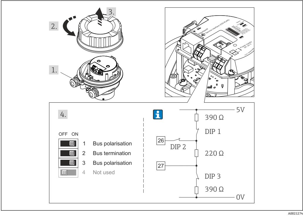
12 使用 I/O 电子模块上的 DIP 开关端接(波特率小于 1.5 MBaud)
