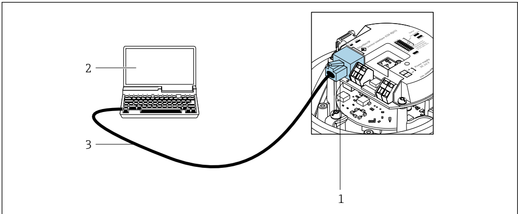
图 19 订购选项“输出”，选型代号 L: PROFIBUS DP
