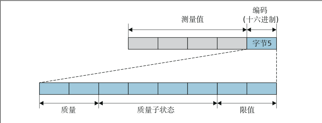
图 16 编码字节结构
