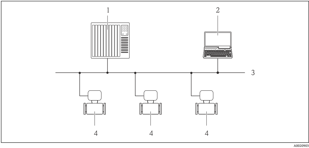
图 14 通过 PROFIBUS DP 网络进行远程操作
