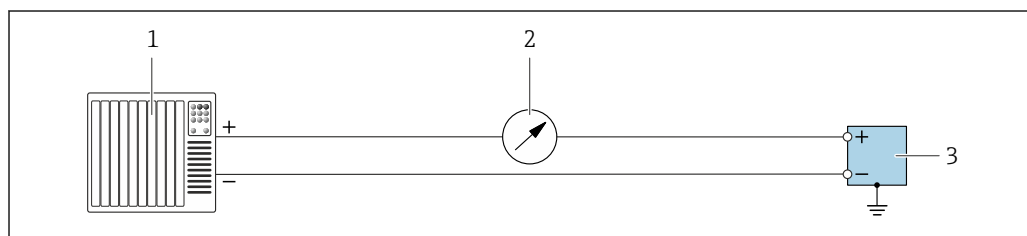
18 Exemplo de conexão para saída em corrente 4 para 20 mA (ativa)
