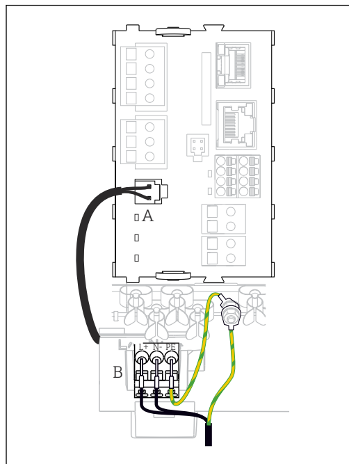
21 BASE2-E 电源接线示意图
