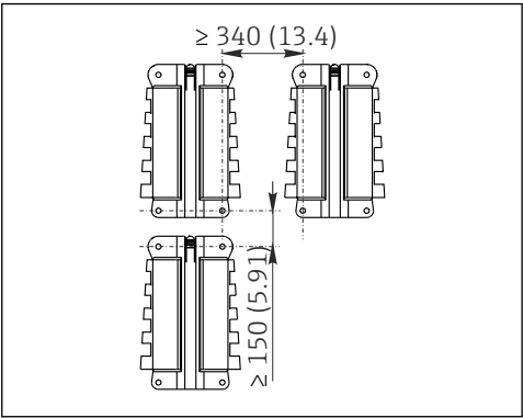
34 安装间距; 单位: mm (in)
