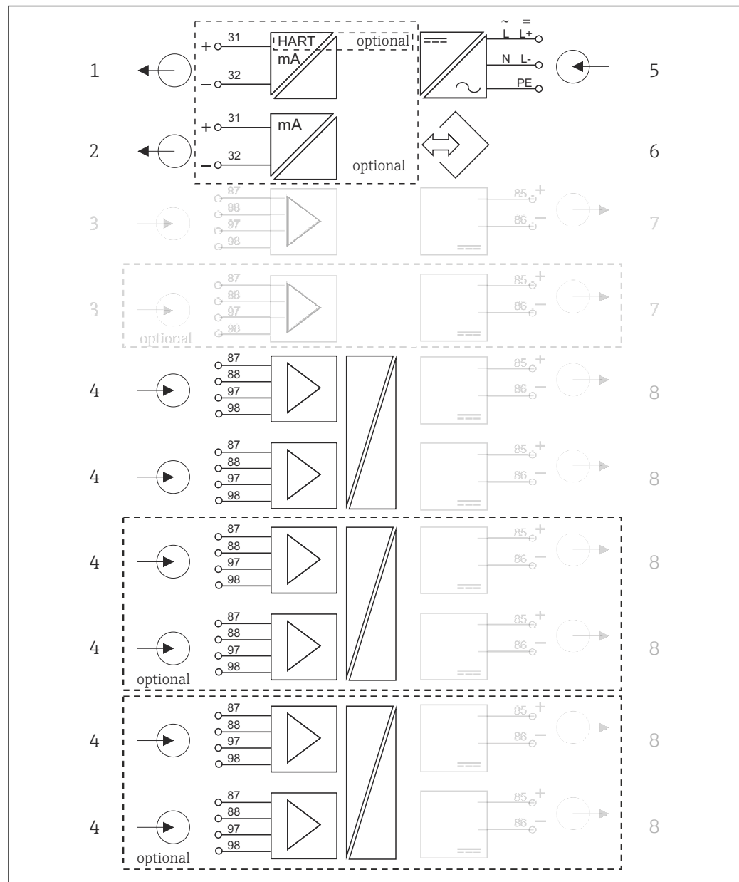
图 11 CM448 (安装有本安传感器通信模块 2DS Ex-i) 的电路框图
