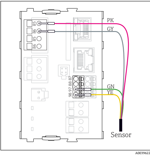
25 传感器，连接附加电源
