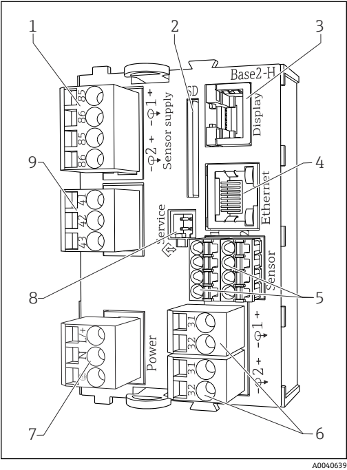
17 基本模块 BASE2-H 或 -L（双通道型设备）
