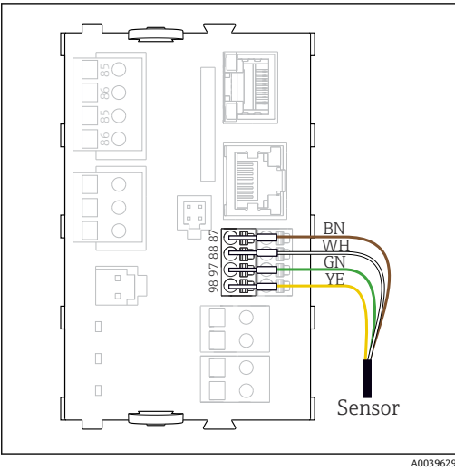
24 传感器，不连接附加电源
