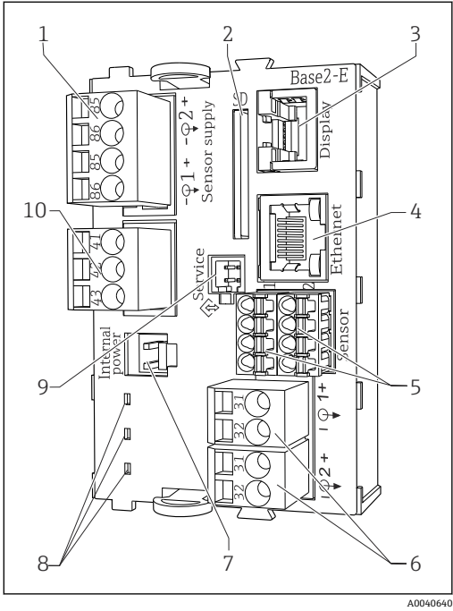
18 基本模块 BASE2-E（四通道型和八通道型设备）
