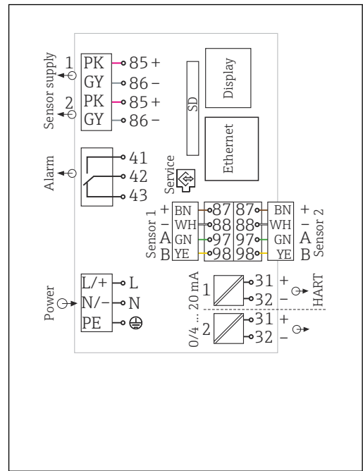
20 BASE2-H 或 BASE2-L 模块的完整接线图
