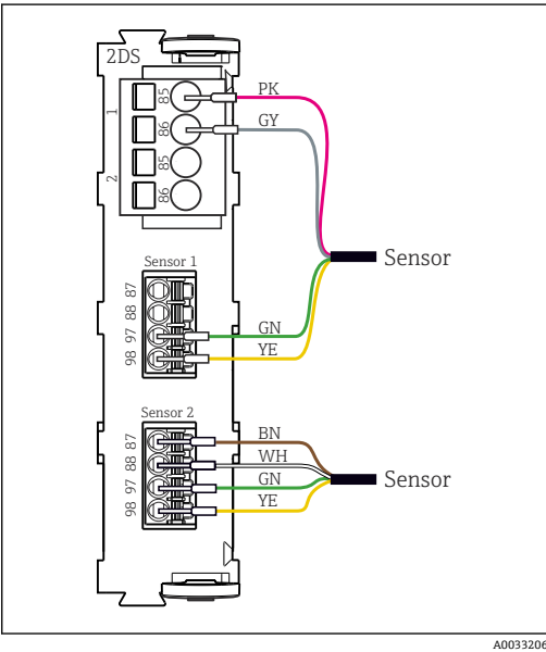
26 传感器，连接/不连接传感器模块 2DS 处的附加电源
