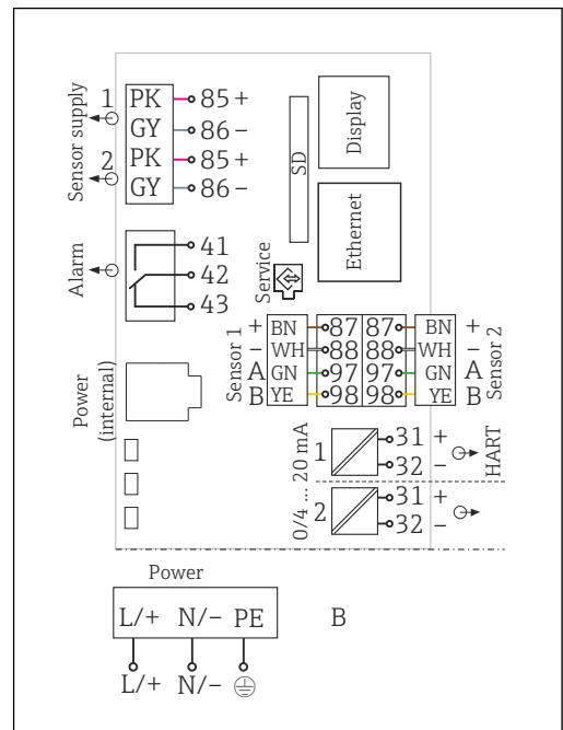
22 BASE2-E 模块和扩展供电单元 (B) 的完整接线图
