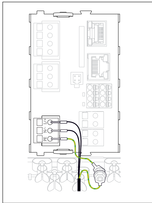
19 BASE2-H 或 BASE2-L 模块的电源接线示意图
