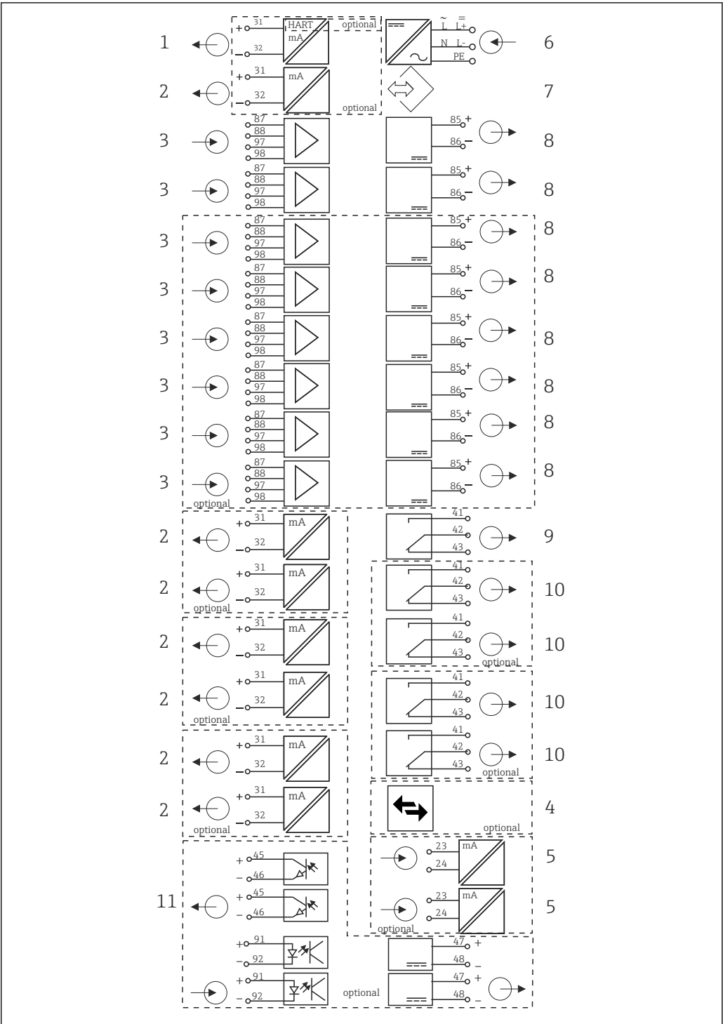
10 CM448 的电路框图
