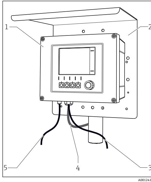
图 1 测量系统 (例如双通道型设备)
