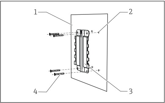
35 墙装示意图
