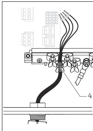
20 Připojte kabel k uzemňovací sponě
