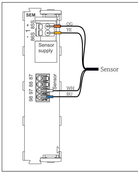
31 Připojení spektrometru k modulu SEM
