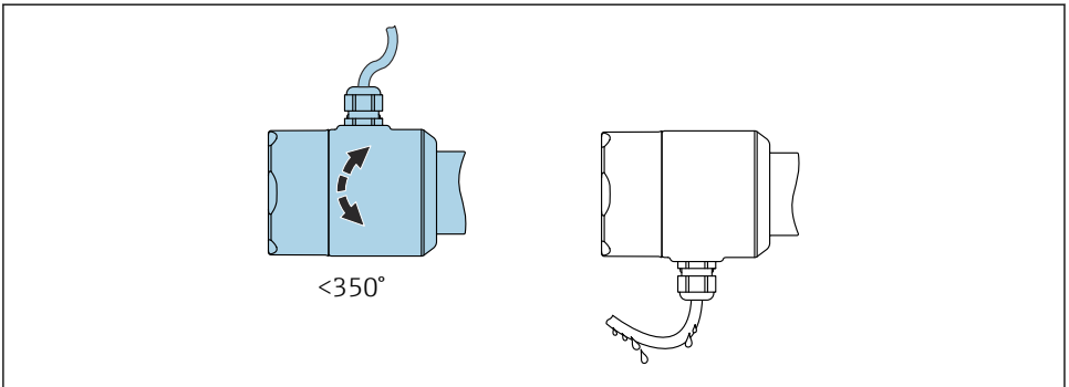
☞ 12 고정 나사가 없는 하우징: 케이블에 배수 루프를 만드십시오.
