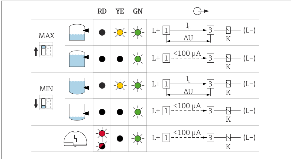
▣ 16 FEL42 스위칭 동작, LED 신호
