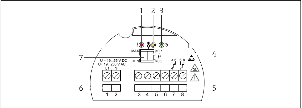
☐ 22 기판 FEL44 예
