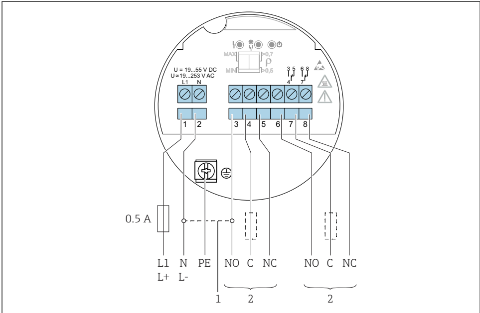
☞ 17 릴레이 출력이 있는 범용 전류 연결(기판 FEL44)
