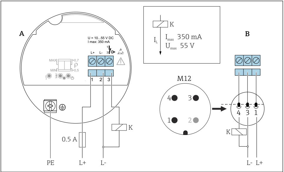
15 단자 할당 FEL42
