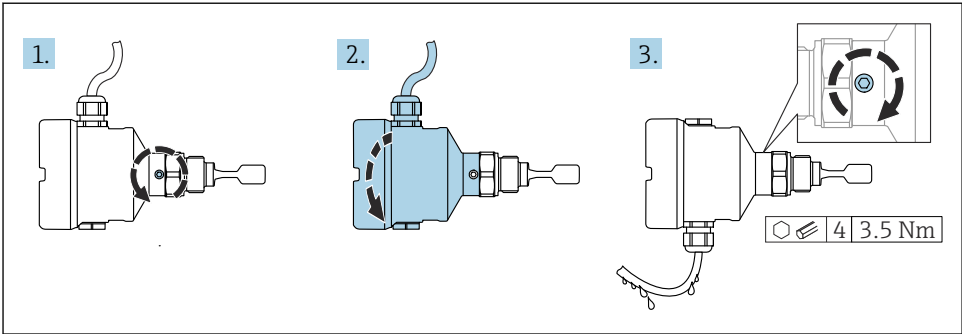
☞ 13 외부 잠금 나사가 있는 하우징: 케이블에 배수 루프를 만드십시오.
