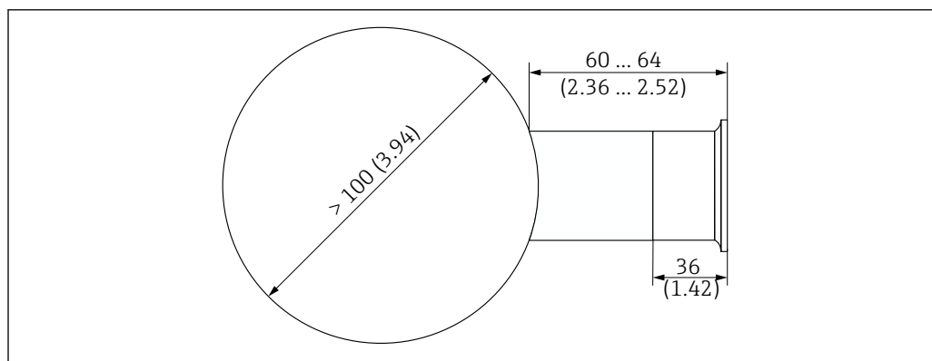
19 Conexão de tubo com adaptador soldado. Unidade: mm (pol.)
