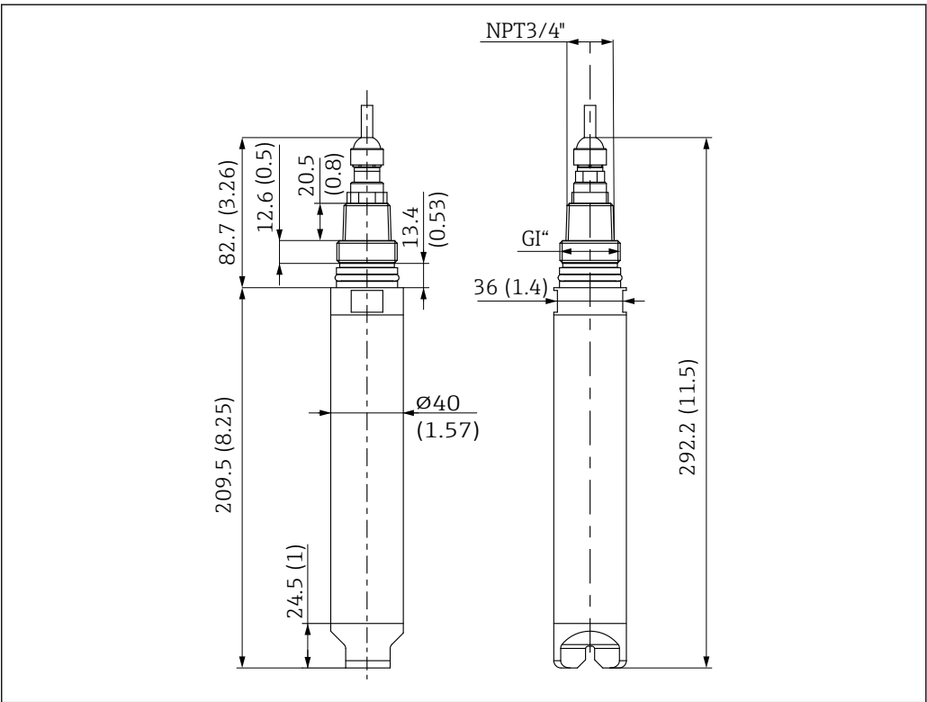
15 Dimensões . Dimensões: mm (pol.)
