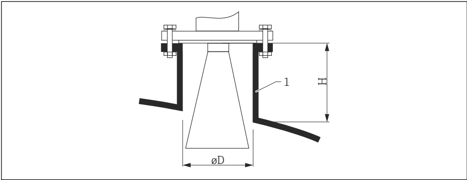
6 A csővég magassága és átmérője a tölcserantennához (FMR54)
