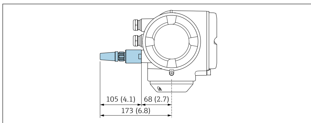
31 Ед. изм.: мм (дюймы)
