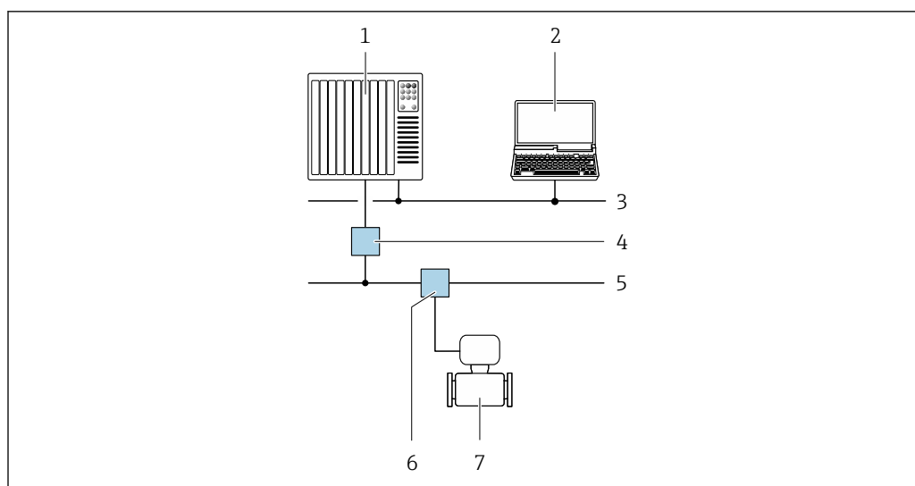
45 Варианты дистанционного управления по сети PROFIBUS PA
