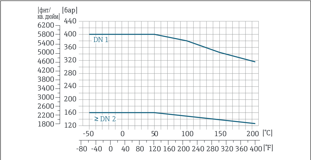
25 Соединение 4-VCO-4: 1.4539 (904L); соединение 8-VCO-4: 1.4539 (904L); резьбовой переходник NPTF: 1.4539 (904L)
