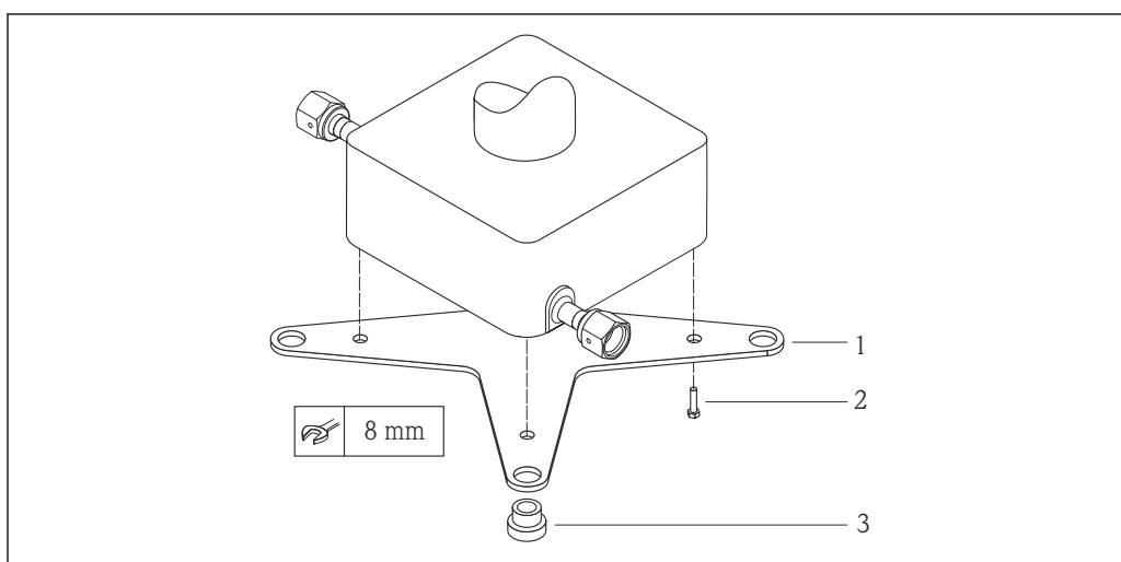
18 Монтажный комплект для монтажной пластины Cubemass
