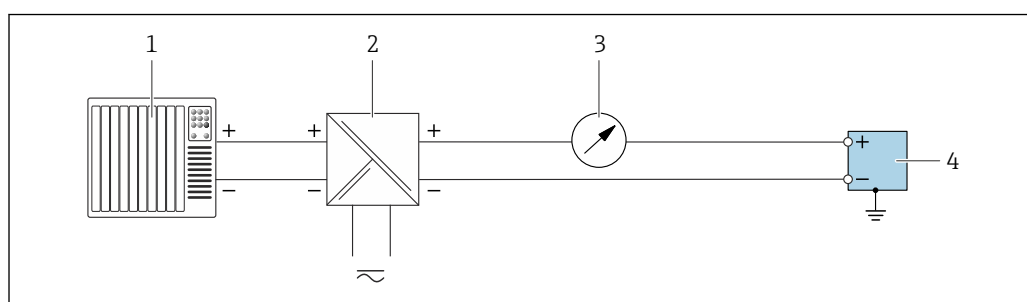
3 Пример подключения для токового выхода 4 до 20 мА (пассивного)
