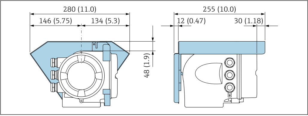
20 Защитный козырек от погодных явлений для Proline 500 – единица измерения- мм (дюймах)
