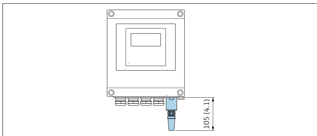
35 Ед. изм.: мм (дюймы)
