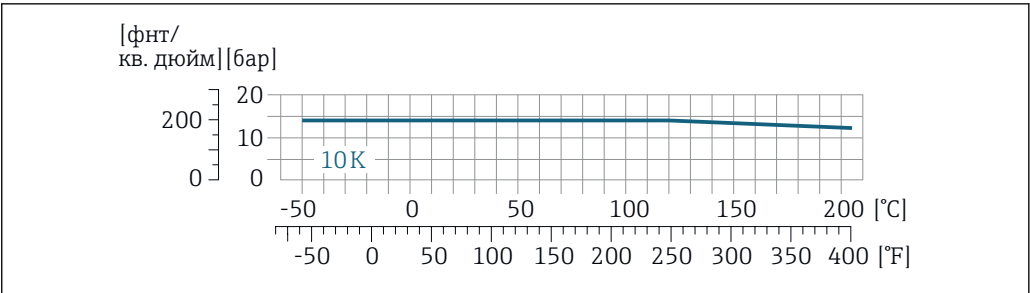
24 С фланцем 1.4539 (904L); свободные (не смачиваемые) фланцы 1.4404 (316/316L)
