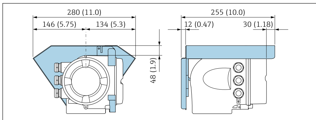
34 Защитный козырек от погодных явлений для Proline 500 – единица измерения- мм (дюймах)
