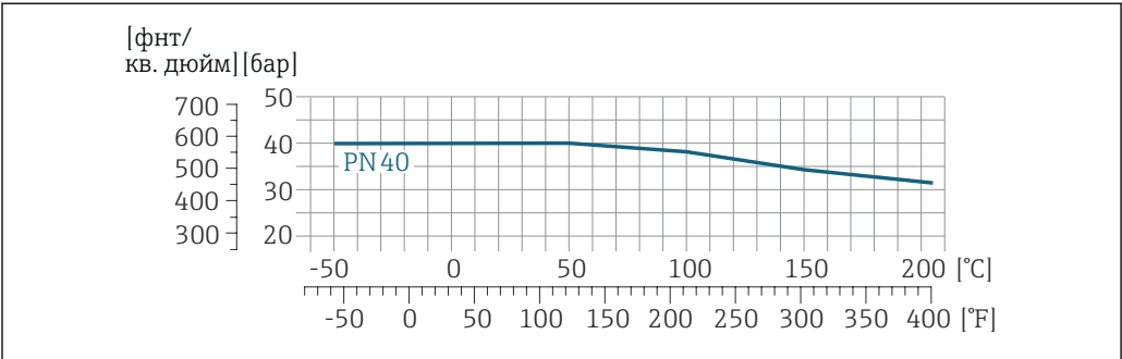
22 С фланцем 1.4539 (904L), сплав Alloy C22; со свободным кольцом (не смачиваемые) фланцы 1.4404 (316/316L)
