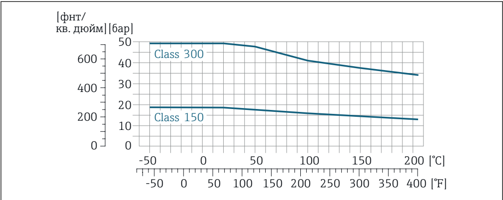
23 С фланцем 1.4539 (904L); свободные (не смачиваемые) фланцы 1.4404 (316/316L)
