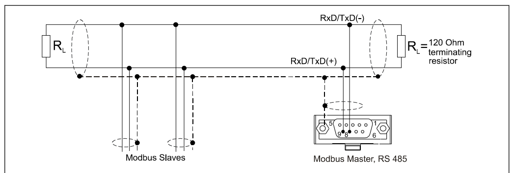
Asignación de pines del conector Modbus RTU
