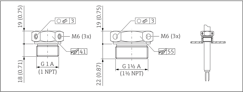
25 常压滑动套管 p_e = 0 bar (0 psi)。测量单位 mm (in)
