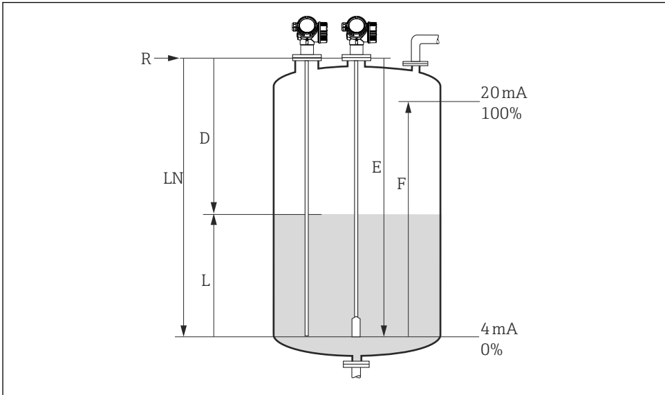
15 Parametri di configurazione per le misure di livello nei liquidi
