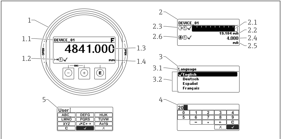
13 Raffigurazione del display operativo e di visualizzazione per il funzionamento on-site
